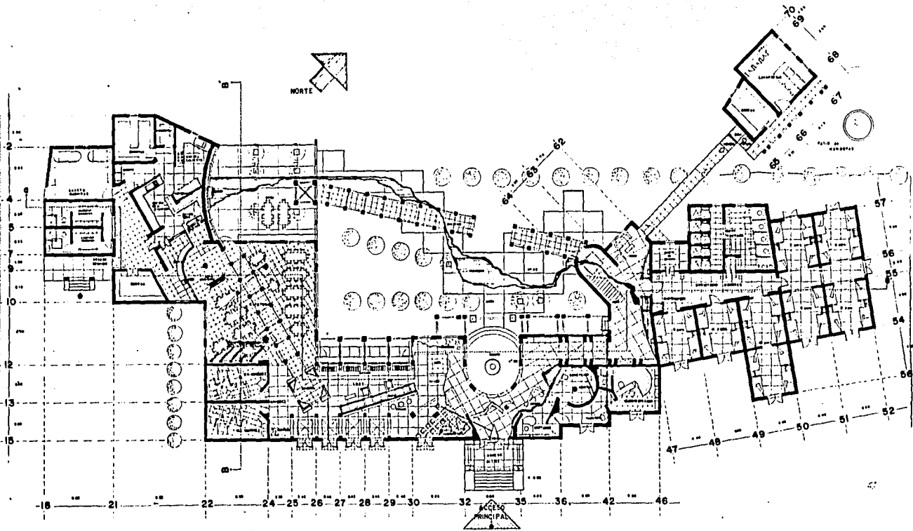
planta baja
