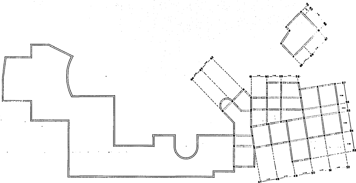
estructura planta alta 00000 1/100
