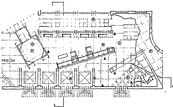
ampliación lobby escala 1/30
