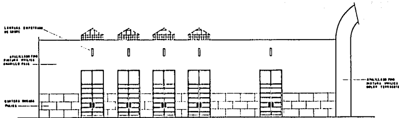
ampliación fachada principal
