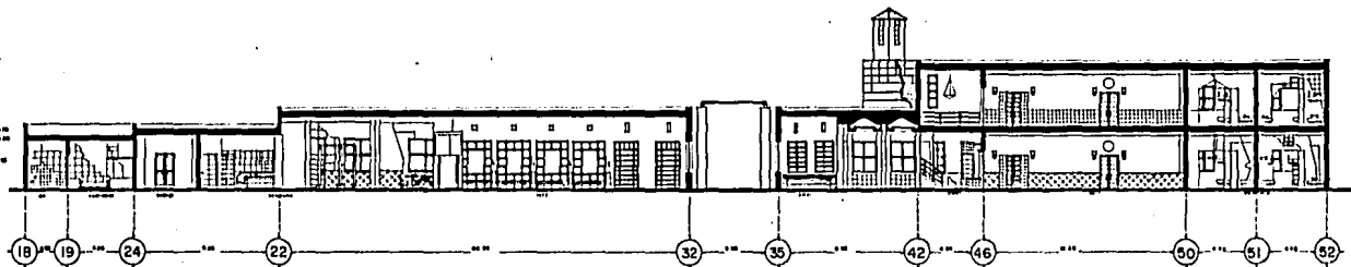
CORTE A-A'
