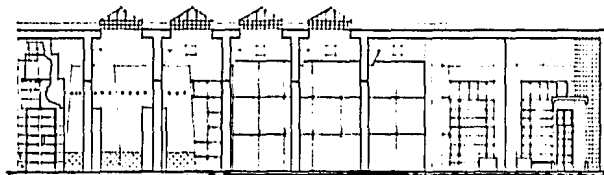
corte aa' escala 1/30
