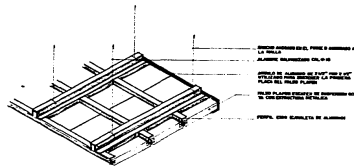
DETALLE UNION DE PERFILES.
