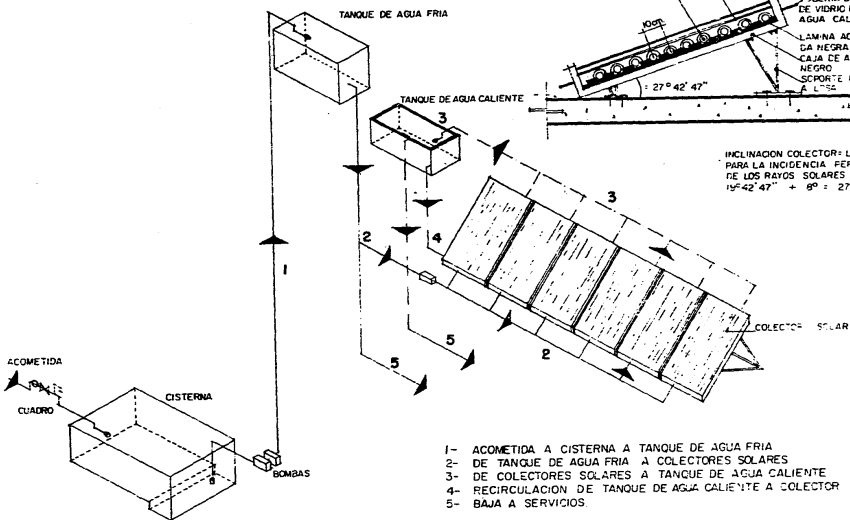
SISTEMA INSTALACION HIDRAULICA CON COLECTORES SOLARES. (area servicios).
