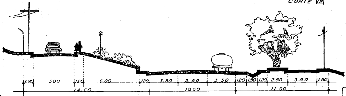
CORTE 12
