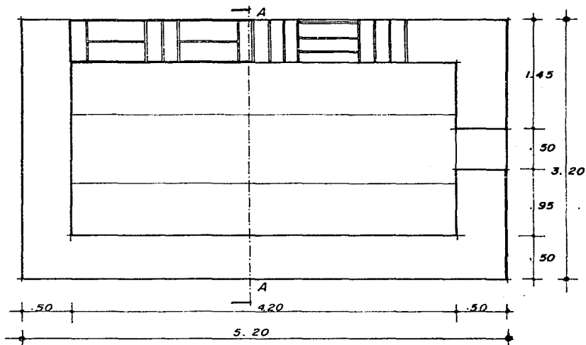
PLANTA TIPO.
