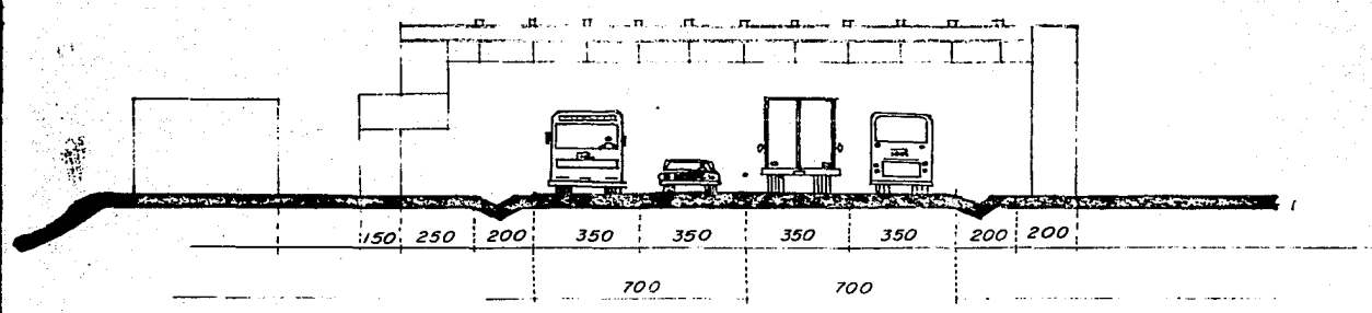
Corte en el acceso a Sn. Andrés A-A'
