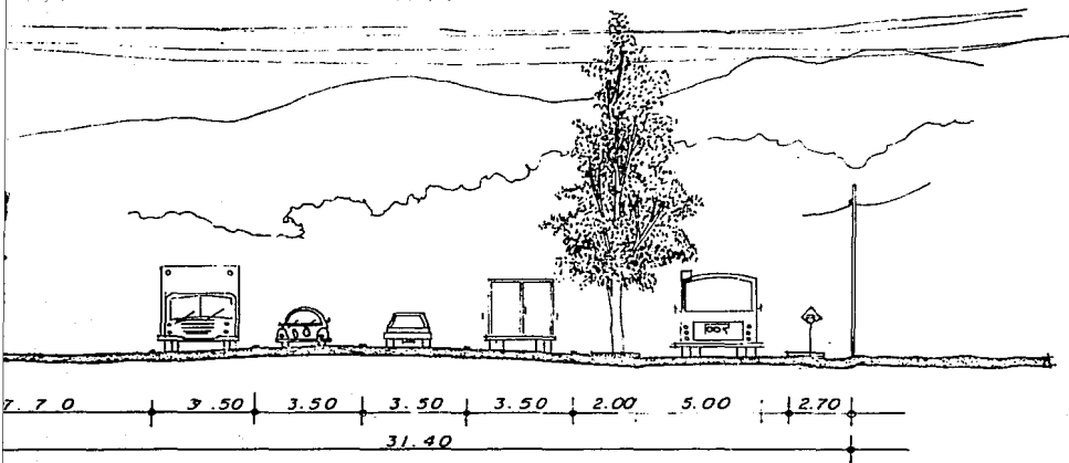
Corte. 4
