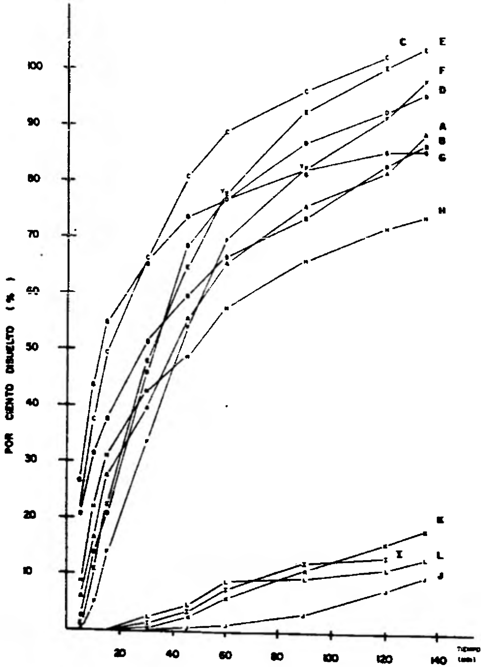
FIG. 6 PERFIL DE DISOLUCION DE 12 PRODUCTOS COMERCIALES METODO PROPELAS 50 R.P.M.
