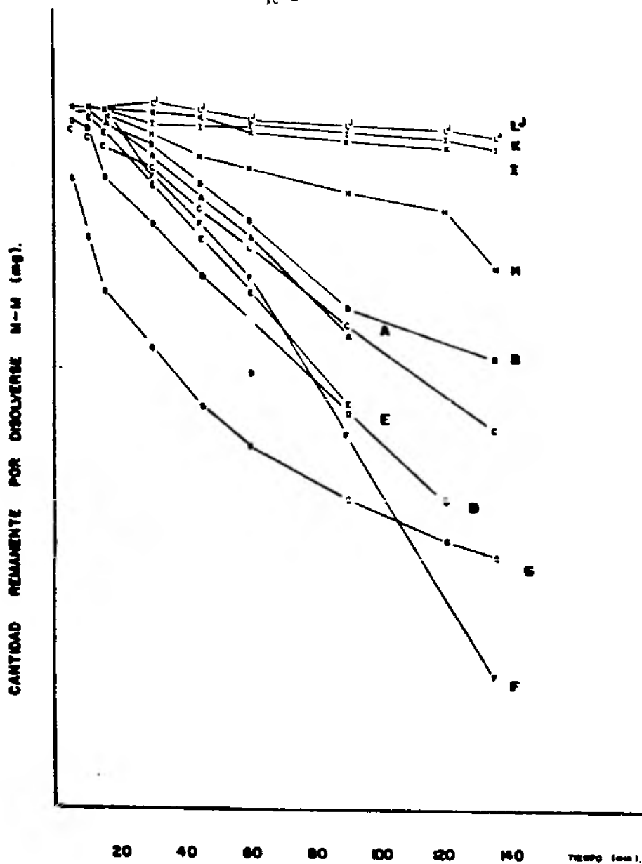
FIG. 12. CONSTANTE DE DISOLUSION DE 12 PRODUCTOS DE CLORAMFENICOL "PROPELAS" 25 R.P.M.
