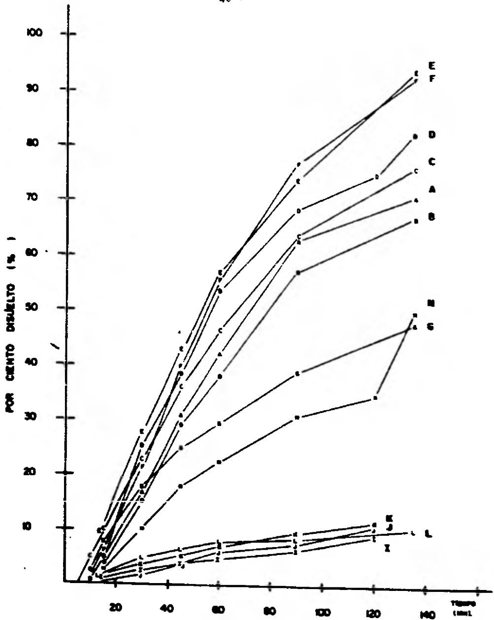
FIG. 7. PERFIL DE DISOLUCION DE 12 PRODUCTOS COMERCIALES METODO PROPELAS 25 R.P.M.
