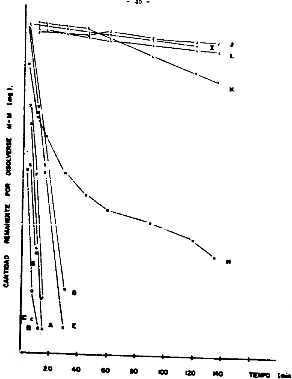
FIG. 10 CONSTANTES DE DISOLUCION DE 12 PRODUCTOS DE CLORAMFENICOL "PROPELAS" 75 R.P. II
