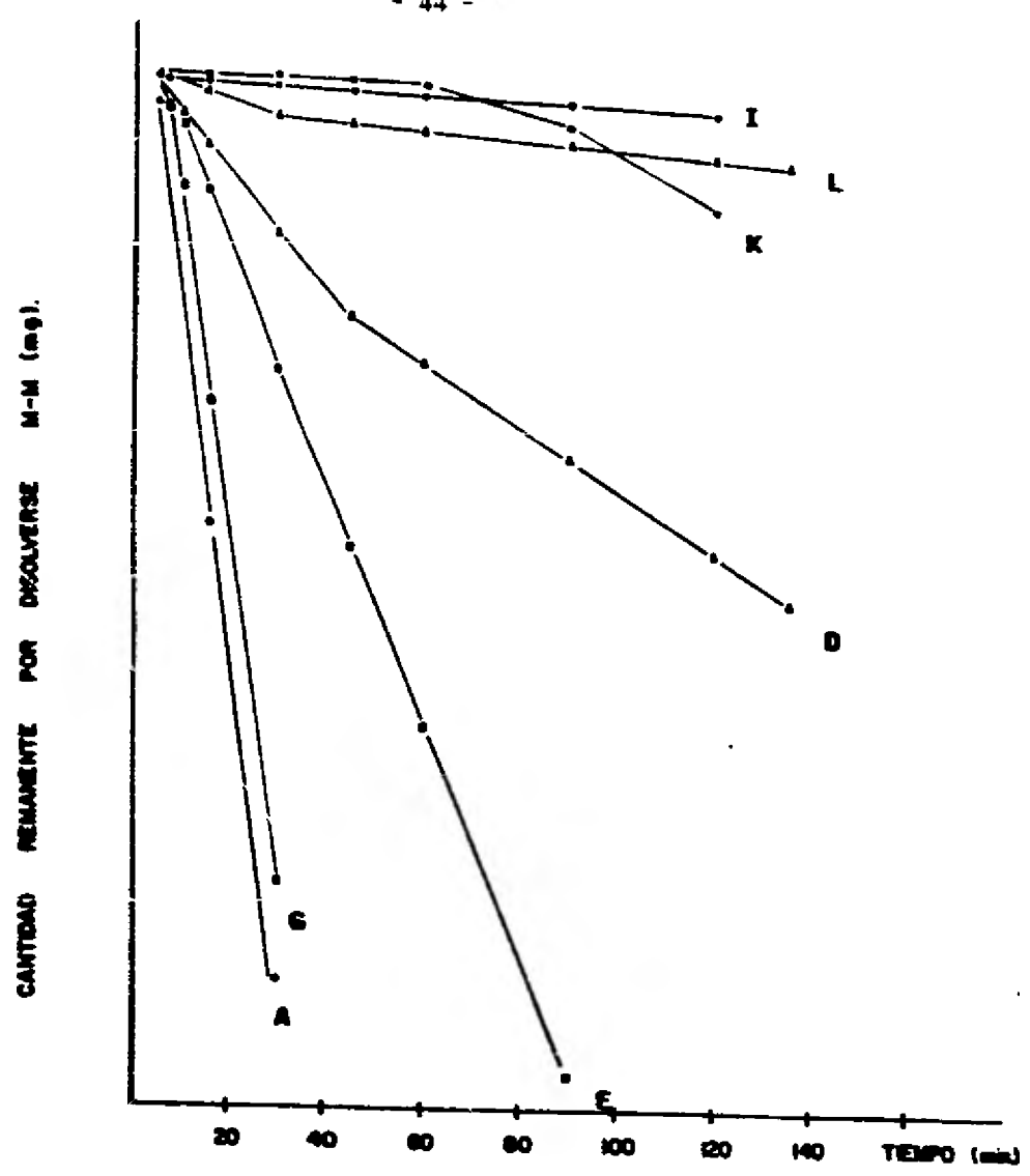
Fig. N.º 9 CONSTANTE DE DISOLUCION DE 7 PRODUCTOS DE CLORAMFENICOL "CAJASTILLAS" 100 R.P.M
