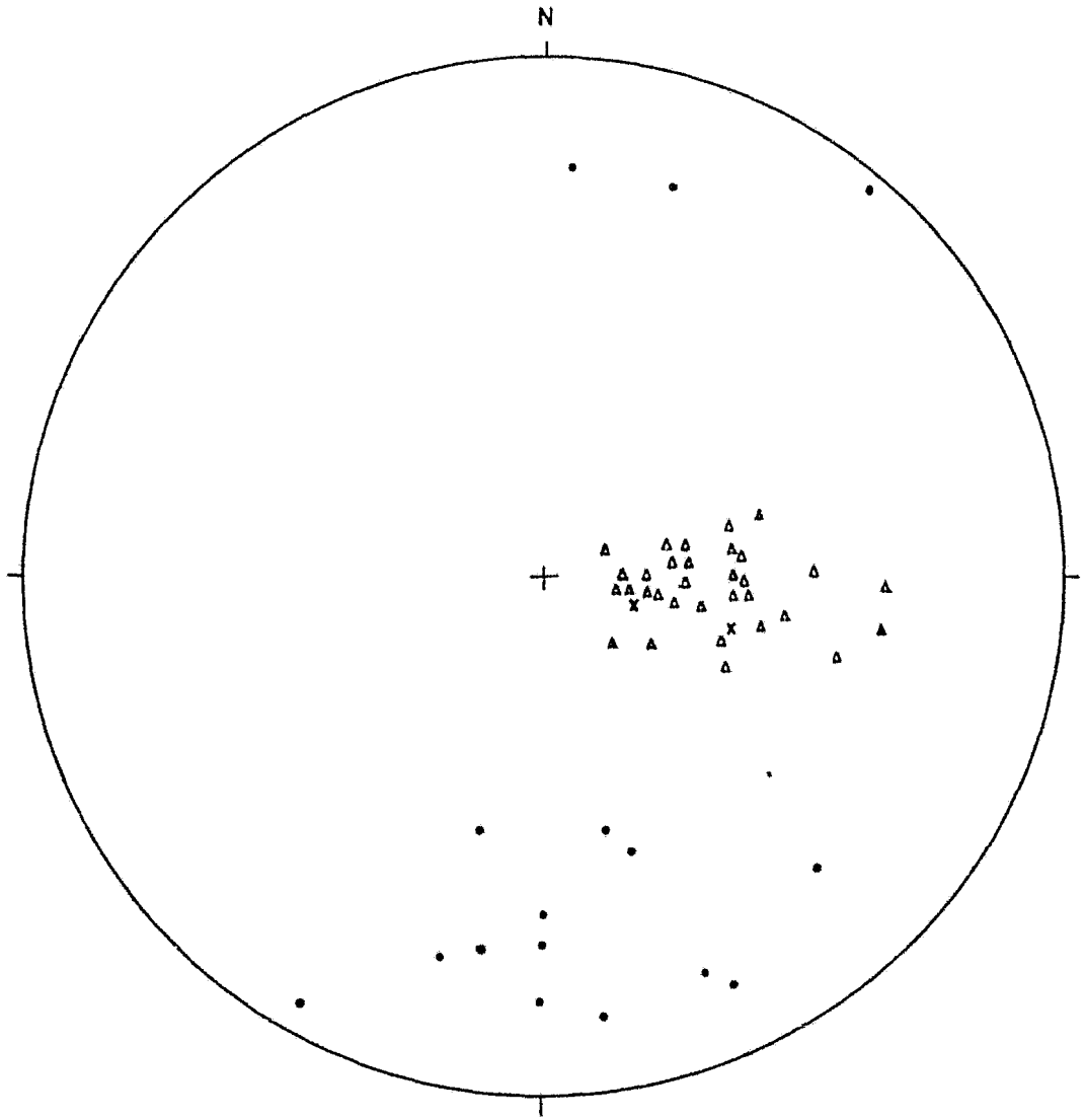
DIAGRAMA DE POLOS PARA LA ELEV.500
