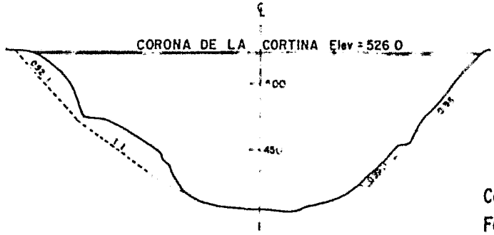
PERFIL DEL EJE DE SIMETRIA
