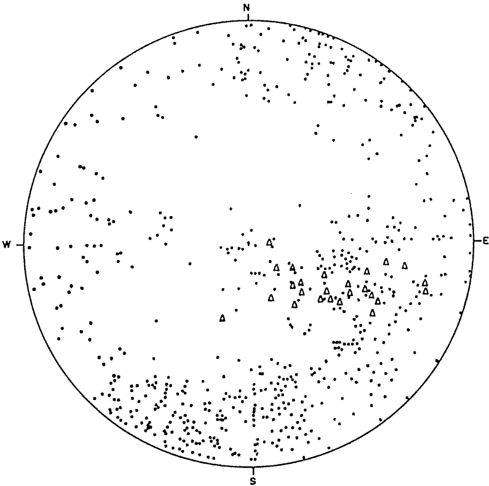
DIAGRAMA DE FRACTURAMIENTO DEL SITIO DE LA OBRA POR EL METODO DE POLOS.
