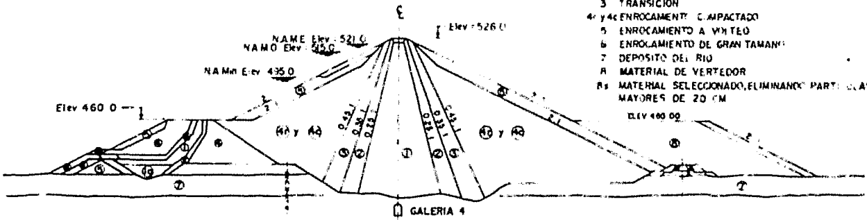
SECCION MAXIMA
