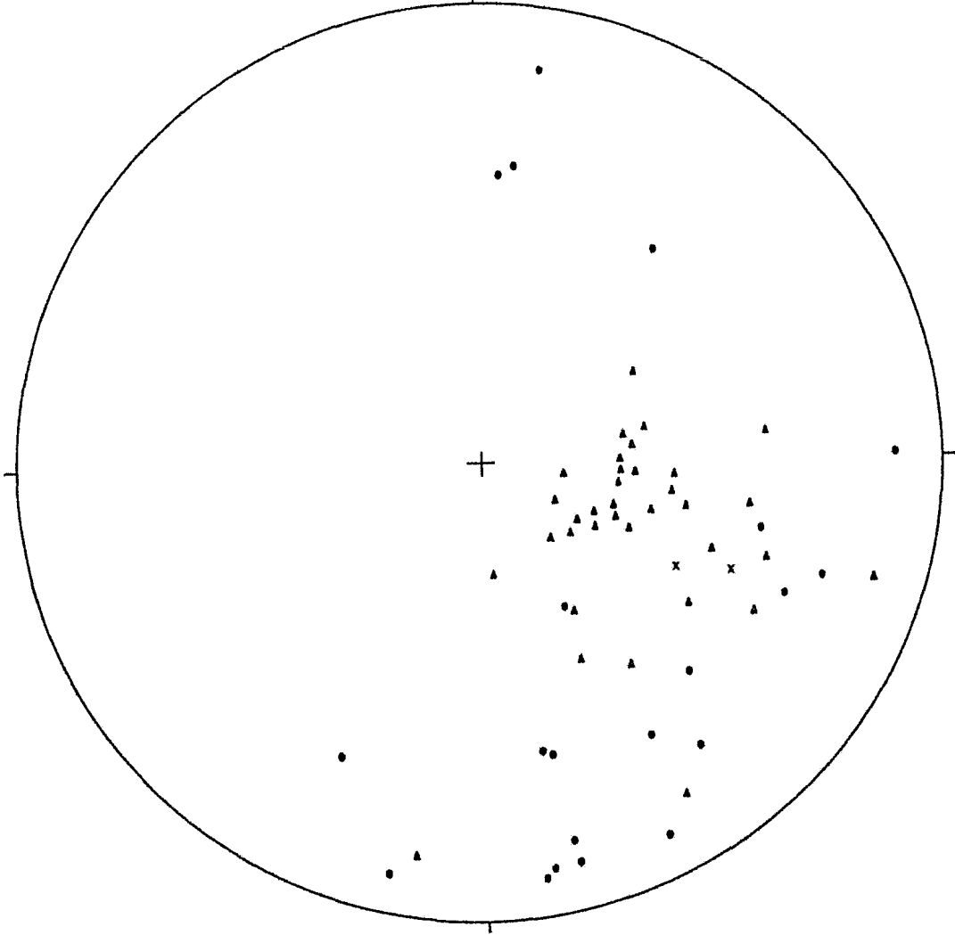
DIAGRAMA DE POLOS PARA LA ELEV. 460
