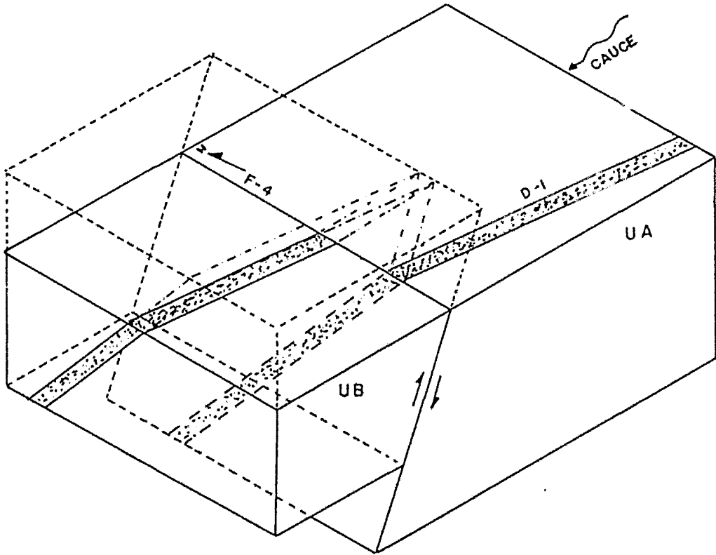
BLOQUE DIAGRAMA PARA FALLA INVERSA
