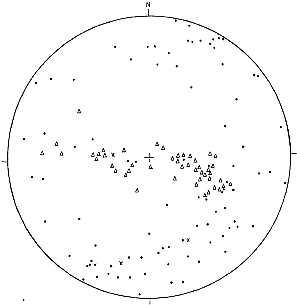
DIAGRAMA DE POLOS DE DISCONTINUIDADES PARA CALCULO DE ORIENTACION DE BARRENOS EN LA PANTALLA PRINCIPAL DE M. D.
