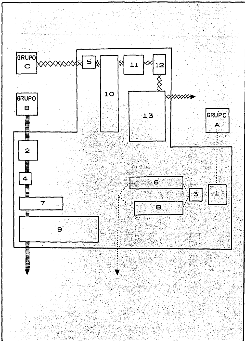
Fig.21. Distribución de planta propuesta para la Industria Nacional productora de partes metálicas (6).
