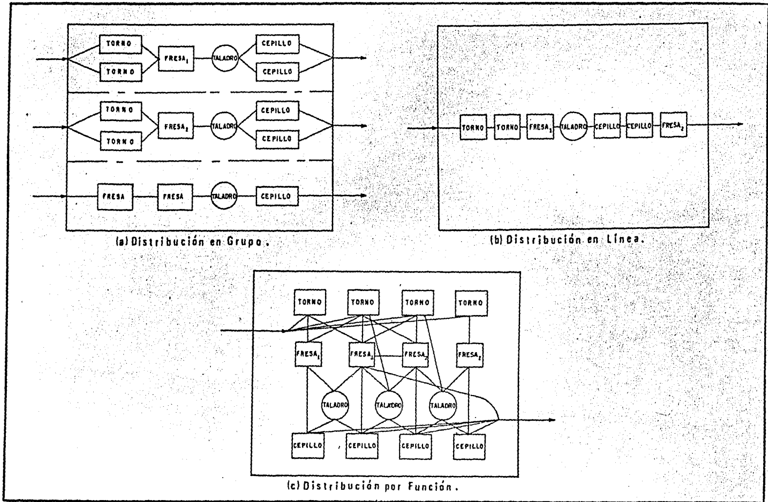
Fig.3. Principales tipos de distribución en la Industria Manufacturera.
