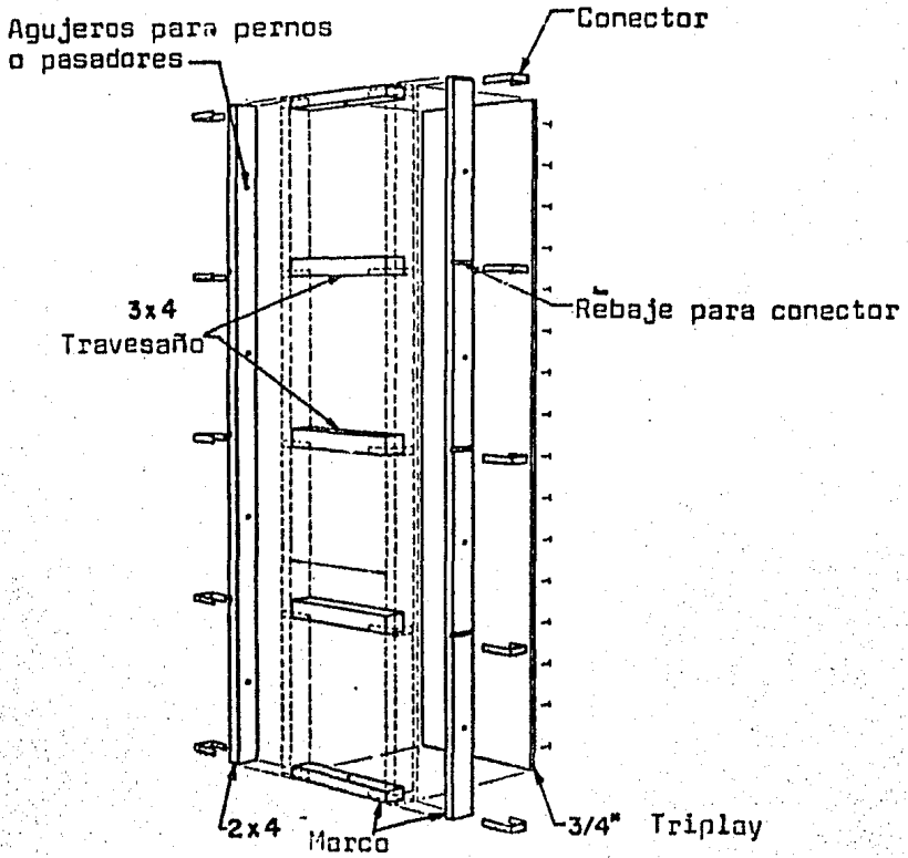
Ensamble típico de cimbra de muro
