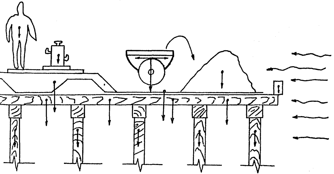
Cargas y presiones sobre una cimbra
