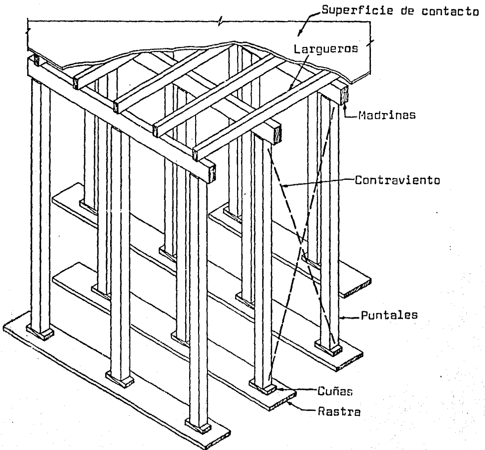
Componentes típicos para cimbra de losas.
