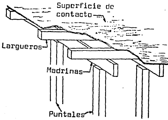
Cimbra típica de losa
