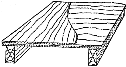
Triplay usado en la dirección menos resistente.
