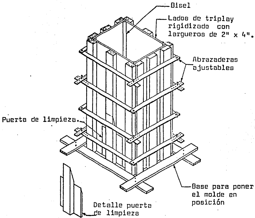
Cimbra típica para columnas
