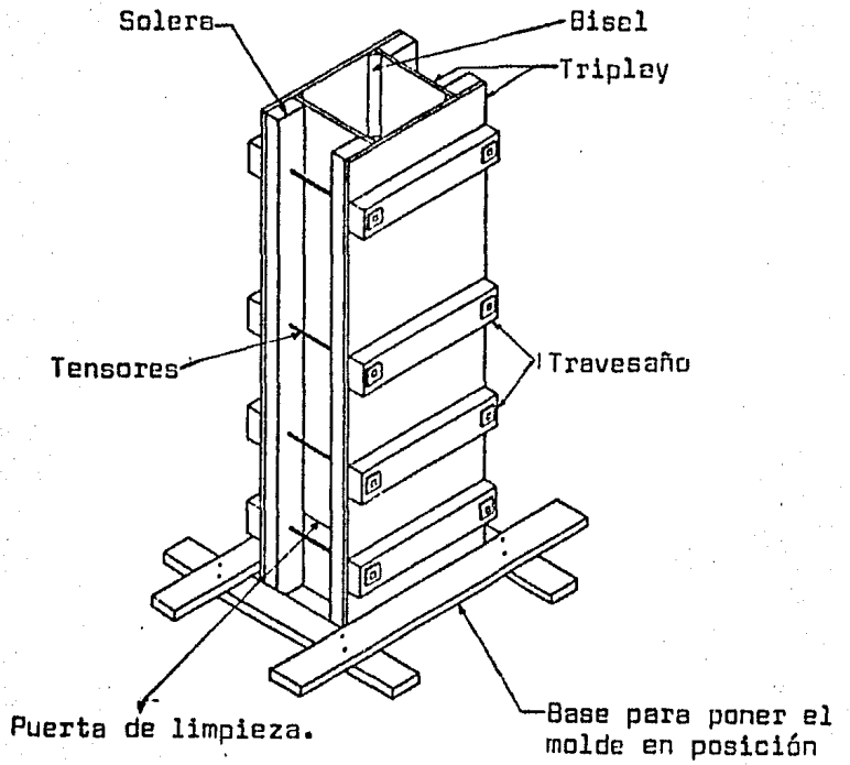
Cimbra típica para columnas ligeras.
