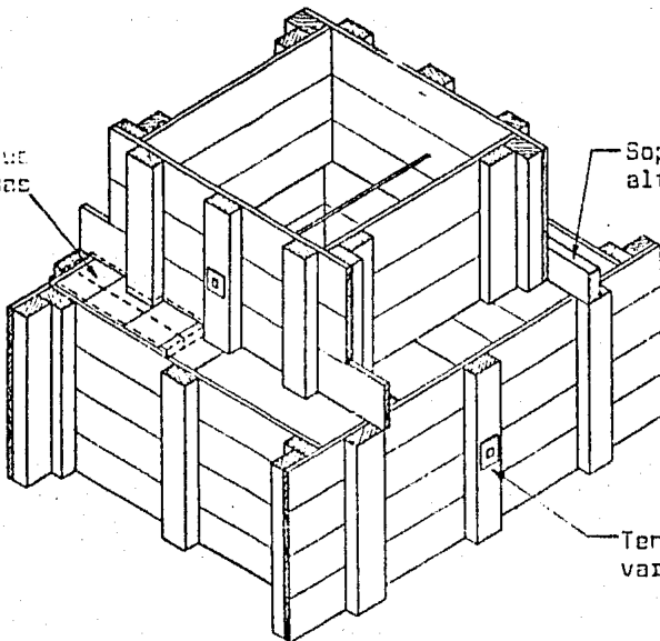
Cimbra para zapata y caca
