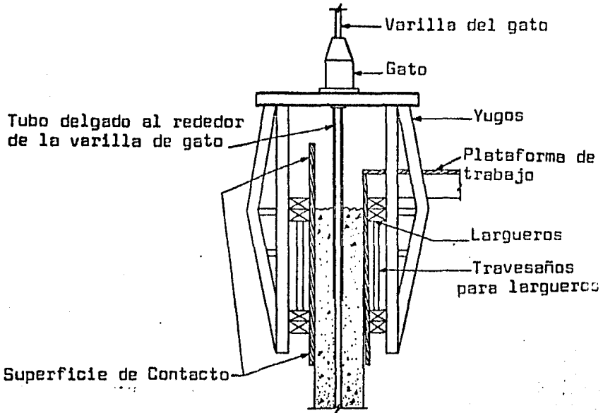
Sección Transversal de cimbra deslizante
