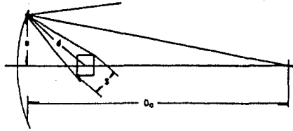
FIG. 3-20 DIAGRAMA QUE MUESTRA LAS DISTANCIAS Y DIMENSIONES UTILIZADAS PARA DETERMINAR LA DISTANCIA MINIMA PARA APLICAR LA LEY DEL CUADRADO INVERSO.
