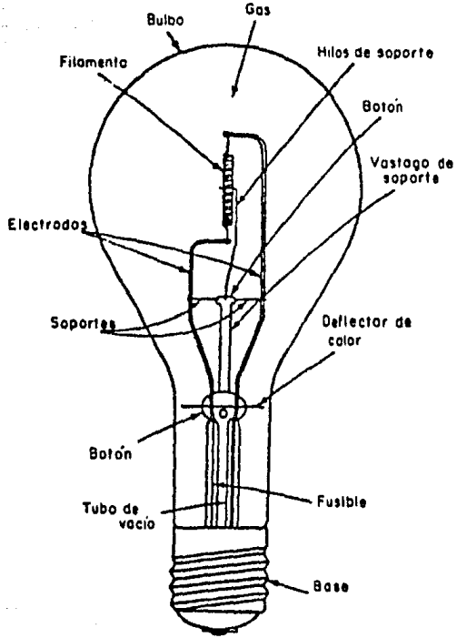
Figura 3-22 Lámpara Incandescente
