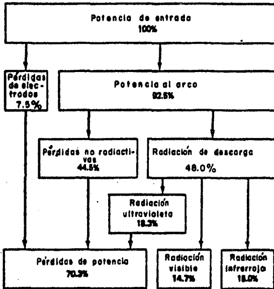
Figura 3-41 Distribución de Energía para Lámpara de Vapor de Mercurio con 56.3 lm/watt (400 w).
