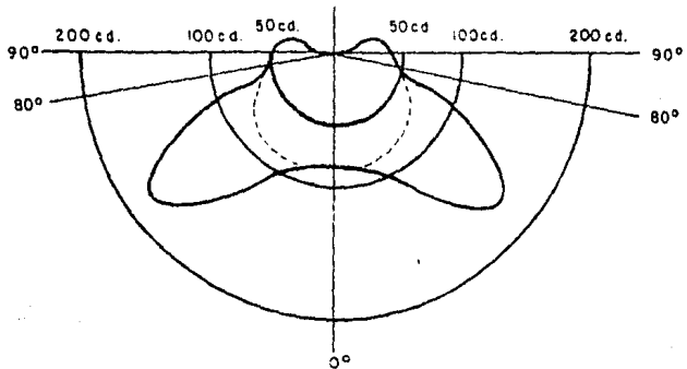
b) SEMI CUT-OFF (HAZ SEMI-RECORTADO)
