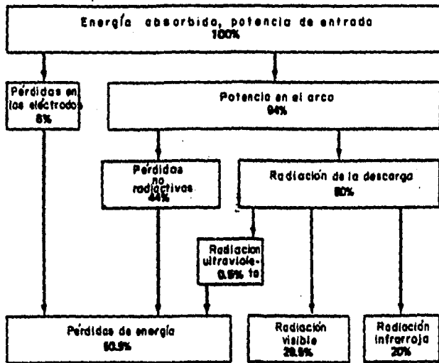
Figura 3-48 Distribución de Energía para la Lámpara de Sodio Alta Presión con 125 lm/watt y 29.5% de radiación Visible.
