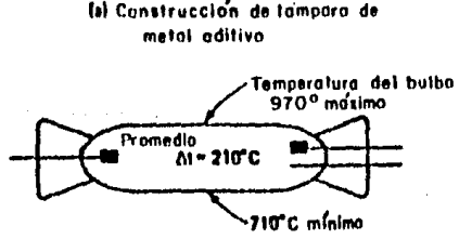
Figura 3-42 Variación de Temperatura Interna y Temperatura de la Pared, de una Lámpara de Aditivos Metálicos.
