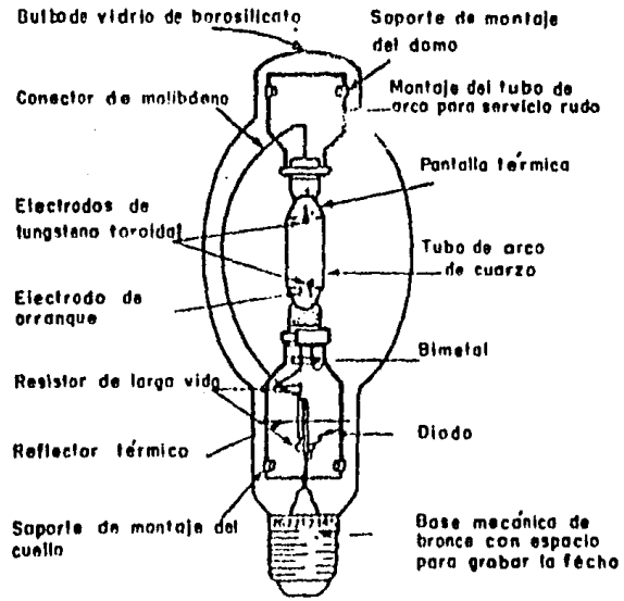
(a) Construcción de lámpara de metal aditivo
