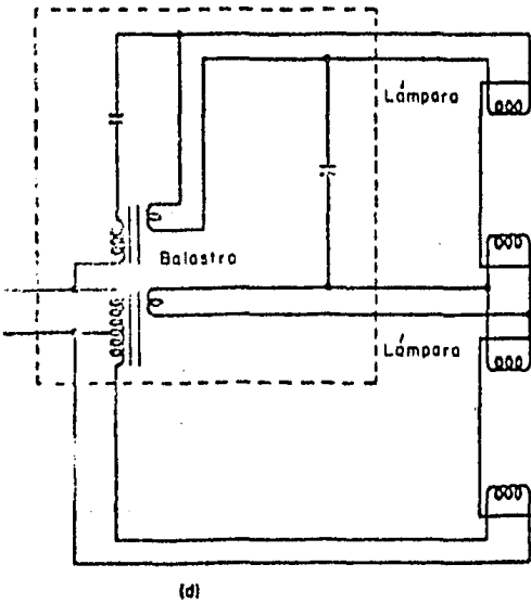
Figura 3-49 Circuitos Típicos de Balastros Fluorescentes.
