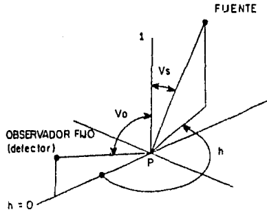
Figura 3-5 MEDICION DE LA FUNCION DE DISTRIBUCION DE REFLECTANCIA BIDIRECCIONAL
