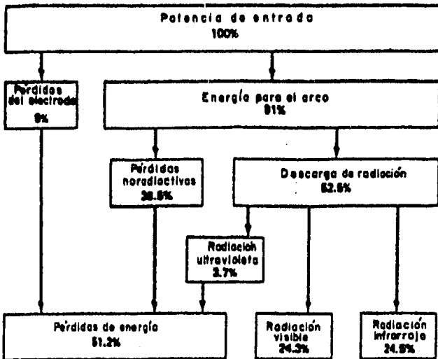
Figura 3-45 Distribución de Energía en una Lámpara de Aditivos Metálicos con 100 lm/watt y 24.3% de Radiación Visible.
