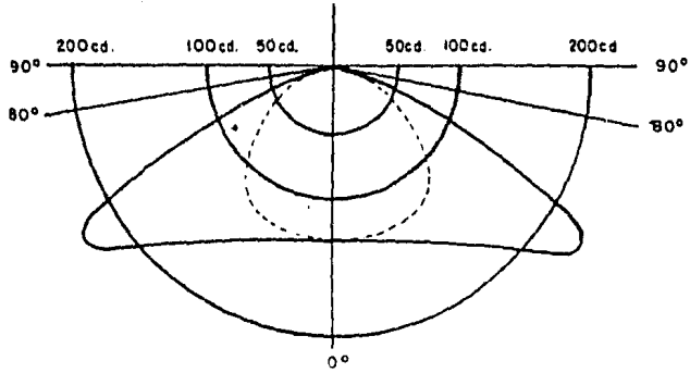
a) CUT-OFF (HAZ REORTADO)
