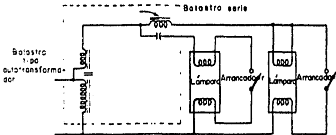
(b) Circuito de precalentamiento en atraso-adelanto
