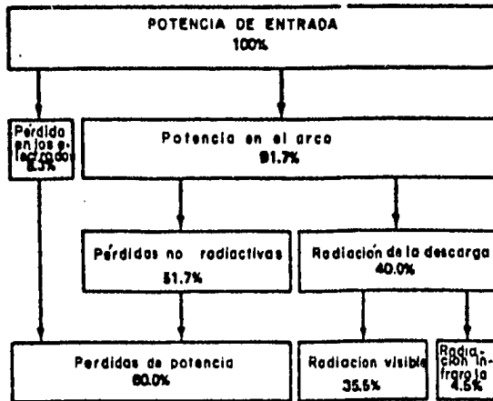
Figura 3-34 Distribución de Energía de una Lámpara de Sodio Baja Presión con 180 lm/watt y 35.5% de radiación Visible.
