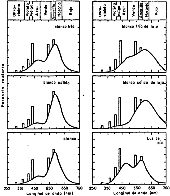
Figura 3-30 Distribución de Potencia Espectral de las Lámparas Fluorescentes Estandar.
