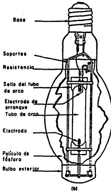
Figura 3-35 Lámpara de Vapor de Mercurio y Tubo de Arco.
