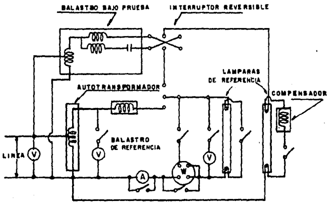
FIG. 3-16. CIRCUITO PARA COMPARAR EL FUNCIONAMIENTO DE LAMPARAS FLUORESCENTES CON DOS BALASTROS DIFERENTES.
