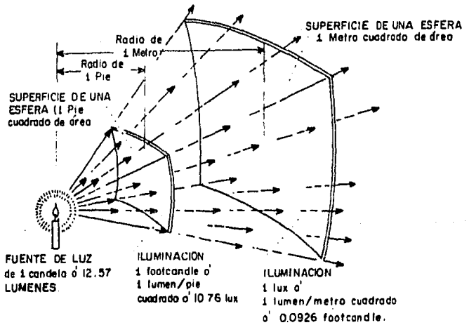
Figura 3-3 Iluminacion.
