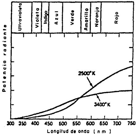
Figura 3-26 Distribución de Potencia Espectral de una Lámpara Incandescente.
