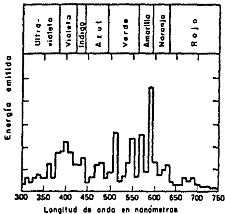
Figura 3-43 Distribución de Potencia Espectral de una Lámpara de Aditivos Metálicos.
