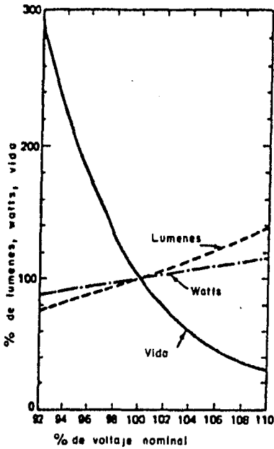
Figura 3-24 Efecto del Voltaje en la Emisión Lumínica y Vida de la Lámpara.
