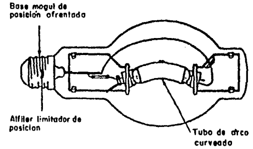
(b) Lámpara de encendido horizontal
