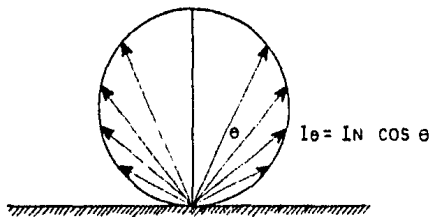
FIG. 3-1 LEY DE LOS COSENOS DE LAMBERT (Difusor perfecto).
