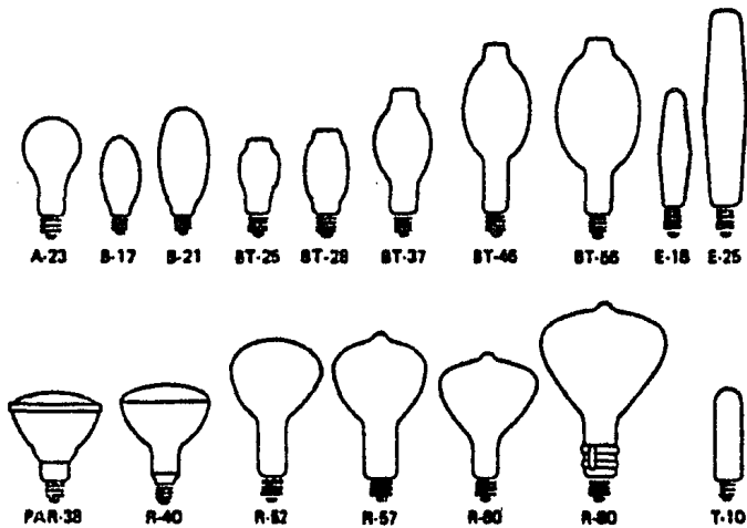
Figura 3-37 Designación de las Formas de Bulbos para Lámparas de Descarga de Alta Intensidad.
