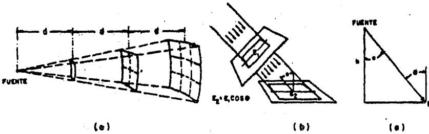
FIG. 3-9 : (a) ILUSTRACION DE LA LEY DEL CUADRADO INVERSO EN LA CUAL SE MUESTRA COMO EL FLUJO DE LUZ SE DISTRIBUYE EN UNA GRAN AREA CONFORME LA DISTANCIA DE LA FUENTE A LA SUPERFICIE AUMENTA. (b) LA LEY DEL COSENO DE LAMBERT QUE MUESTRA QUE LA LUZ QUE INCIDE EN UNA SUPERFICIE A ANGULOS DIFERENTES A LA NORMAL SE DISTRIBUYE EN UNA GRAN AREA. (c) EXPLICACION DE LA LEY DEL COSENO CUBICO.
