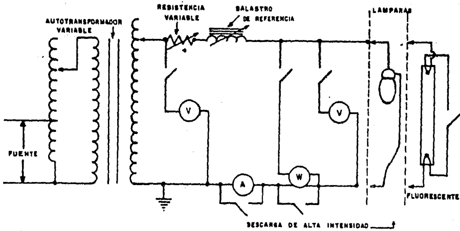
FIG. 3-15. CIRCUITO BÁSICO DE MEDICIÓN PARA LAMPARAS Y BALASTROS DE DESCARGA ELECTRICA.
