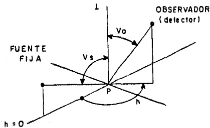
Figura 3-6 MEDICION DE LA INTENSIDAD LUMINOSA REFLEJADA
