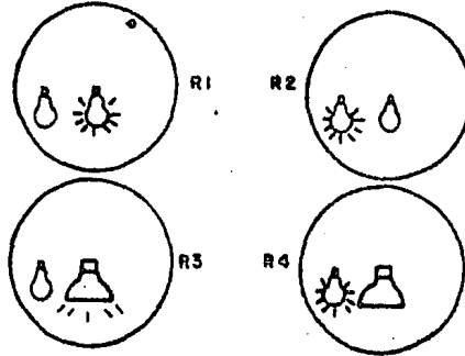
FIG. 8-17 POSICIONES DE LÁMPARA Y LUMINARIO DENTRO DE UNA ESFERA INTEGRADORA PARA DETERMINAR LA EFICIENCIA DE UN LUMINARIO POR EL METODO RELATIVO. EL DIAMETRO DE LA ESFERA DEBE SER AL MENOS 605 VECES MAYOR QUE LA DIMENSION MAXIMA DEL LUMINARIO O VA A SER EVALUADO.
