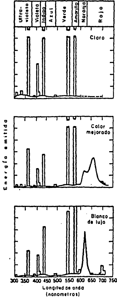
Figura 3-36 Curvas de Distribución de Potencia -- Espectral, para Lámparas de Vapor de Mercurio
