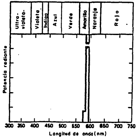
Figura 3-33 Distribución de Potencia Espectral para una Lámpara de Sodio Baja Presión.
