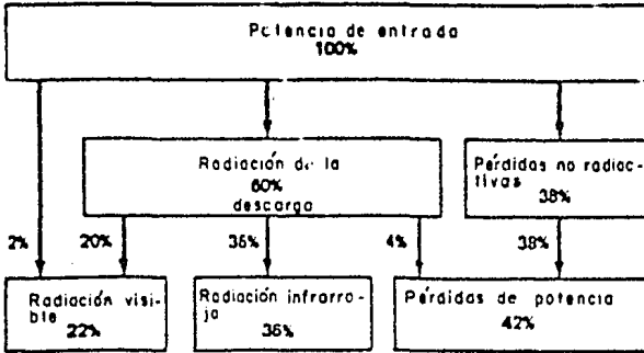
Figura 3-32 Distribución de Energía en una Lámpara Fluorescente con 78.8 lm/watt (40 watts) y con 22% de Radiación Visible.
