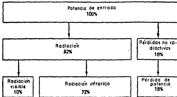
Figura 3-27 Distribución de Energía de una Lámpara Incandescente.
