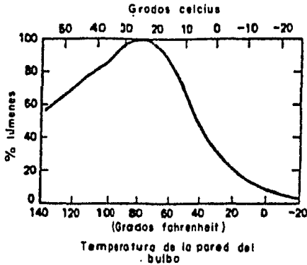
Figura 3-31 Efecto de la Temperatura en las Lámparas Fluorescentes.
