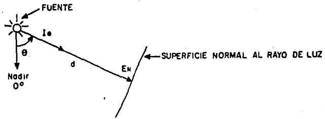
Figura 3-4 Ley del cuadrado inverso
