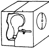
FIG. 3-21 FUENTE AJUSTABLE DE LUMINANCIA, UTIL CUANDO SE CALIBRAN DISPOSITIVOS DE MEDICION DE LUMINANCIA QUE TENGAN ABERTURAS DE DIFERENTES FORMAS. D ES DE ALRREDEDOR DE 76mm. (3").
