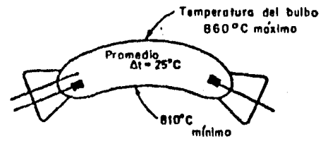
Figura 3-42 Variación de Temperatura Interna y Temperatura de la Pared, de una Lámpara de Aditivos Metálicos.
