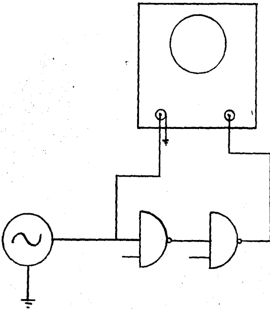
Fig. 4.7 Circuito Prueba de histéresis.
