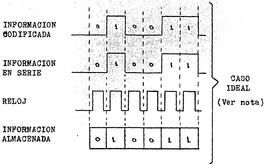
Fig. 3.4 Lectura ideal código de barras.
