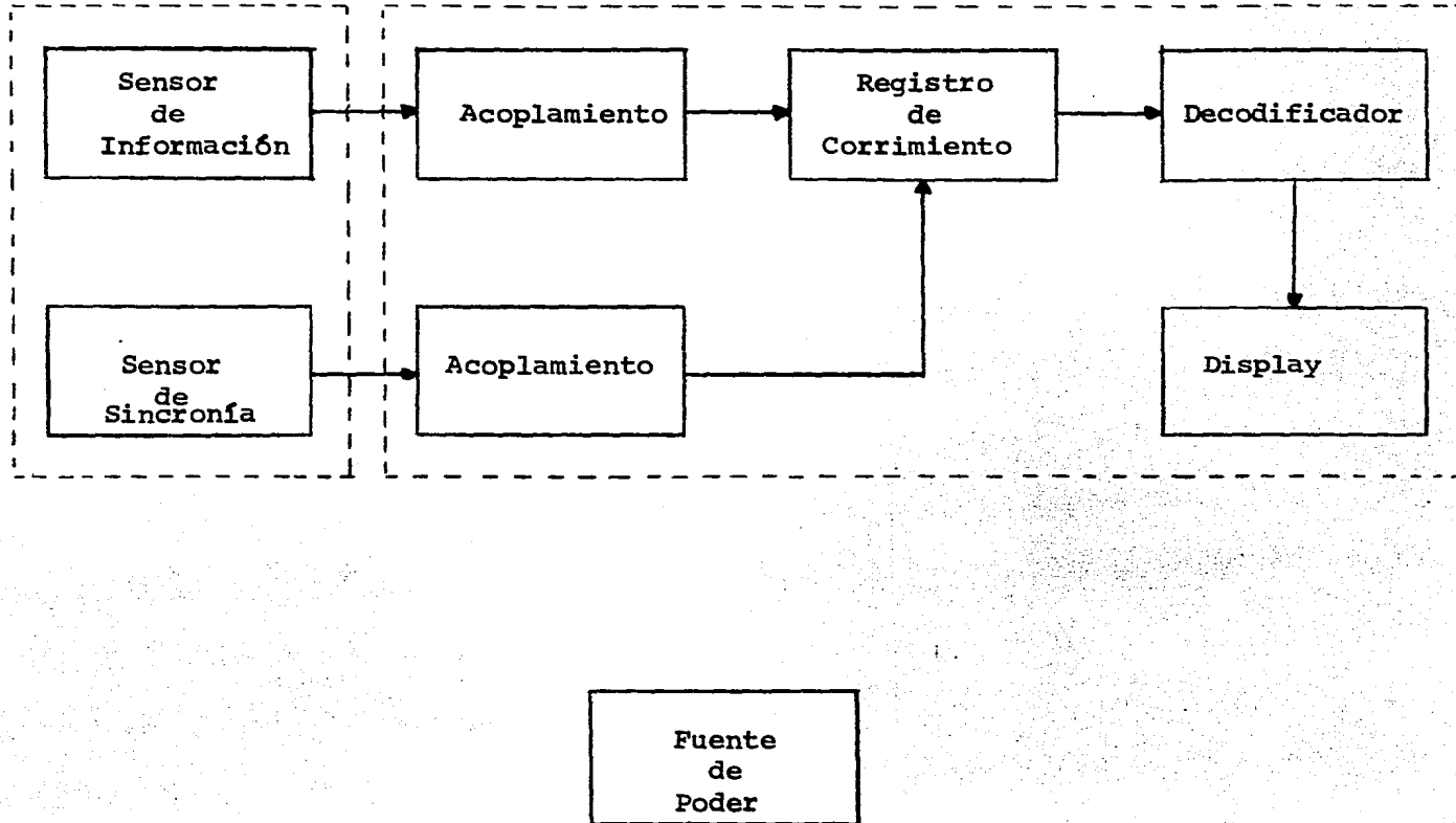
Fig. 4.1 Diagrama General.
