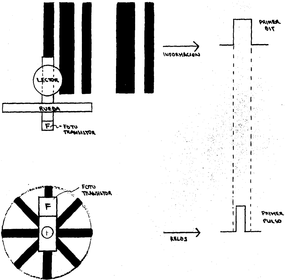
Fig. 3.8. Funcionamiento de sincronía.
