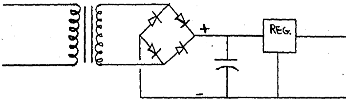
Fig. 4.20 Circuito de la fuente completo
