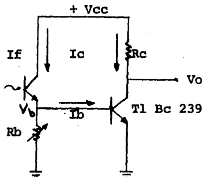
Fig. 4.5 Acoplamiento del sensor.
