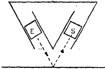
Fig. 4.2 Disposición del sensor-emisor.
