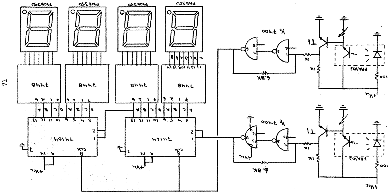
Fig. 4.26 DIAGRAMA ELECTRONICO GENERAL.
