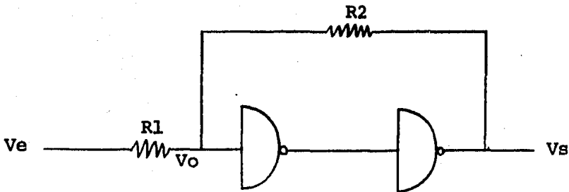
Fig. 4.9 Circuito de histéresis realimentado.
