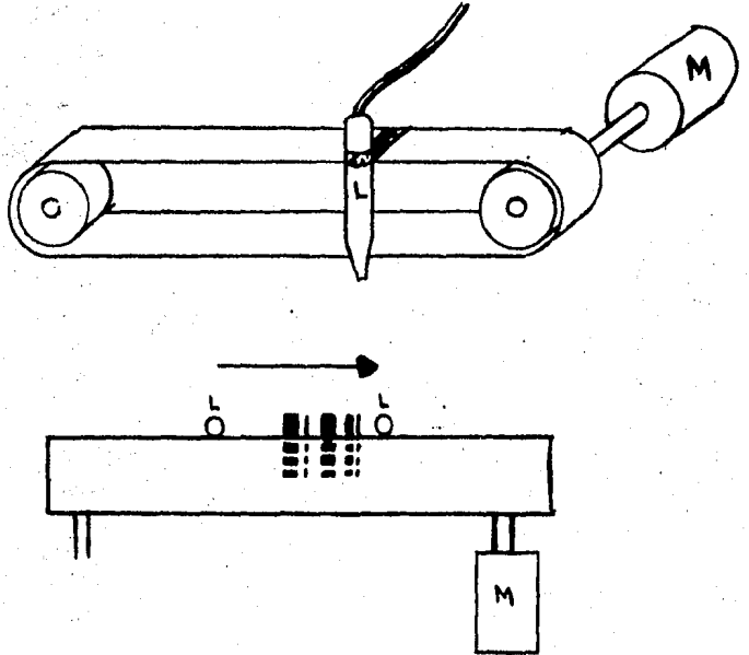
Fig. 3.6 Método de sincronía con motor.
