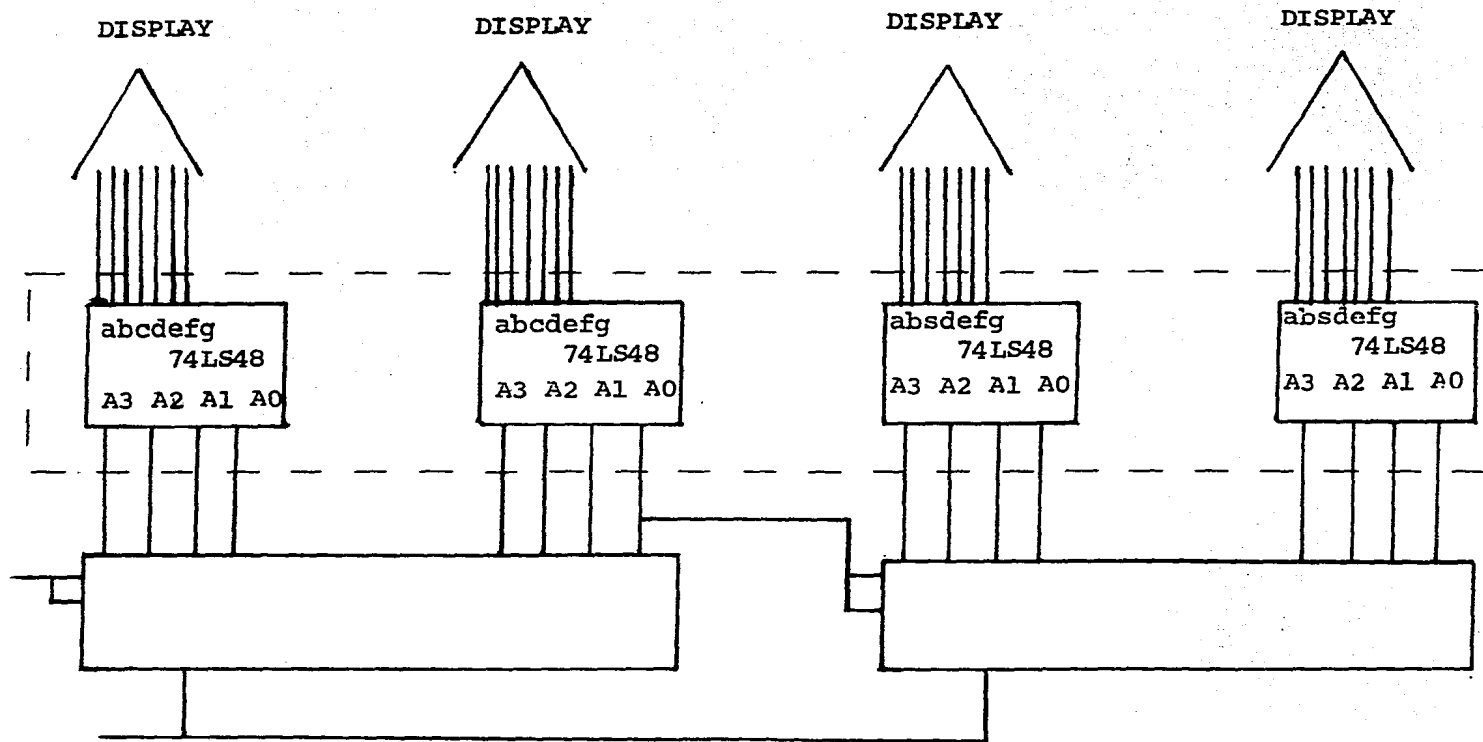
Fig. 4.15 Diagrama bloq.ue decodificador.
