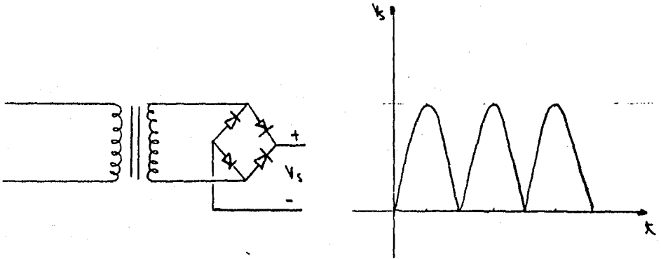
Fig. 4.17 Rectificador onda completa.
