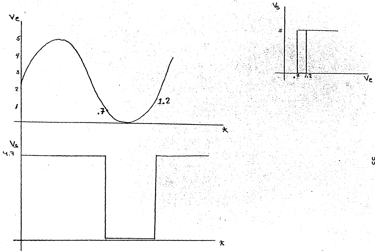
Fig. 4.10 Ampliación de la histéresis con la realimentación.
