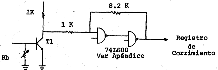
Fig. 4.11 Circuito del bloque acoplamiento.
