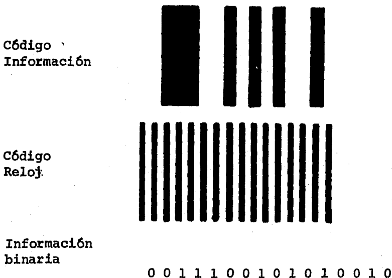
Fig. 3.9 Código de barras usado.
