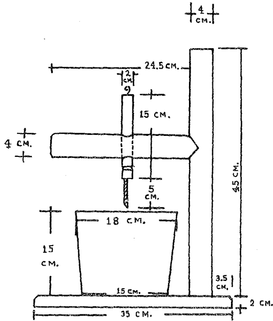
PENETROMETRO.
