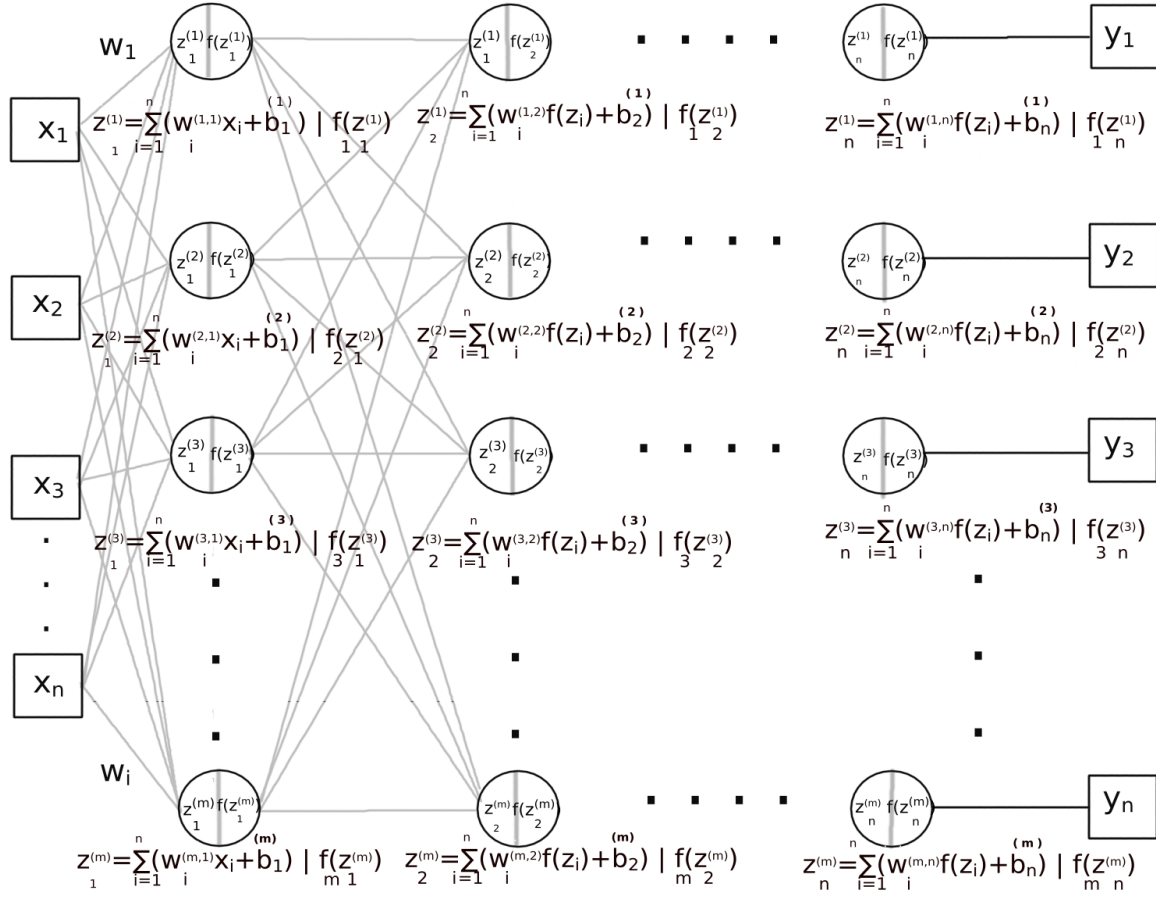
Figura 3.3.1: Representación gráfica de un perceptrón multicapa
