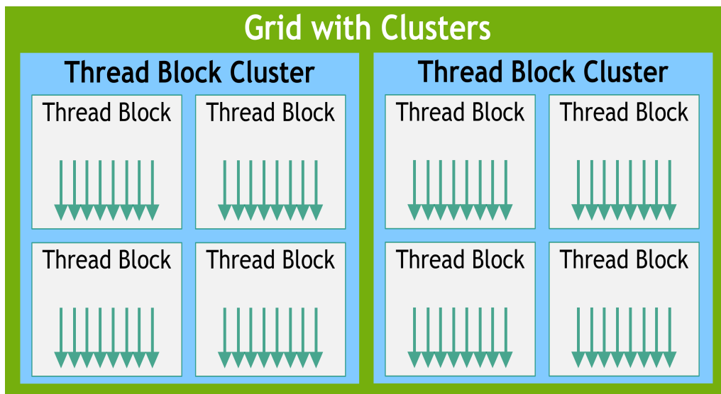
Figura 8.2.4: Grupo de núcleos CUDA
