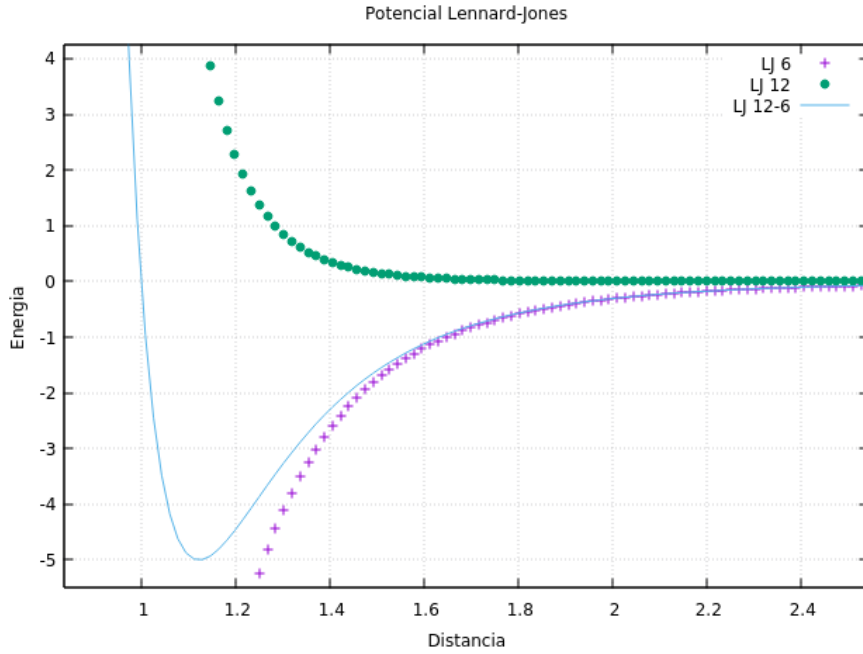
Figura 2.2.1: Gráfica de las energías de Lennard-Jones
