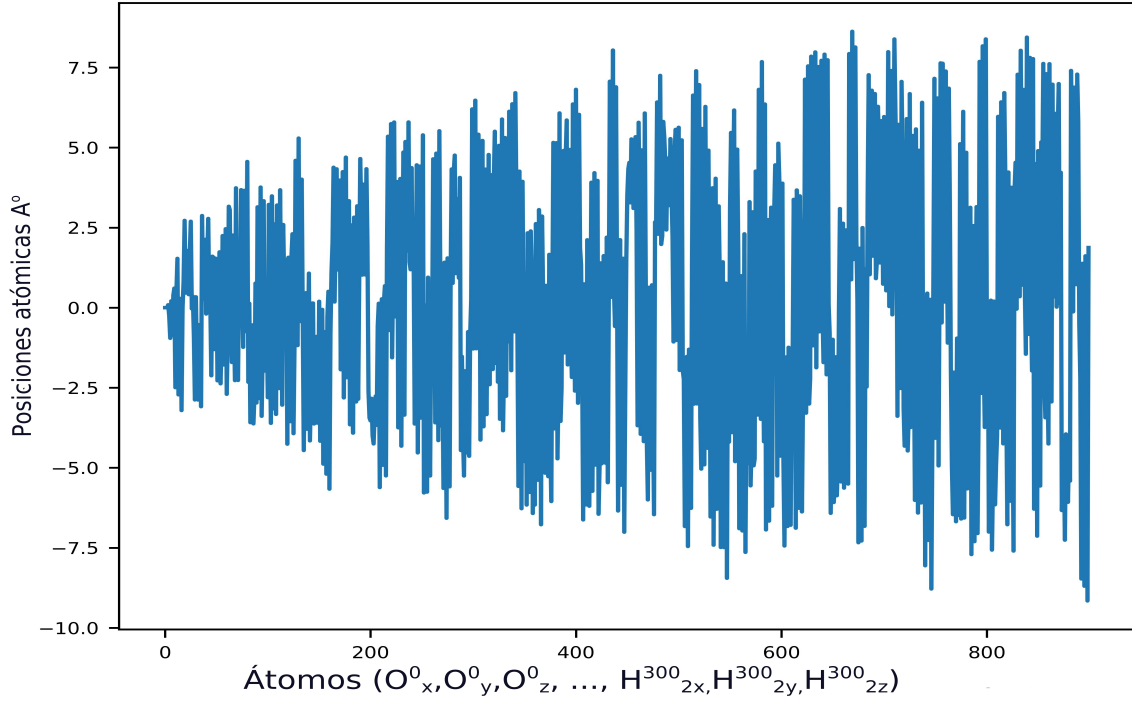
Figura 4.1.1: Distribución y posicionamiento al origen del primer vecindario en el cuadro de tiempo t = 0
