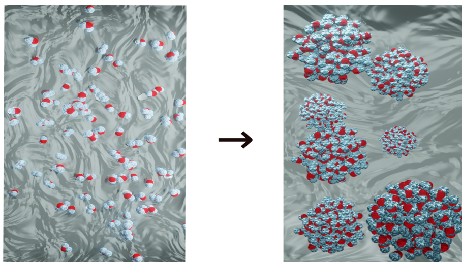
Figura 4.0.5: Partición del contenedor de agua donde, cada cúmulo simboliza un vecindario
