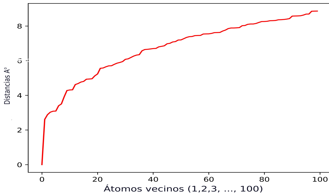
Figura 4.1.5: Distribución de las distancias del primer vecindario
