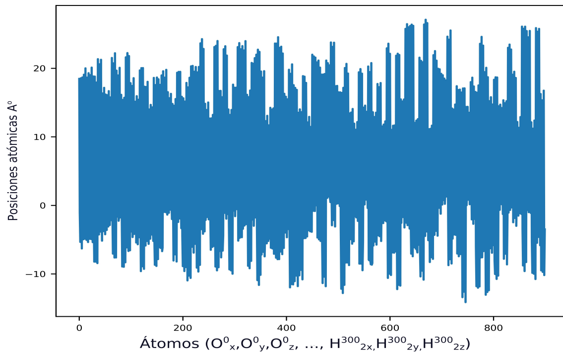
Figura 4.0.6: Distribución del primer vecindario respecto al oxígeno central en el cuadro de tiempo t = 0
