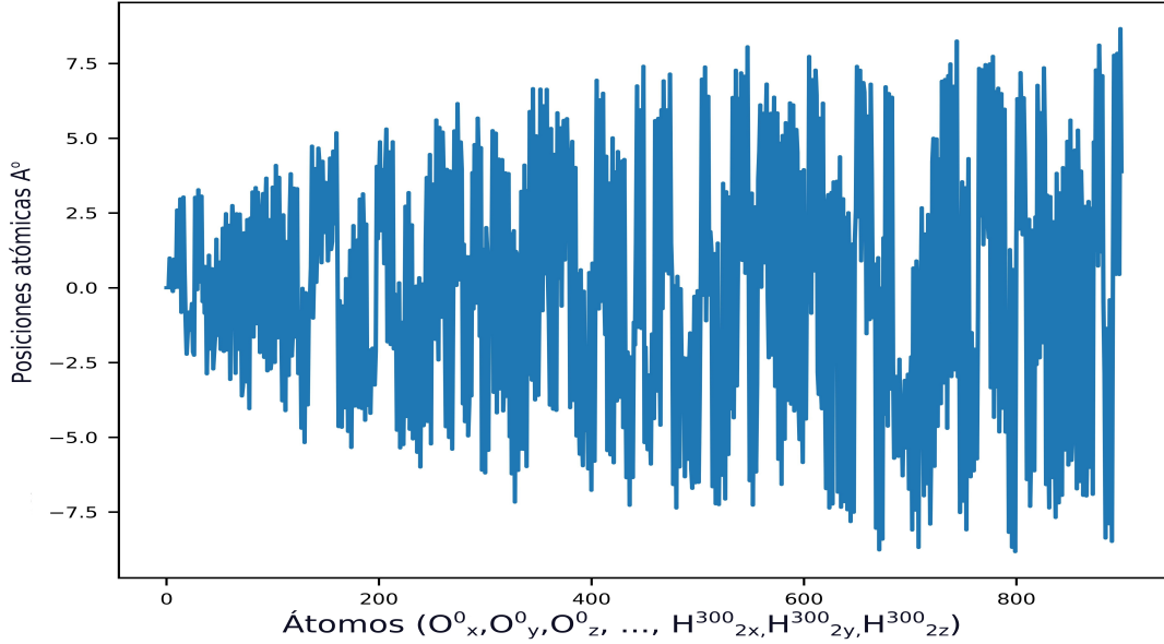
Figura 4.1.2: Distribución tras la rotación sobre los ejes y, z del primer vecindario en el cuadro de tiempo t = 0
