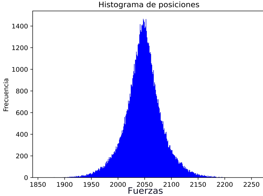
Figura 4.4.2: Distribución de las fuerzas totales de forma individual
