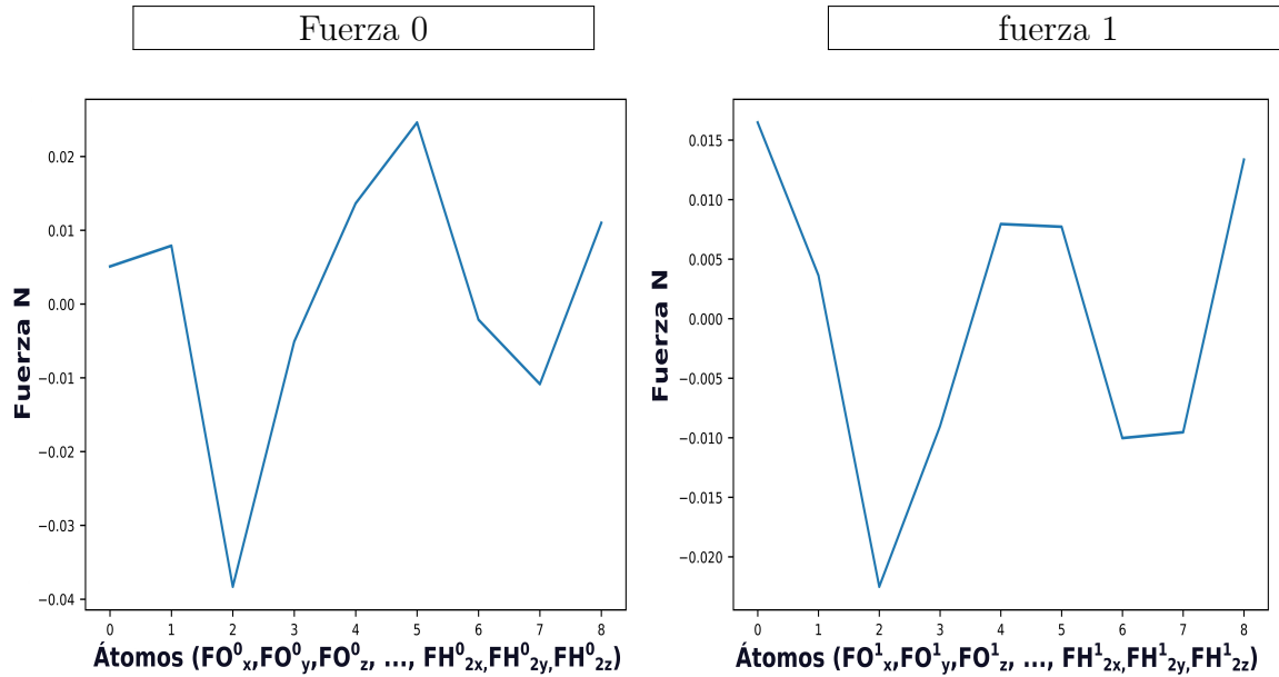
Figura 4.4.1: Distribución de las fuerzas totales en una molécula de agua en el cuadro de tiempo t = 0
