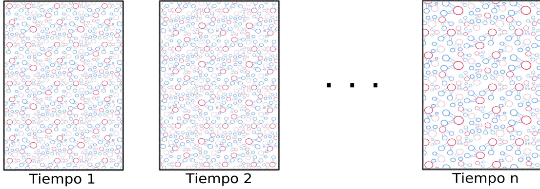
Figura 4.0.2: Diferentes cuadros de tiempo t_1, t_2, \dots, t_n
