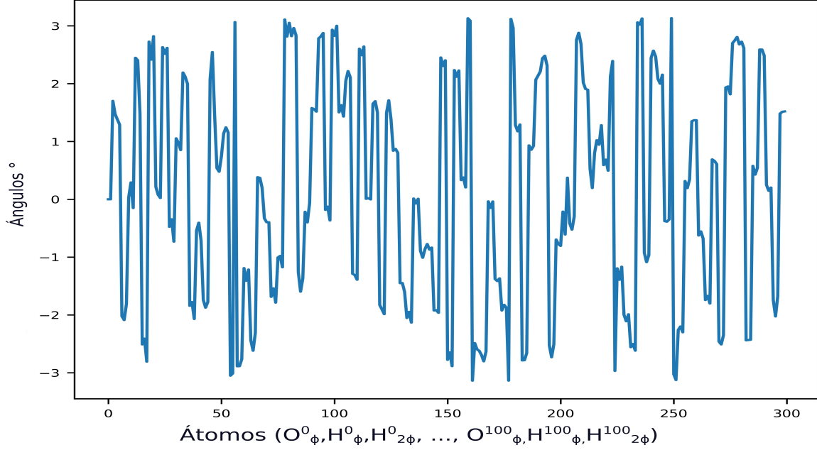
Figura 4.1.7: Distribución en \phi del primer vecindario en el cuadro de tiempo t = 0
