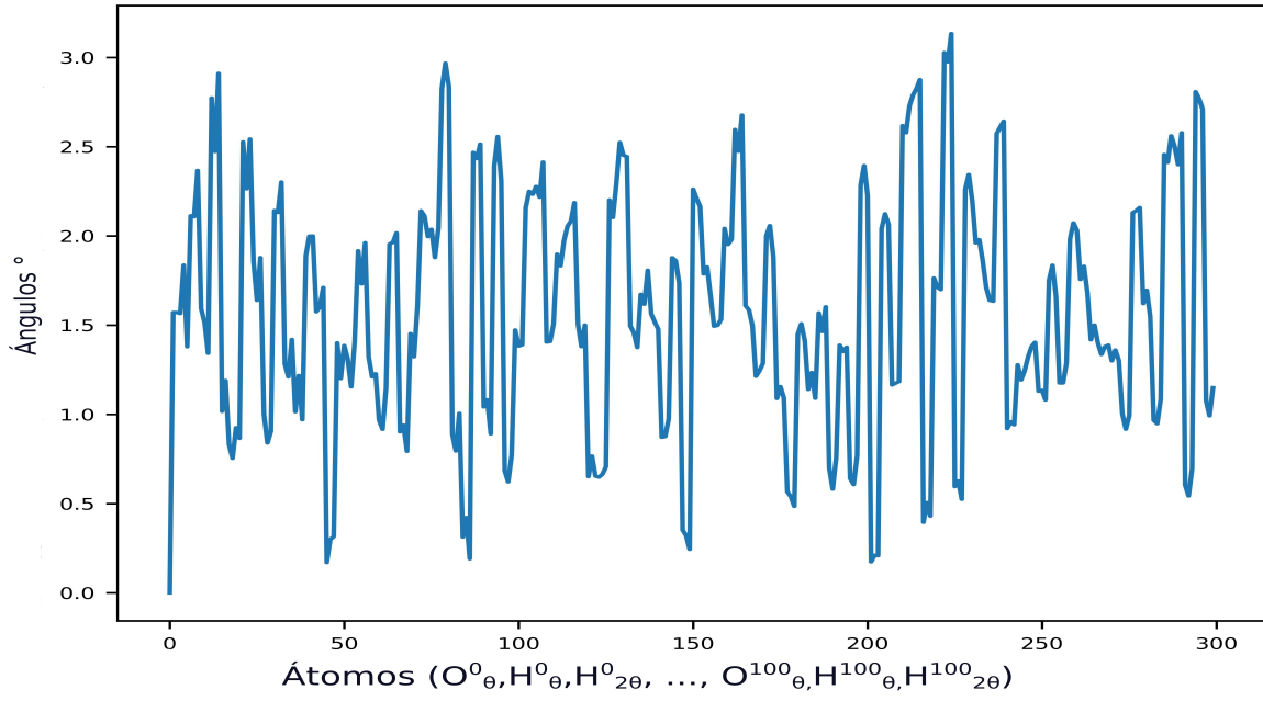
Figura 4.1.6: Distribución en \theta del primer vecindario en el cuadro de tiempo t = 0
