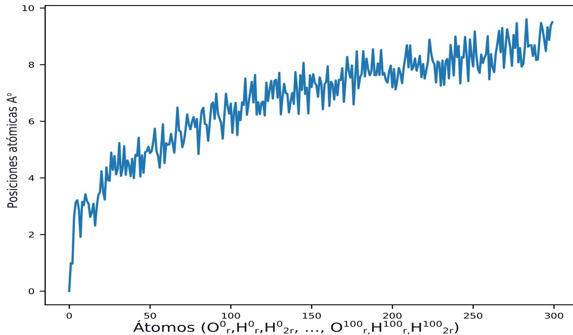
Figura 4.1.4: Distribución en r del primer vecindario en el cuadro de tiempo t = 0
