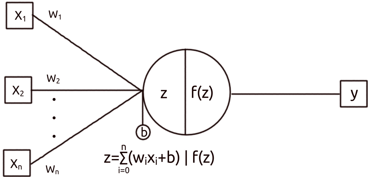
Figura 3.1.1: Representación gráfica de un perceptrón
