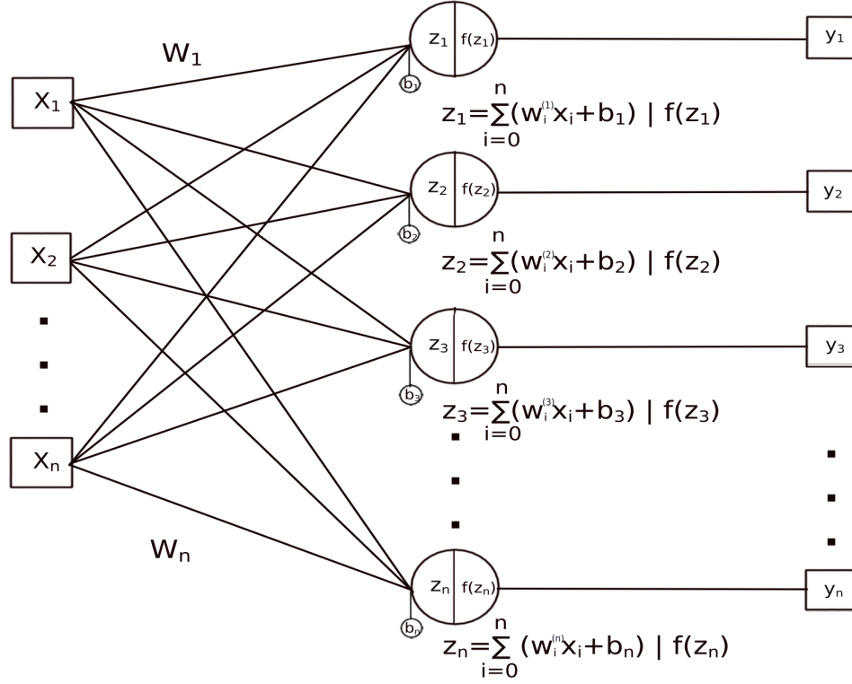
Figura 3.2.1: Representación gráfica de un perceptrón monocapa
