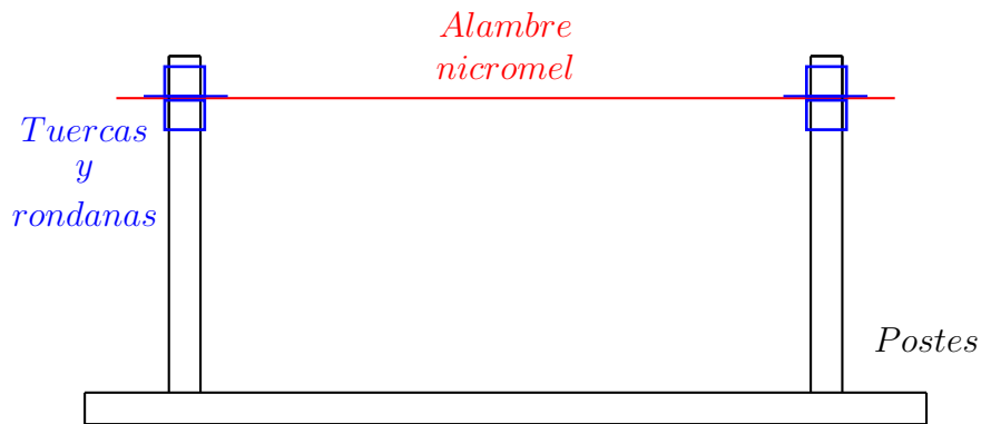
Figura 3.1: Esquema del arreglo general para producir la pluma térmica, la figura no se encuentra a escala.
