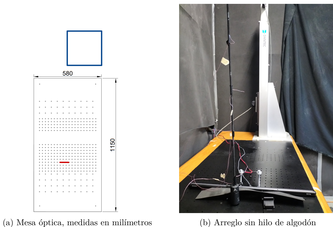
Figura 3.2: Arreglo experimental
