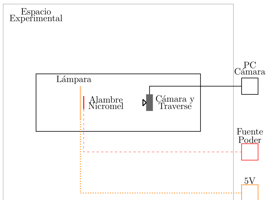
Figura 1.1: Entorno experimental, vista superior. Los componentes no están a escala.
