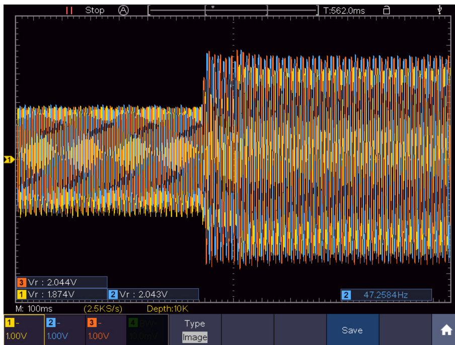
Figura 4.13: Comportamiento de las corrientes del ETM ante un cambio de carga.
