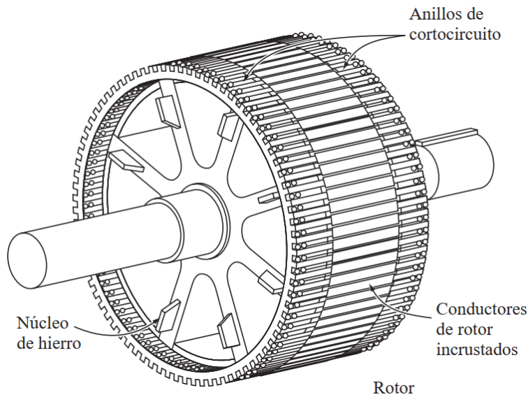
Figura 3.5: Motor jaula de ardilla. Tomado de [51].
