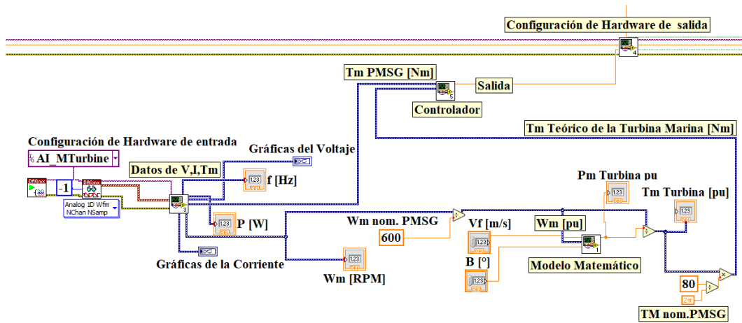
Figura 4.9: Código en LabView del sistema de emulación de turbina marina.
