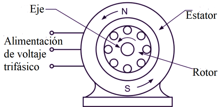
Figura 3.6: Esquema de un motor de inducción. Adaptado de [52].
