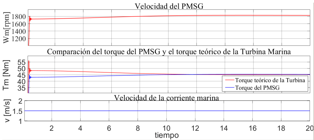
Figura 4.4: Comportamiento del sistema de emulación de turbina marina en estado estable.
