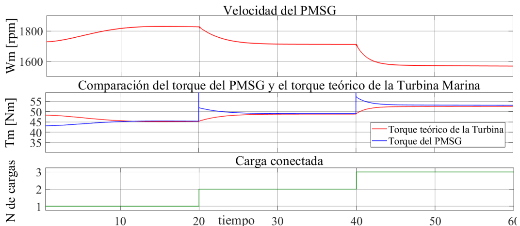
Figura 4.5: Comportamiento del sistema de emulación de turbina marina ante un cambio de carga.
