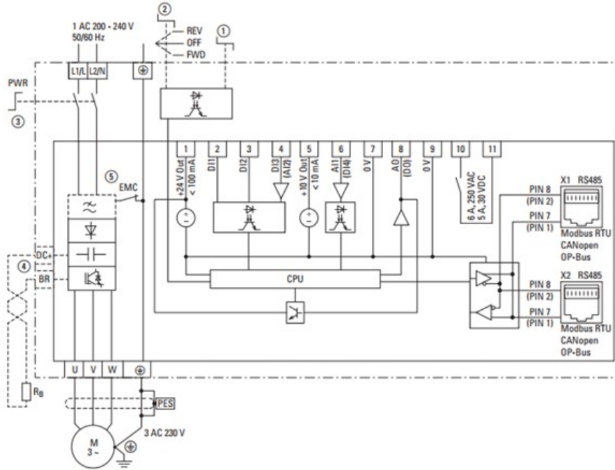
Figura 3.2: Diagrama de bloques. Variador de Frecuencia DC1-12011NB. Tomado de [50].
