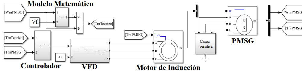
Figura 4.3: Implementación en software de la cama de pruebas del ETM.
