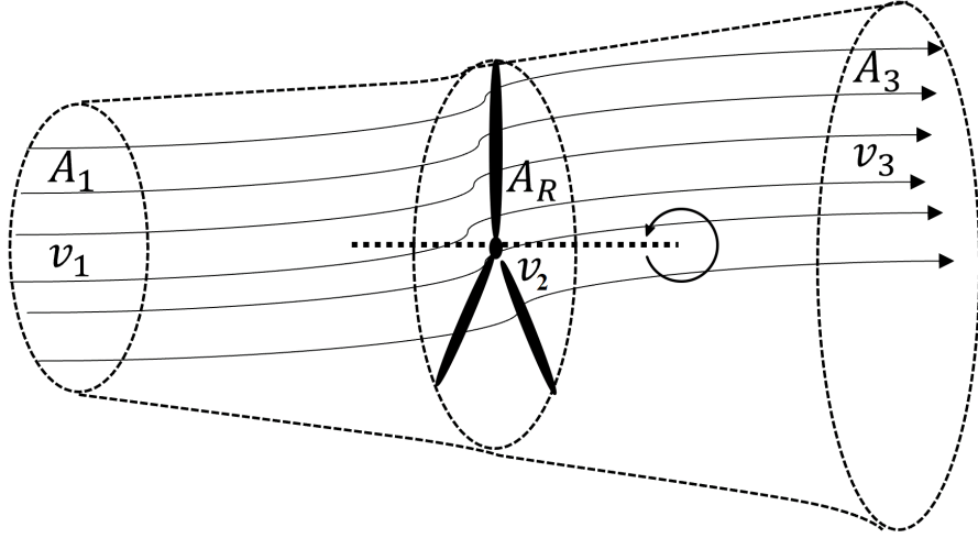
Figura 2.6: Flujo por un volumen de control.
