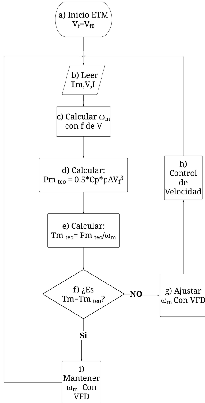
Figura 4.2: Algoritmo Sistema de emulación de Turbina Marina.
