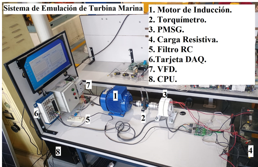
Figura 4.7: Cama de pruebas del sistema ETM.
