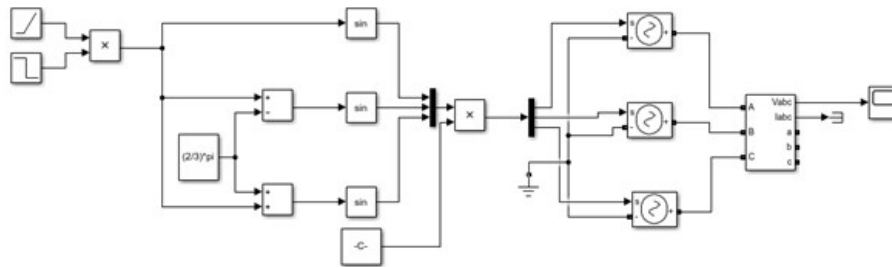
Figura 3.3: Variador de Frecuencia. Modelo Matlab/Simulink.
