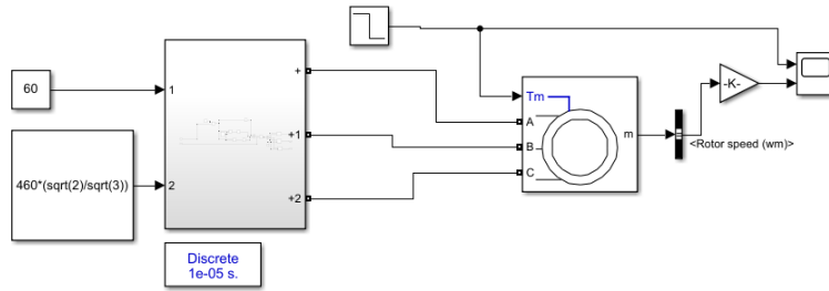
Figura 3.8: Diagrama de bloques del Motor de inducción.
