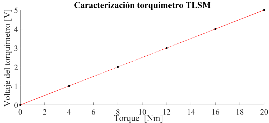
Figura 3.16: Curva característica del Torquímetro TLSM.
