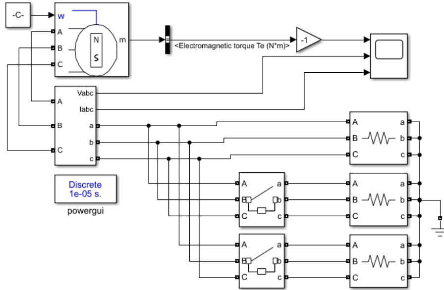
Figura 3.12: Escenario de simulación PMSG.
