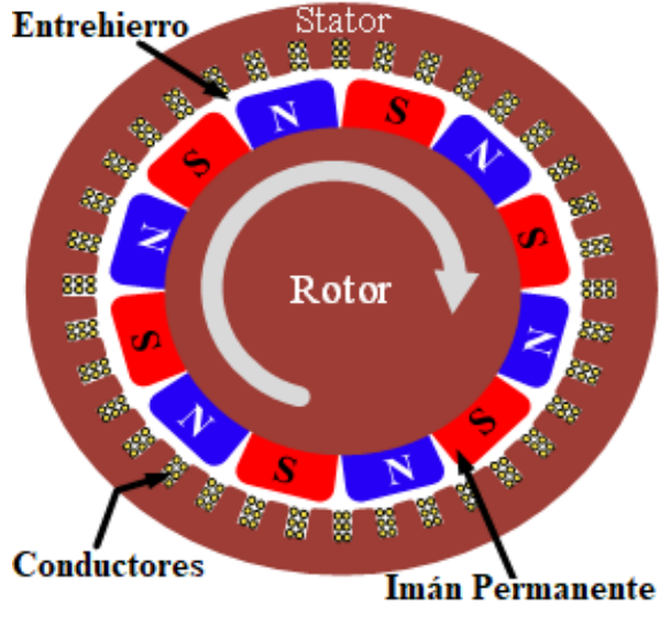
Figura 3.10: Generador síncrono de imanes permanentes.
