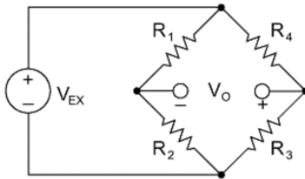
Figura 3.15: Puente de Wheatstone. Adaptado de [57].
