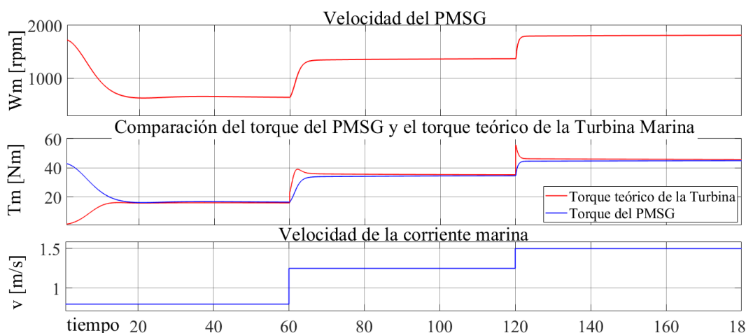
Figura 4.6: Comportamiento del sistema de emulación de turbina marina ante un cambio de velocidad.
