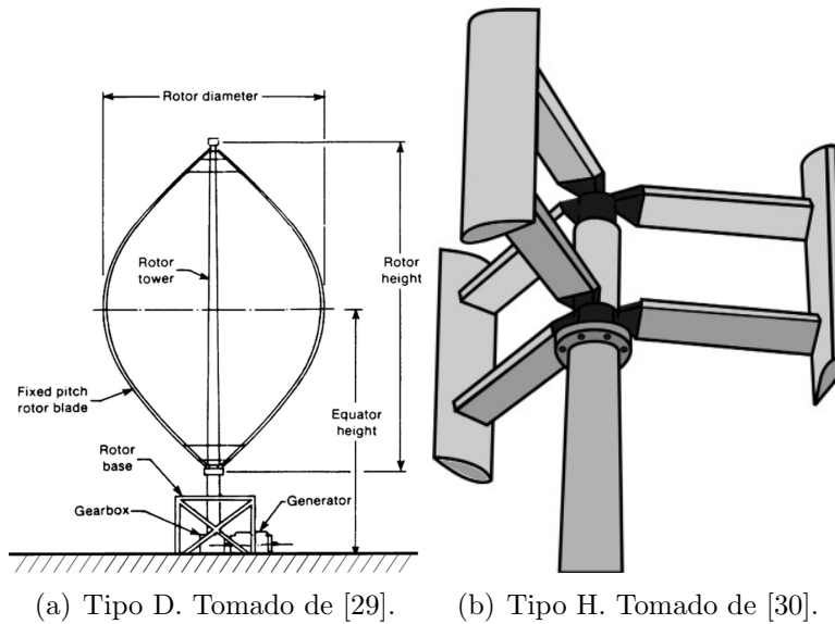
Figura 2.7: Turbinas Darrieus.
