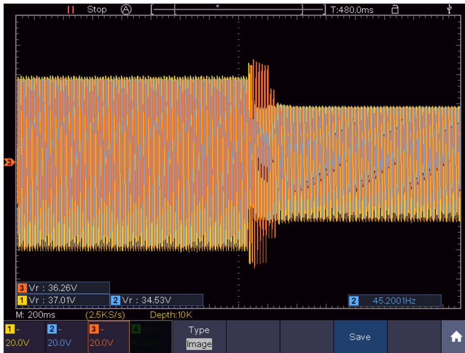
Figura 4.12: Comportamiento de los voltajes del ETM ante un cambio de carga.
