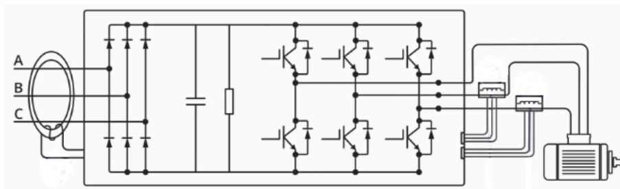
Figura 3.1: Configuración típica de un VFD. Adaptado de [49].
