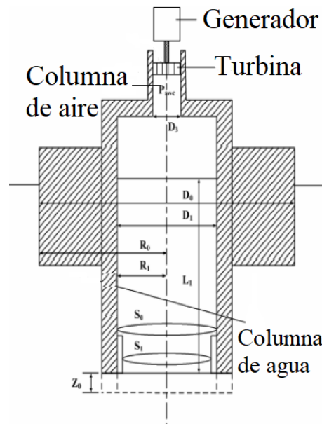
Figura 2.9: Ejemplo de Wave Energy Converter. Tomado de [35].
