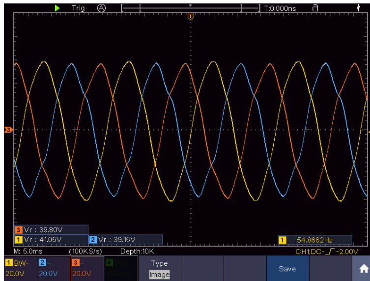
Figura 4.10: Voltaje trifásico del ETM en estado estable.
