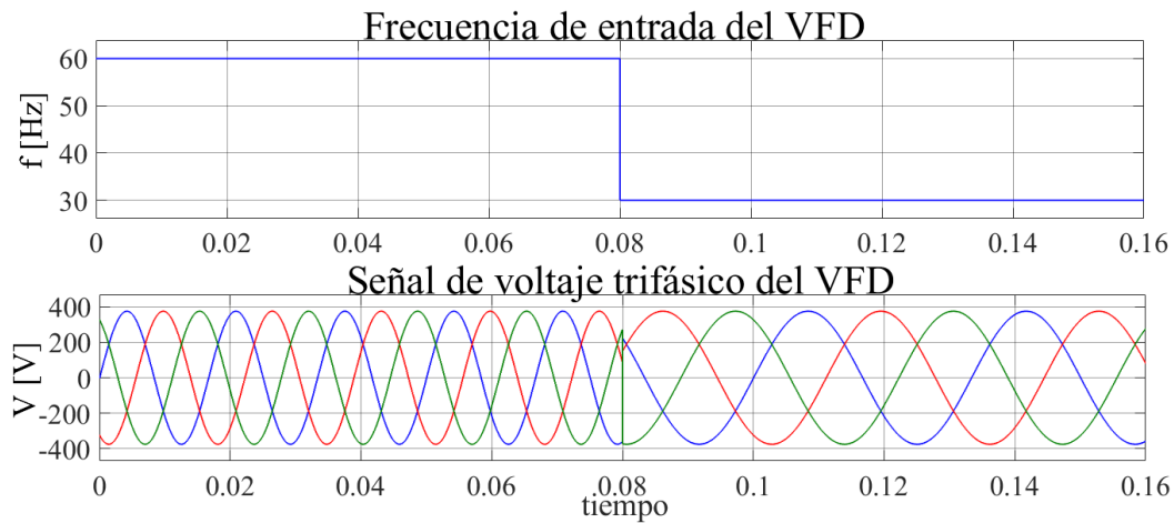
Figura 3.4: Simulación del VFD.
