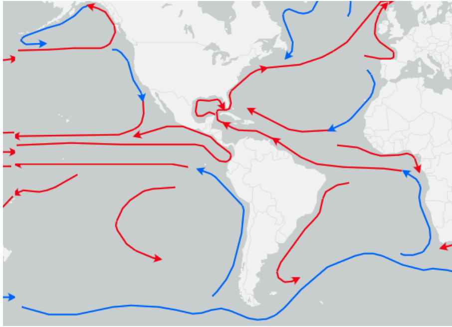
Figura 2.4: Corrientes marinas a lo largo de la Tierra. Tomado de [16].
