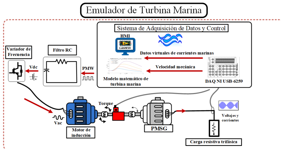
Figura 4.1: Diagrama general del sistema de emulación de turbina marina.
