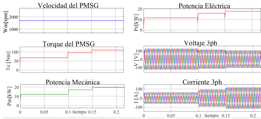
Figura 3.13: Resultados de simulación del PMSG.
