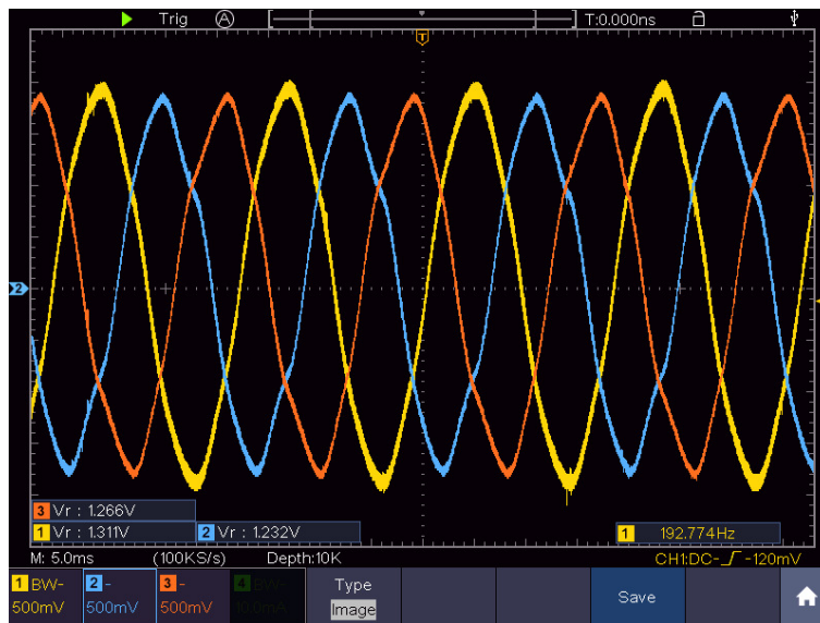
Figura 4.11: Corriente trifásica del ETM en estado estable.
