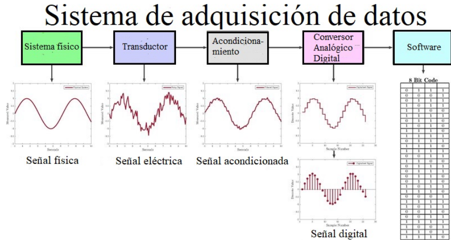
Figura 3.17: Operación de un sistema de adquisición de datos. Adaptada de [58].
