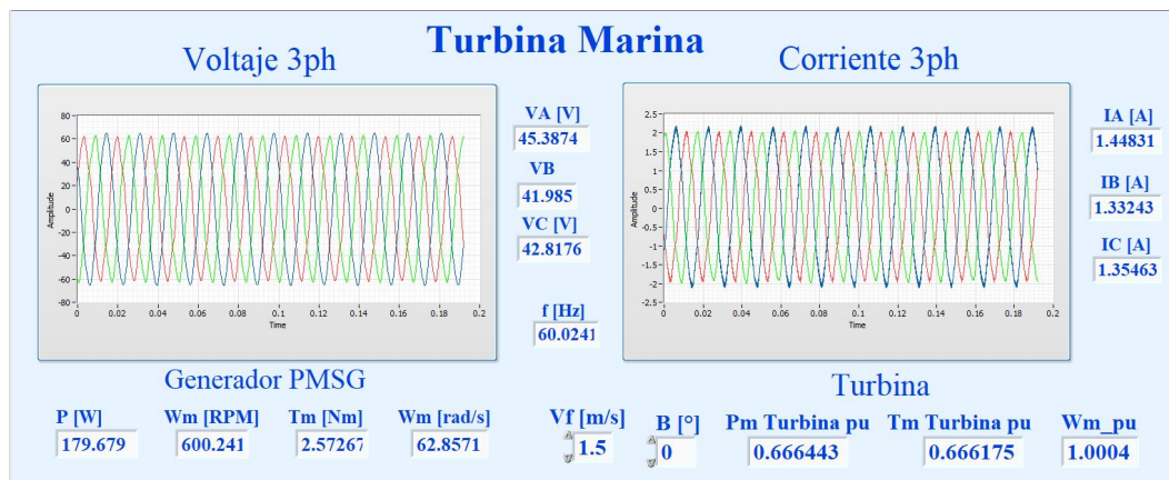
Figura 4.8: Interfaz HMI del sistema de emulación de turbina marina.
