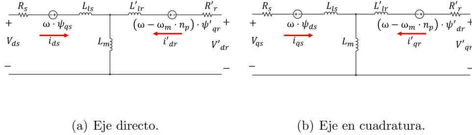
Figura 3.7: Circuito equivalente del motor de inducción.
