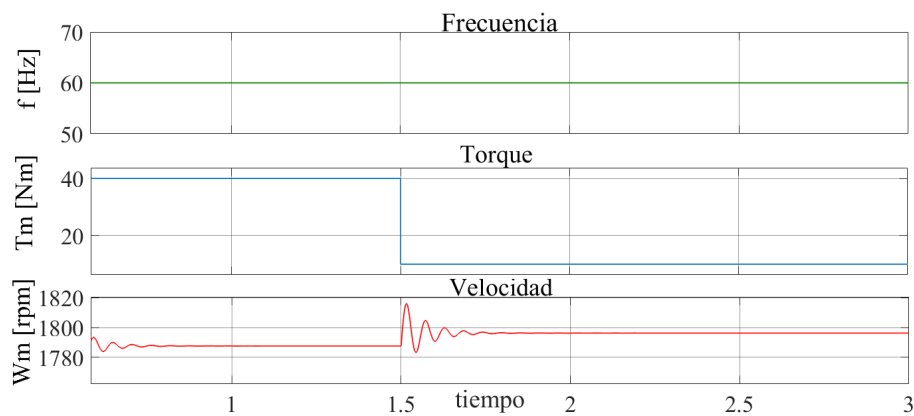
Figura 3.9: Simulación del Motor de inducción.
