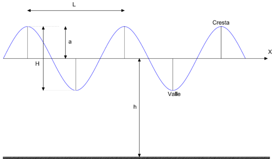
Figura 2.1: Representación de una ola marina. Tomado de [8].
