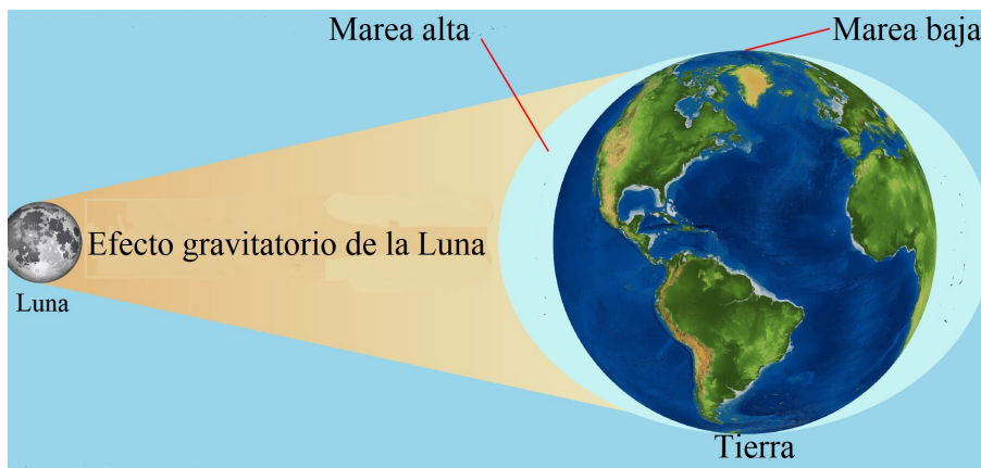
Figura 2.3: Mareas en la Tierra. Adaptado de [13].
