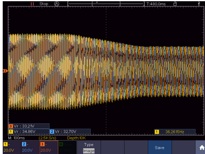
Figura 4.14: Comportamiento de los voltajes del ETM ante un cambio de velocidad.
