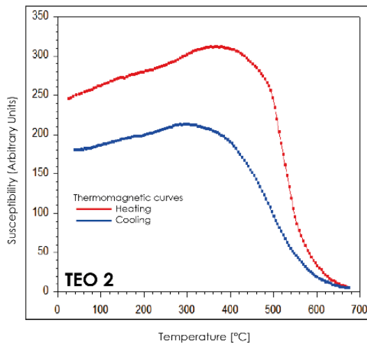
Figura 27. curvas termomagnéticas continuas de TEO 2
