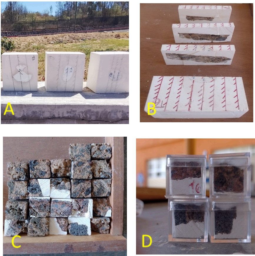
Figura 20. Muestras encapsuladas y cortadas en el laboratorio. A) Bloques de yeso secándose en el sol; B) Bloque cortado para obtener especímenes; C) Especímenes cortados pertenecientes a la muestra T6; D) Especímenes de la muestra T6 encapsuladas en cubos de acrílico
