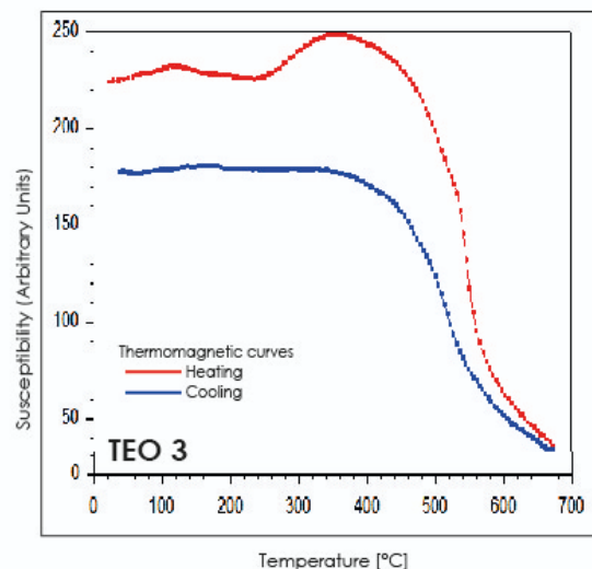
Figura 28 curvas termomagnéticas continuas de TEO 3
