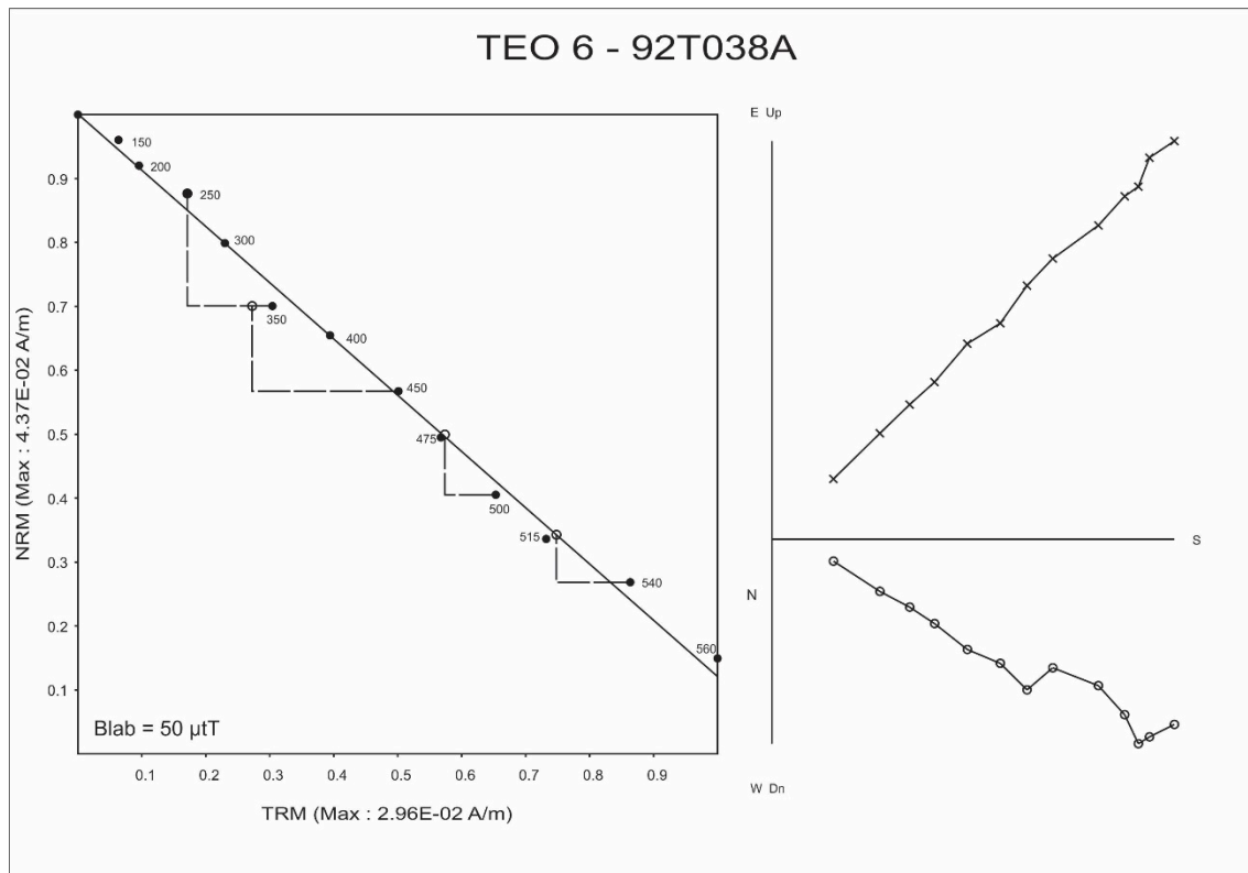
Figura 34. Especímenes 14, 23 y 38 aprobados después del experimento de paleointensidad.
