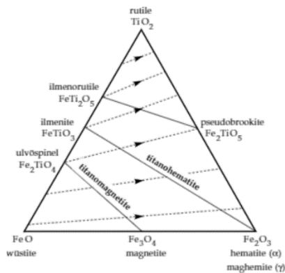
Figura 4. Diagrama ternario del grupo de minerales de óxidos de hierro y titanio (Lowrie, 2007)
