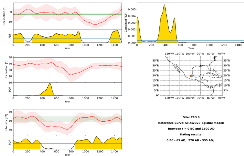
Figura 38. Datación arqueomagnética utilizando el modelo geomagnético global SHAWQ2k
