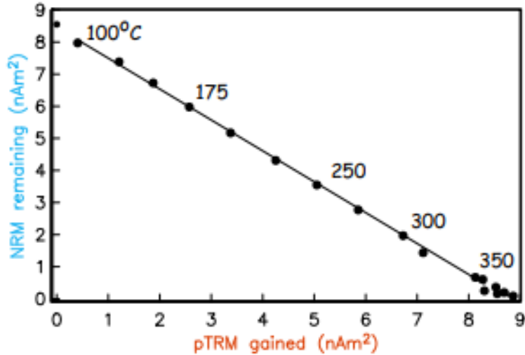
Figura 9. Grafica de Arai. pTRM vs NRM (Tauxe 2005)
