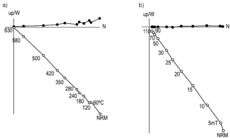
Figura 5. Diagramas de Zijderveld usando a) Desmagnetización escalonada con temperaturas crecientes y b) Desmagnetización en campos alternos crecientes en dos muestras de un horno romano en Toledo, España (Catanzariti et al., 2012)
