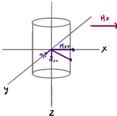
Figura 9. Tensor de anisotropía de TRM. El campo HX no solo crea magnetización en el eje x, sino que también afecta a los demás ejes (y/z) (García, 1996). Imagen: Karen Arreola Romero.
