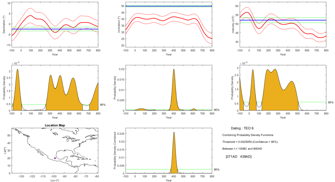
Figura 36. Datación arqueomagnética utilizando el modelo geomagnético global
