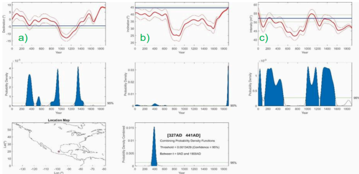
Figura 10. Datación arqueomagnética utilizando el modelo geomagnético global SHA.DIF.14k (Pavón-Carrasco et. al 2011, 2014; a) Declinación; b) Inclinação y c) Intensidad absoluta (Goguitchaichvili A. et. al., 2022)
