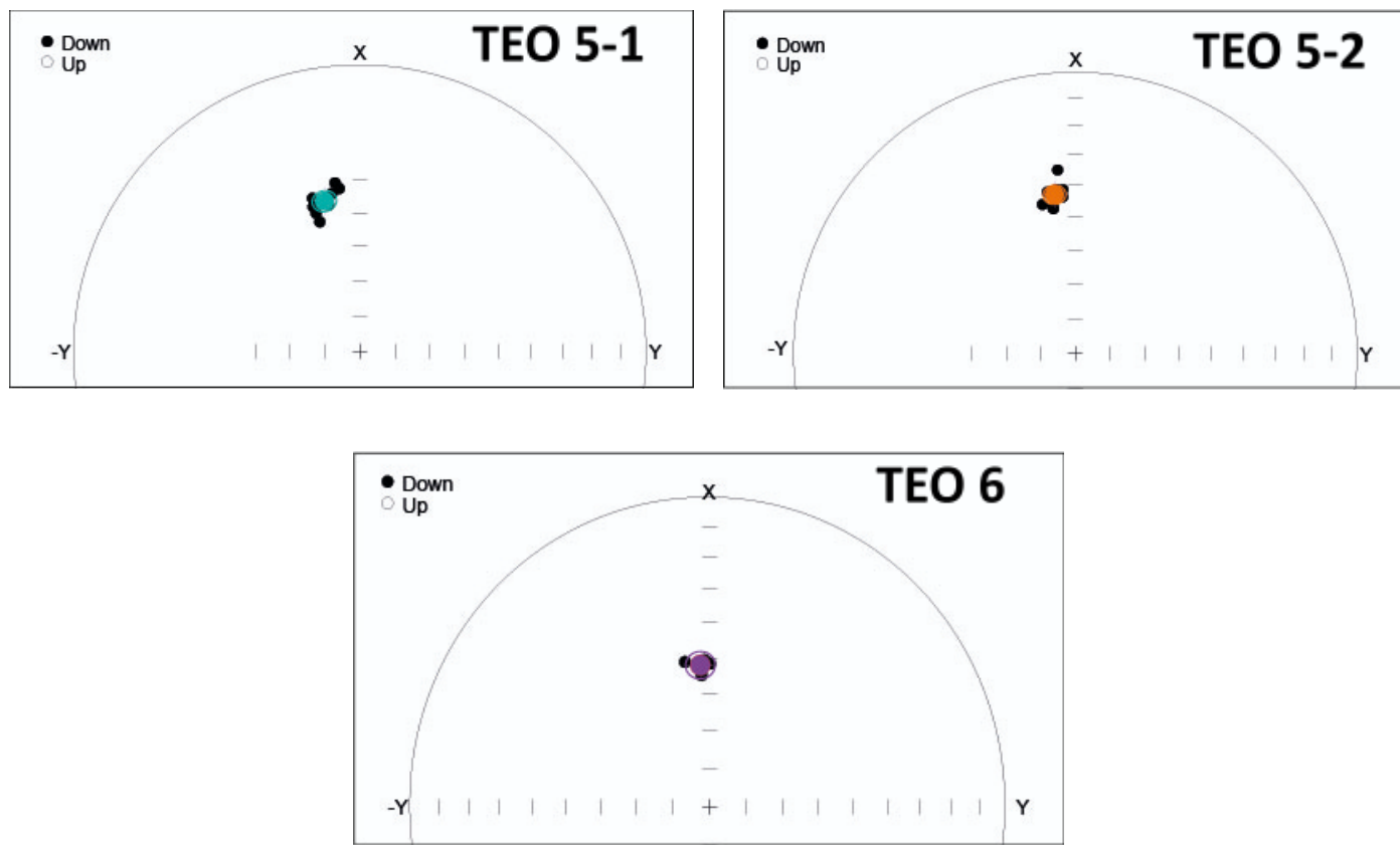
Figura 33. Esteriograma de iguales areas de las paleodirecciones pertenecientes a las muestras TEO1, TEO2, TEO3, TEO4, TEO5-1, TEO5-2, TEO6
