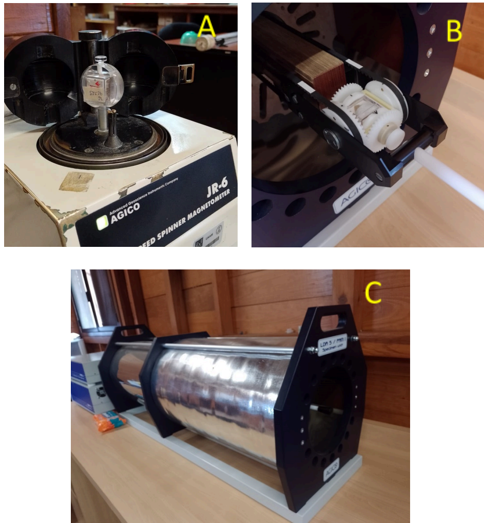
Figura 21. Experimentos de desmagnetización por campos alternos. A) la medición de la NRM usando el magnetómetro de giro AGICO JR6a; B) Muestra prepara para el experimento de desmagnetización; C) Desmagnetizador LDA5
