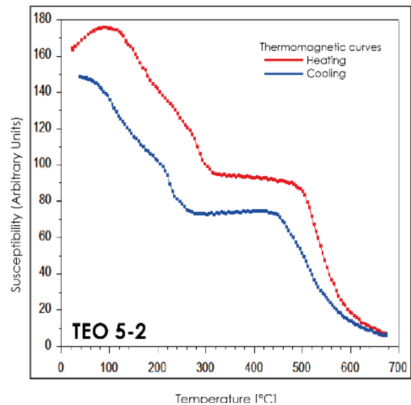
Figura 30. curvas termomagnéticas continuas de TEO 5-2
