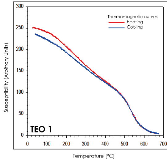
Figura 26. curvas termomagnéticas continuas de TEO 1
