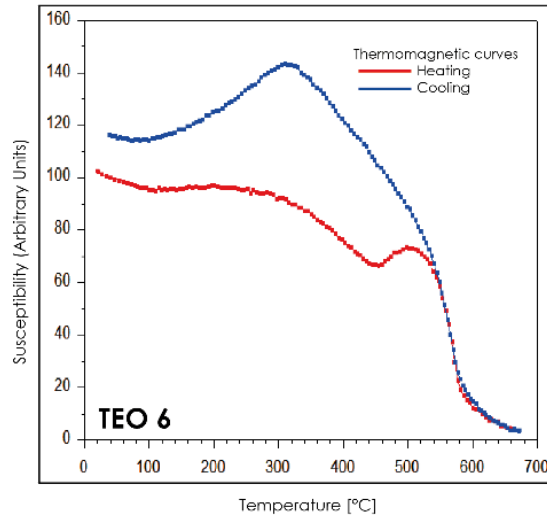
Figura 31. curvas termomagnéticas continuas de TEO 6
