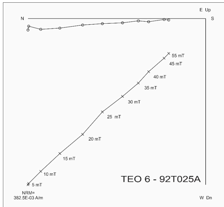
Figura 32. diagrama de Zijderveld representativos obtenidos durante los tratamientos de desmagnetización progresiva de campo alterno. La NRM indica el valor inicial de la magnetización en A/m y también se indica el valor del campo aplicado en cada paso en mT.
