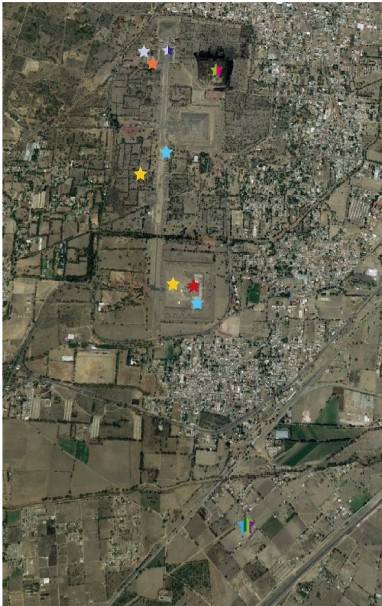
Figura 1. zonas de muestreo de los diferentes estudios arqueomagnéticos en Teotihuacán. Autor: Karen Arreola Romero
