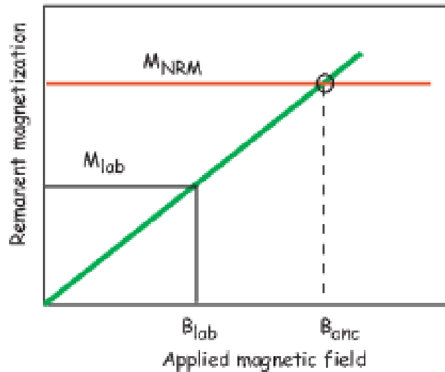
Figura 6. Principios de estimación de paleointensidad. (Tauxe 2005)
