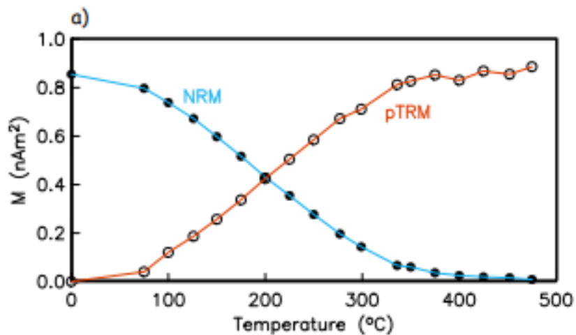
Figura 7. Ilustración del método Thellier-Thellier para determinar la paleointensidad absoluta (Tauxe 2005)
