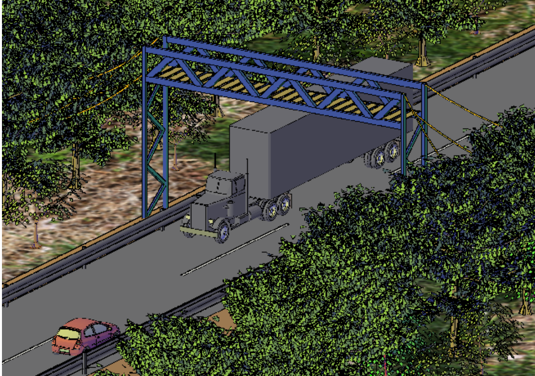
Figura 21 Paso para fauna arborícola a base de estructura metálica con tablonces de madera
