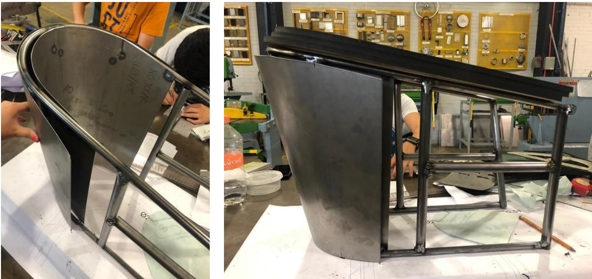
Figura 34. Manufactura del contenedor.
