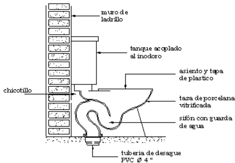
Figura 15. Estructura de un sanitario convencional. (Eddie, 2010)
