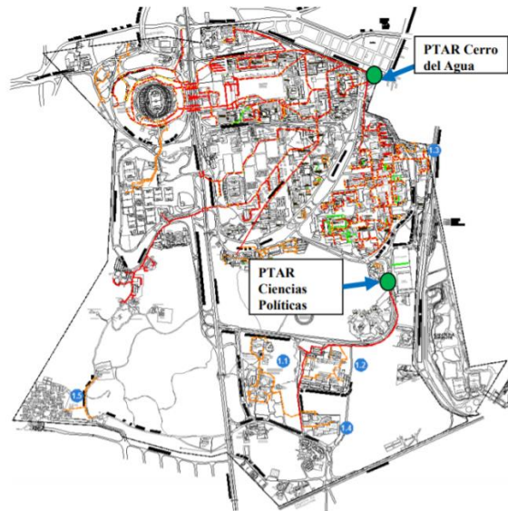
Figura 11. Sistema de drenaje 2018 (Rocha, 2018)
