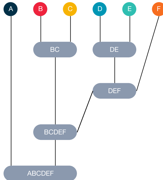
Fig. 4.3. Ejemplo de dendrograma asociado al agrupamiento jerárquico.
