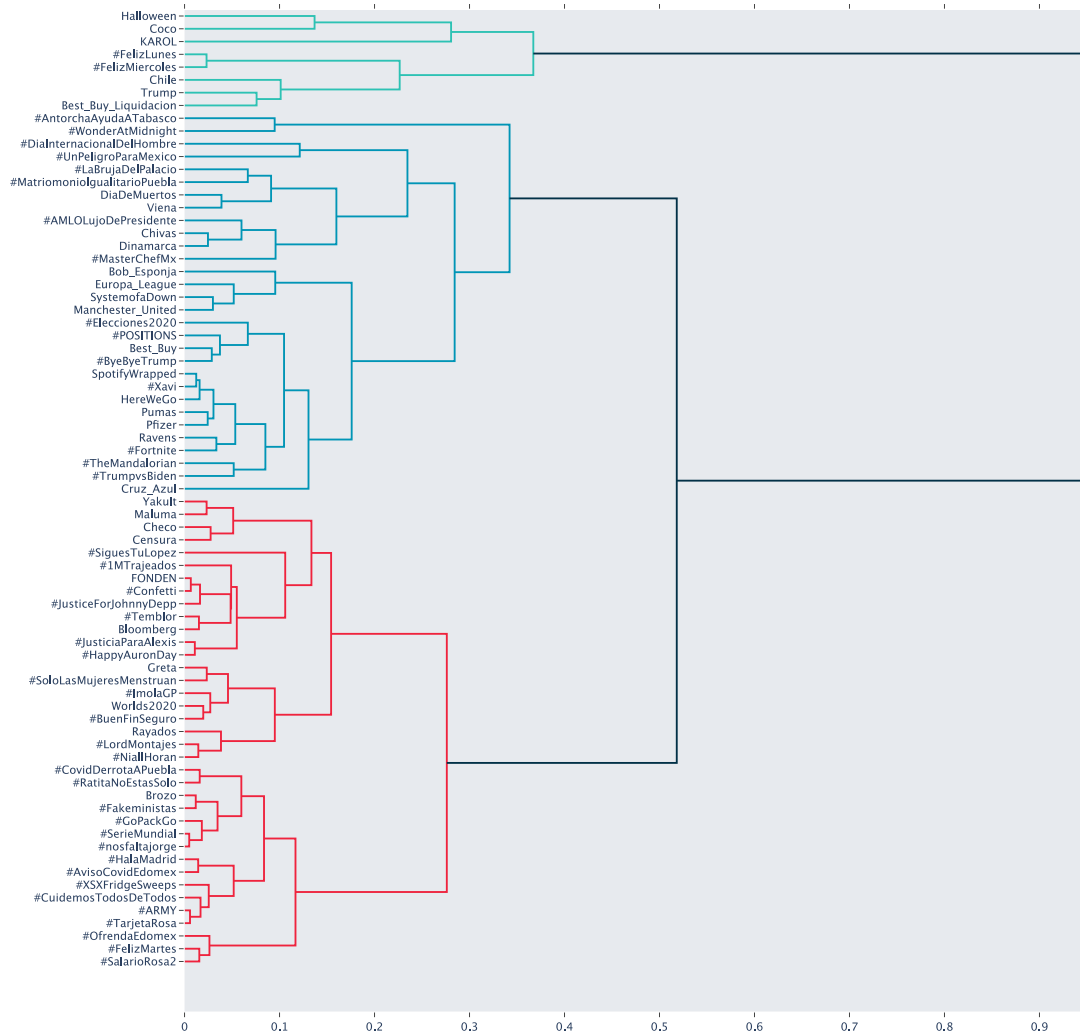
Fig. 5.6. Agrupamiento jerárquico utilizando complete linkage
