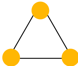
Fig. 2.1. Grafo no dirigido de tres nodos y tres aristas.
