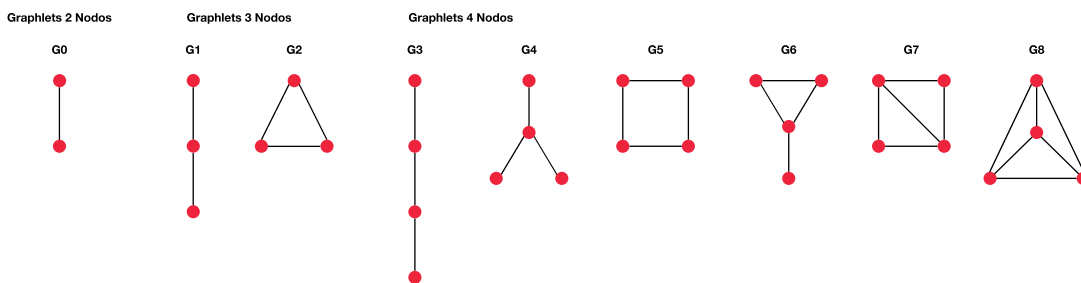
Fig. 3.1. Graphlets de 2, 3 y 4 nodos.
