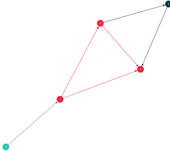
Fig. 3.4. Grafo dirigido de 5 nodos.
