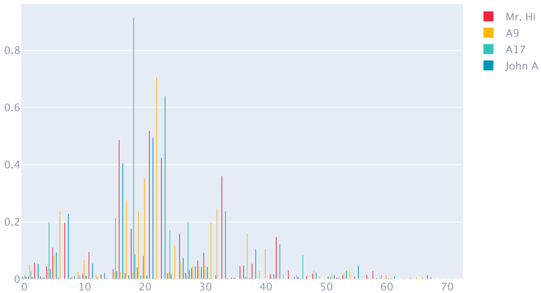
Fig. 3.7. Comparación del conteo de órbitas normalizado para 4 usuarios de la red Karate Club .
