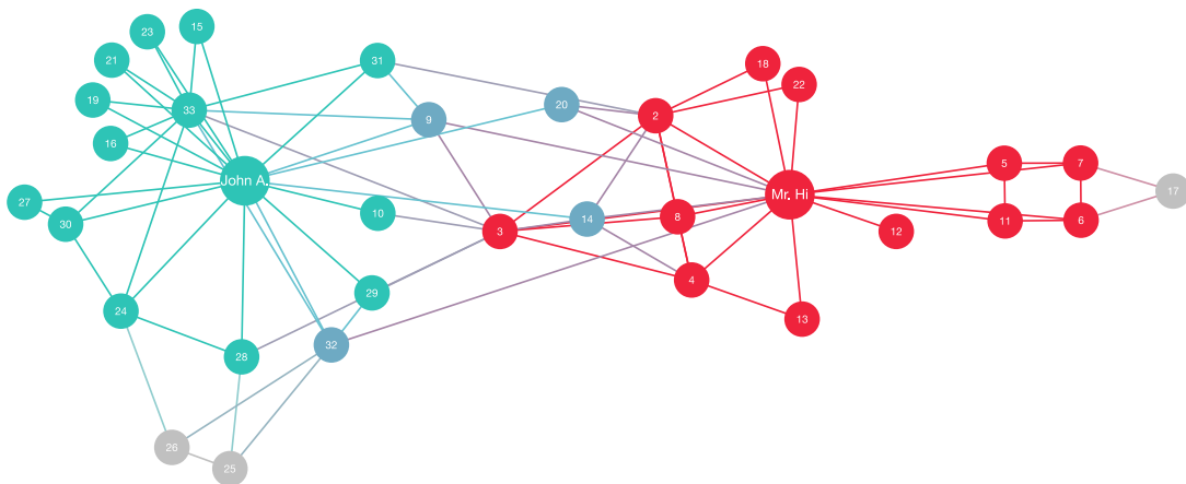
Fig. 3.6. Red de Karate Club [Zac77]. Los nodos más influyentes, Mr. Hi, John A. y sus respectivos vecinos a distancia 1 han sido coloreados.
