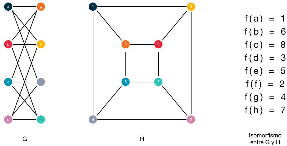
Fig. 2.3. Ejemplo de Isomorfismo entre G y H
