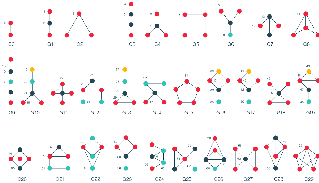
Fig. 3.3. Graphlets y órbitas no dirigidas de 2 a 5 nodos.
