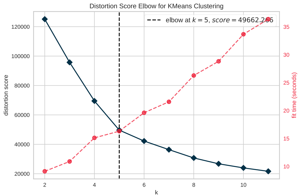
Fig. 5.1. Método Elbow o Codo para determinar el tamaño de K
