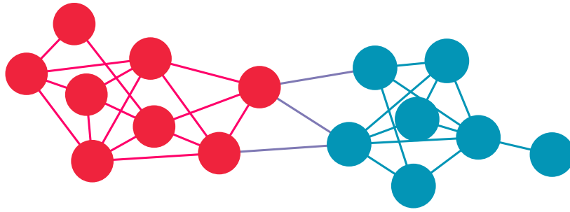
Fig. 2.6. Nodos de una red divididos en 2 grupos donde el color del nodo representa el grupo al que pertenece.
