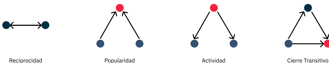
Fig. 4.2. Algunos patrones propuestos por Lusher y Robins para describir configuraciones sociales dentro de procesos colectivos [Lus]. Las aristas dirigidas permiten la distinción entre jerarquías y posiciones de poder dentro de la red.
