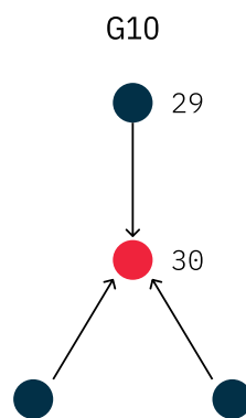
Fig. 5.13. Graphlet 10 y órbitas 29 y 30.
