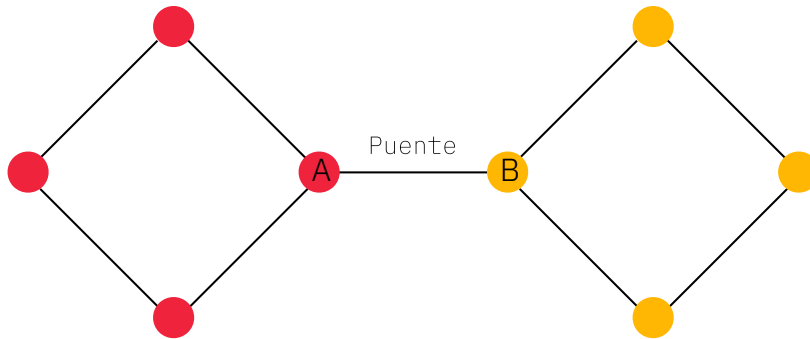
Fig. 1.3. En un grafo se conoce como puente a los nodos que conectan dos grupos, estos nodos tienen una alta intermediación ya que necesariamente por ellos pasan los caminos más cortos entre nodos de ambos grupos.
