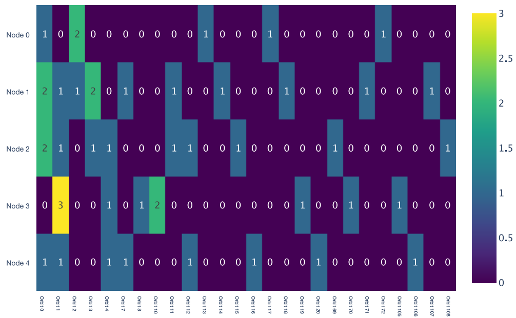
Fig. 3.5. Matriz de conteo de órbitas para el grafo 3.4
