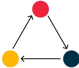
Fig. 2.2. Grafo Dirigido ( DiGraph ). Podemos observar que la dirección de las aristas esta representada por una flecha que indica en donde se origina la arista (inicio de la flecha).
