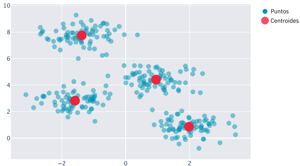
Fig. 2.5. Centroides.
