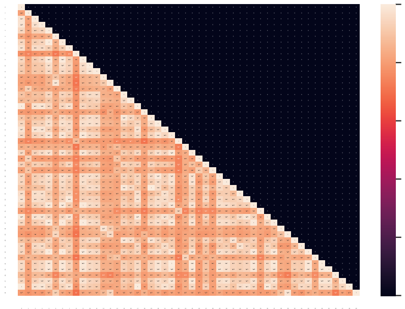
Fig. 5.2. Exploración de la estabilidad del agrupamiento que se obtiene usando KMeans y K = 5 . En este ejercicio se calculó la Información Mutua Normalizada entre distintas ejecuciones del algoritmo.
