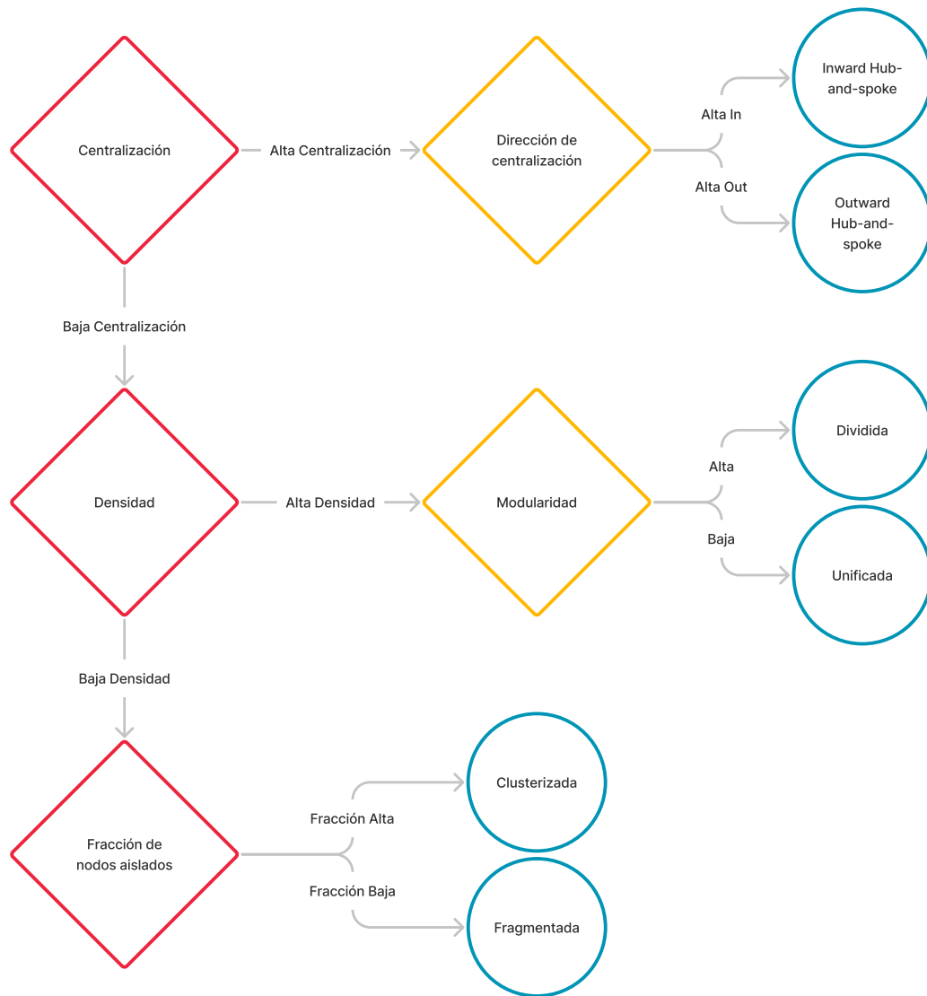
Fig. 1.1. Árbol de decisión para clasificar redes temáticas en Twitter, propuesto por Himelboim et al. [Him+17]
