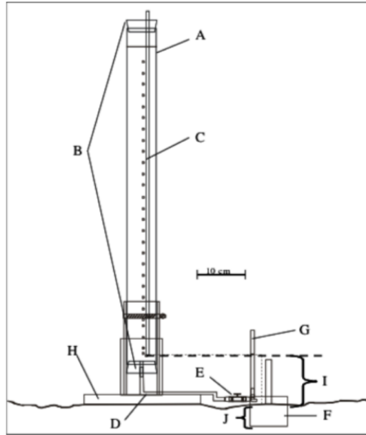
Figura 14. Esquema del infiltrómetro de carga constante y anillo sello. Tomado de Gómez-Tagle (2008)
