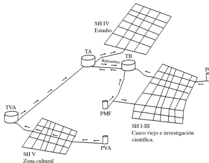
Figura 11. Esquema de distribución entre pozos y tanques en CU. Adaptado de Rocha (2010)
