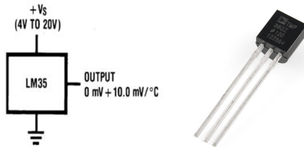
(a) Diagrama Esquemático del (b) Sensor de temperatura de la Sensor serie LM45. serie LM45 comercial.
