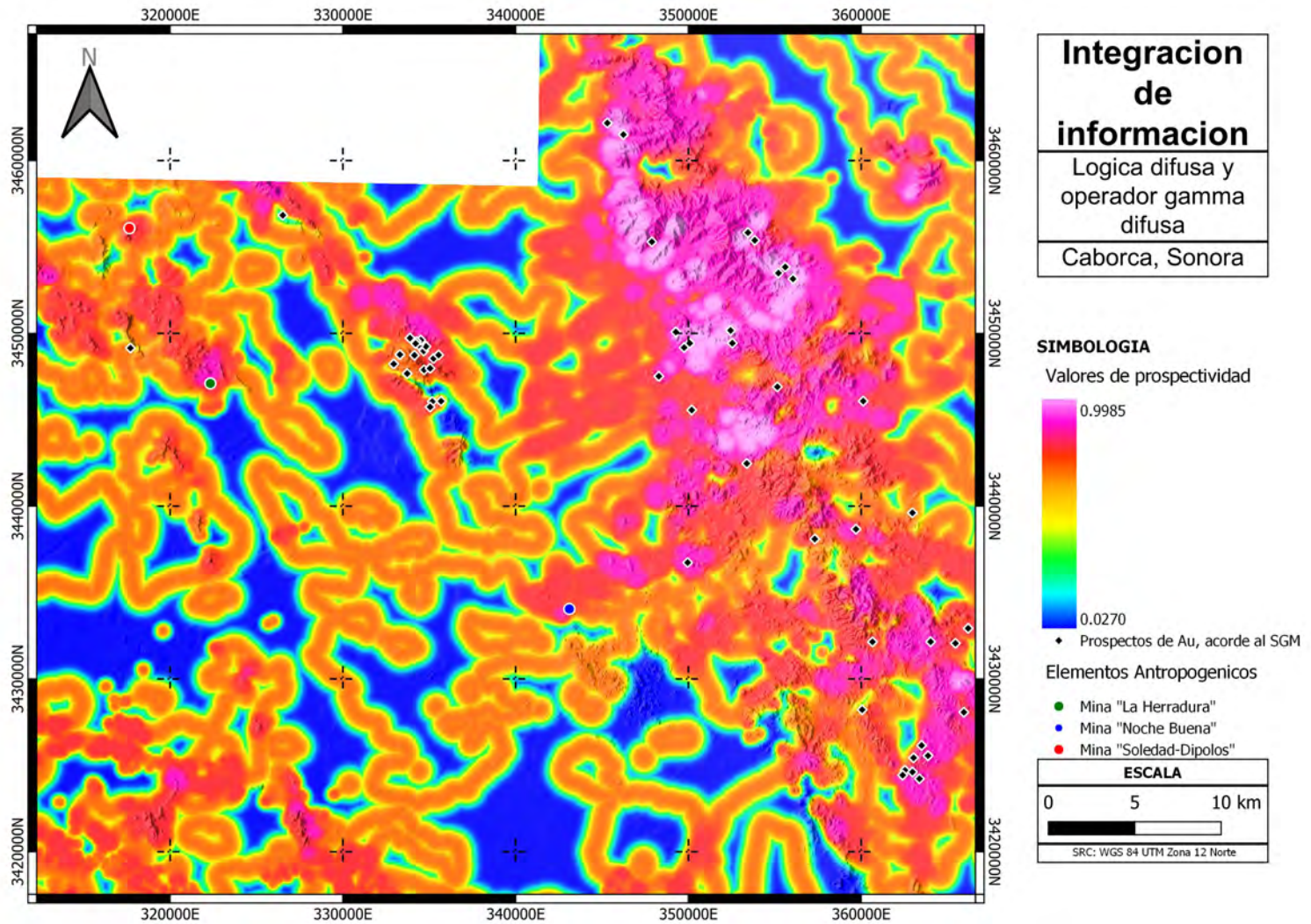
Figura 49: Mapa resultante del motor de inferencia con el operador gamma difusa.
