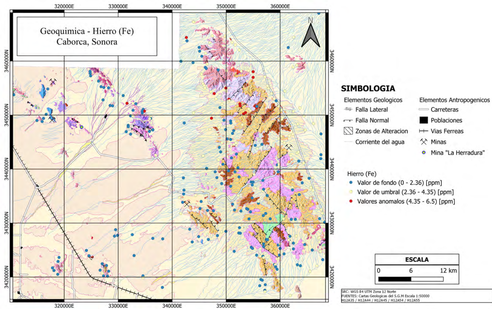
Figura 35: Mapa de la distribución del Hierro en los sedimentos de arroyo del área de estudio.
