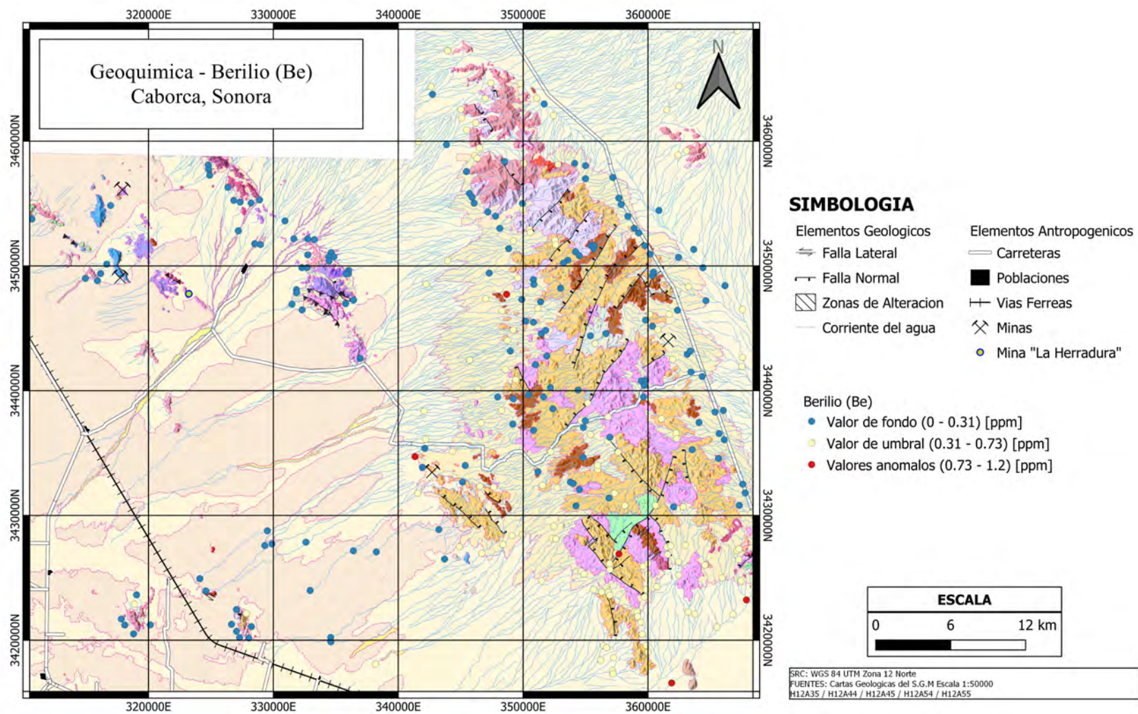
Figura 33: Mapa de la distribución del Berilio en los sedimentos de arroyo del área de estudio.
