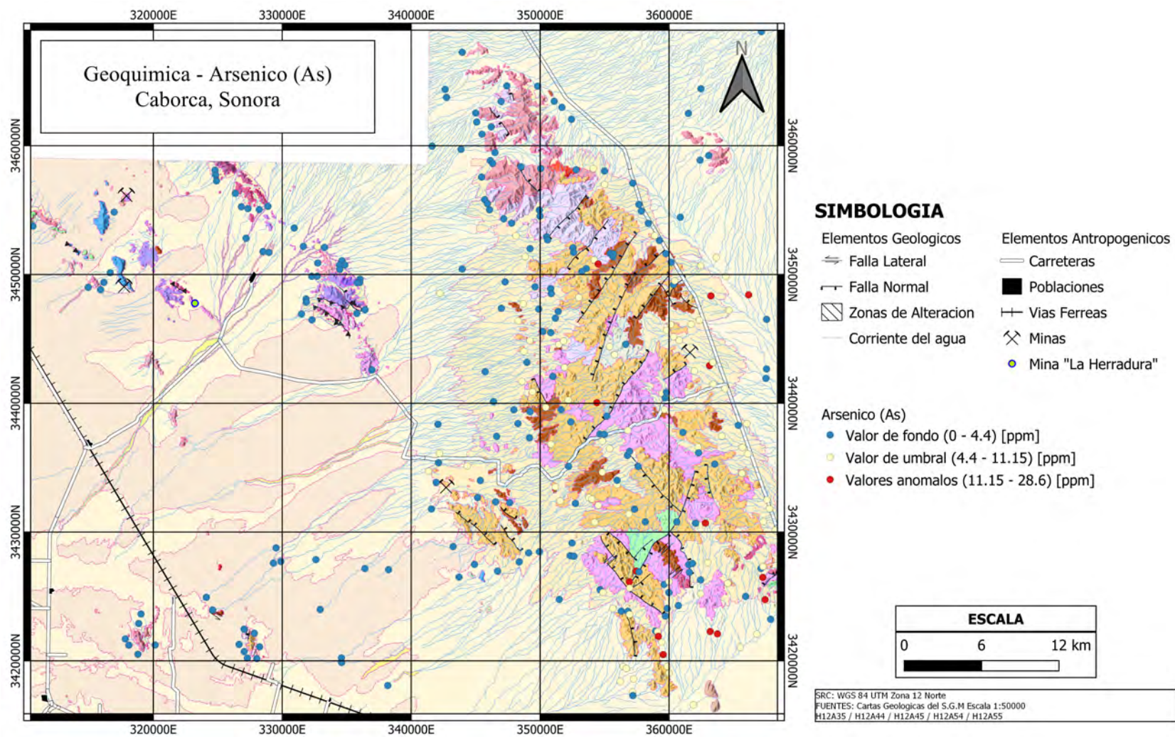
Figura 31: Mapa de la distribución del Arsénico en los sedimentos de arroyo del área de estudio.
