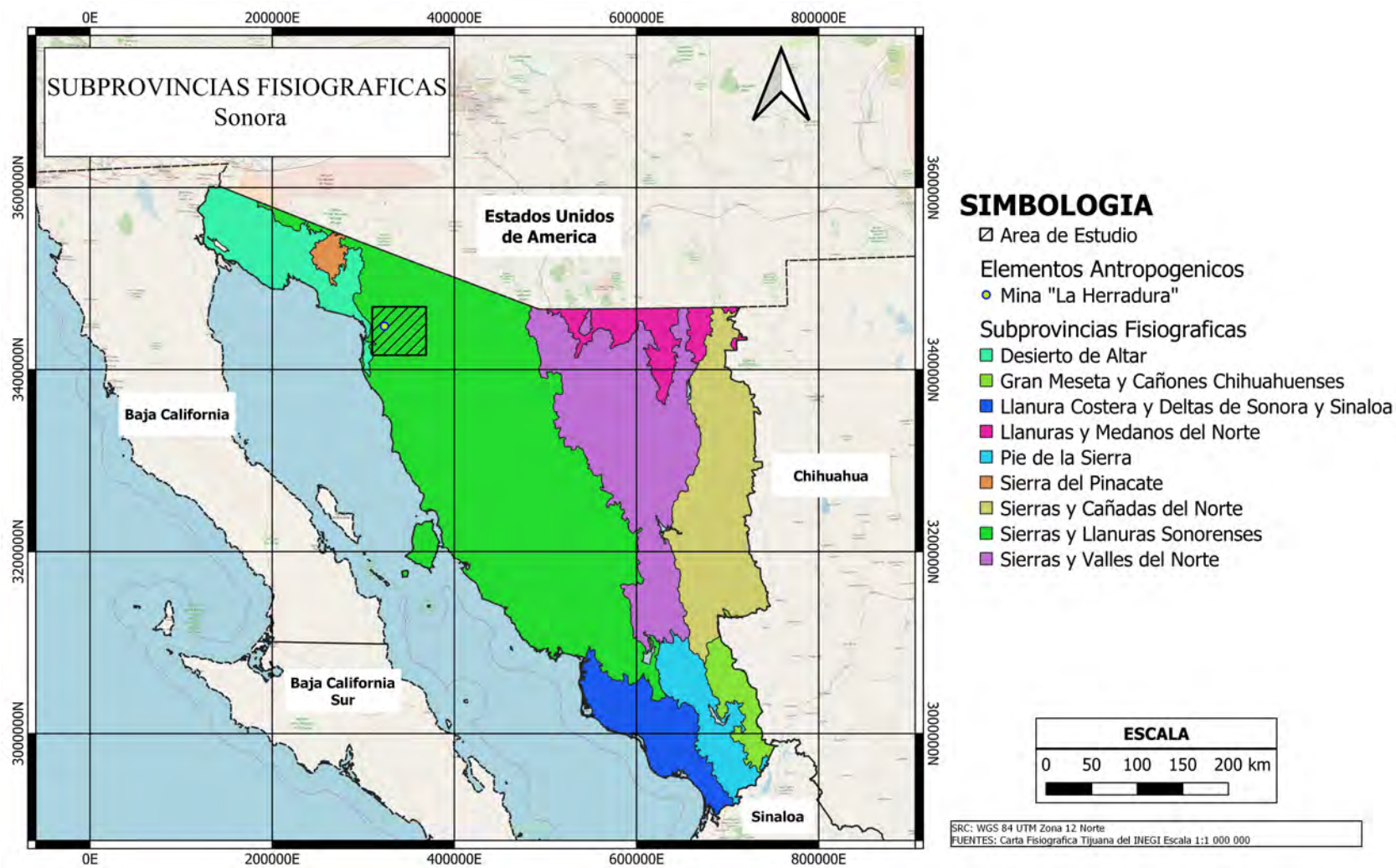
Figura 11: Subprovincias fisiográficas del estado de Sonora con la ubicación del área de estudio.
