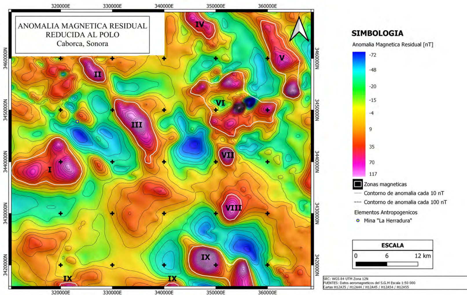
Figura 25: Anomalia magnética residual reducida al polo con la identificación de zonas magnéticas.
