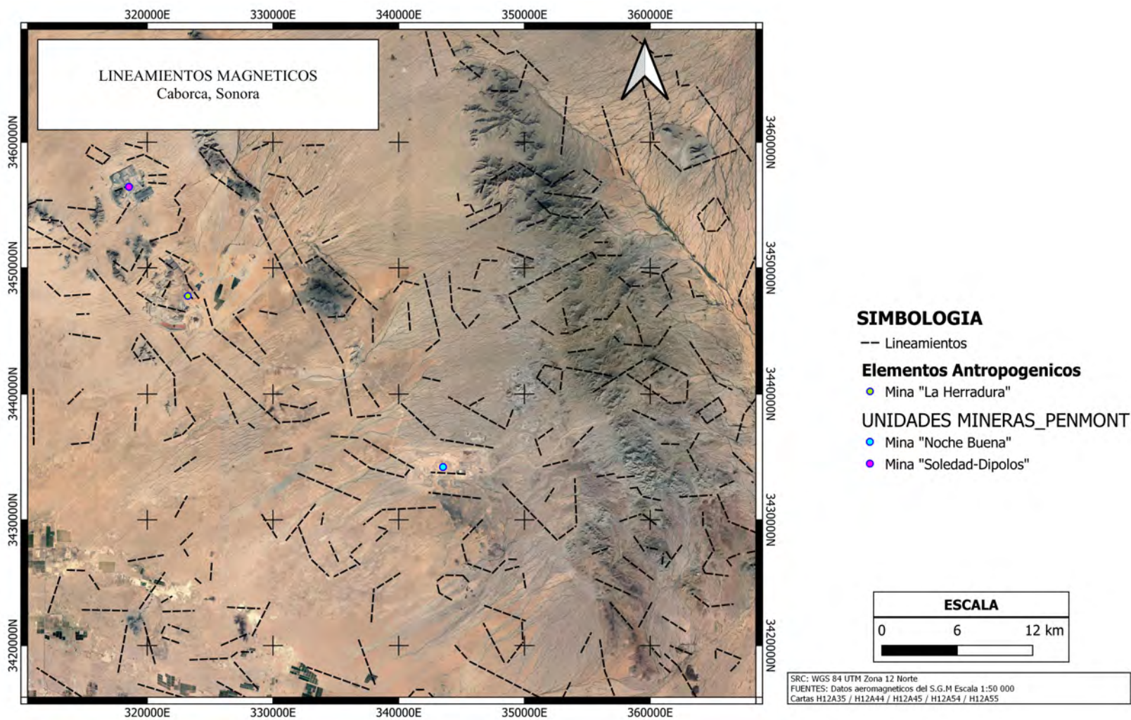
Figura 29: Lineamientos magnéticos identificados con el método de FSED.
