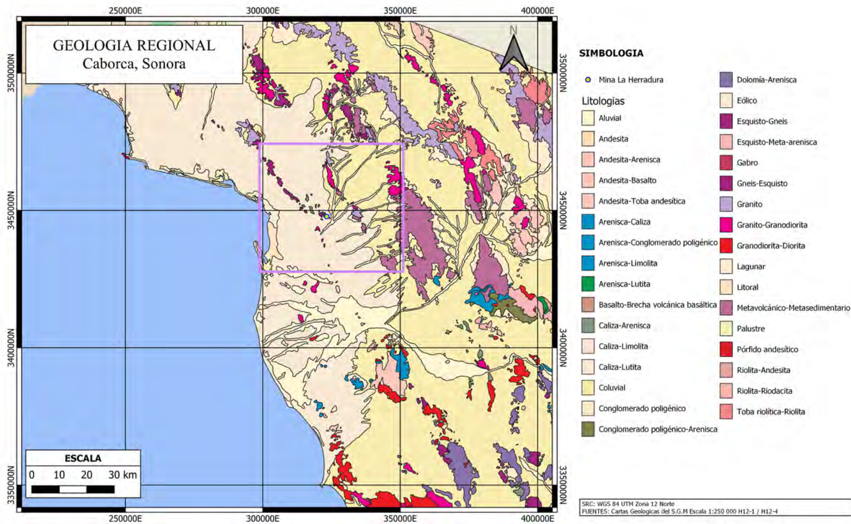
Figura 14: Mapa geológico regional del NW de México.
