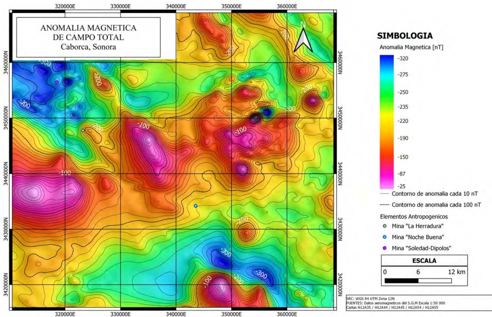
Figura 22: Anomalia magnética de campo total.
