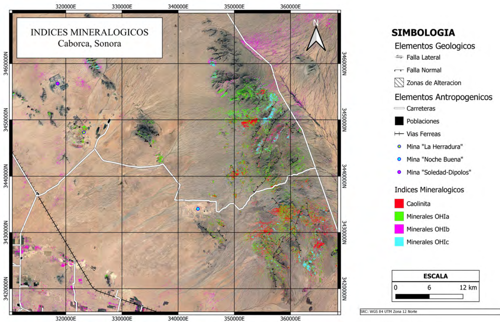
Figura 44: Identificación de minerales de interés mediante índices mineralógicos.
