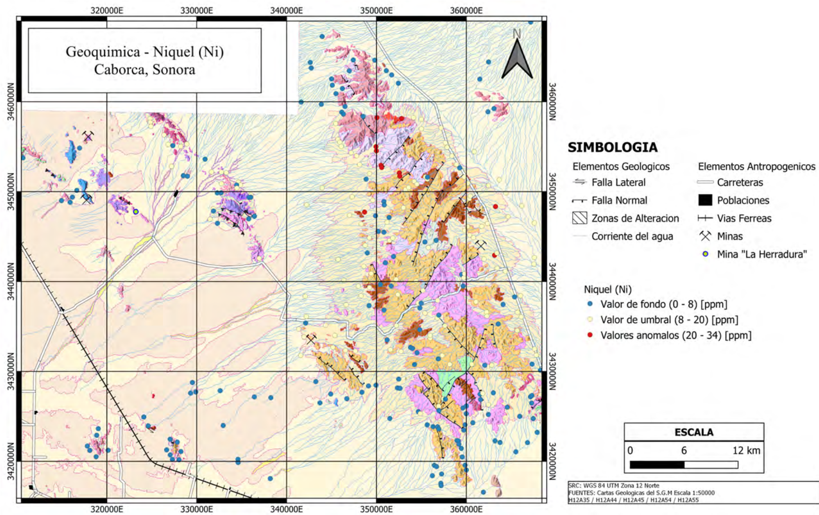
Figura 38: Mapa de la distribución del Níquel en los sedimentos de arroyo del área de estudio.
