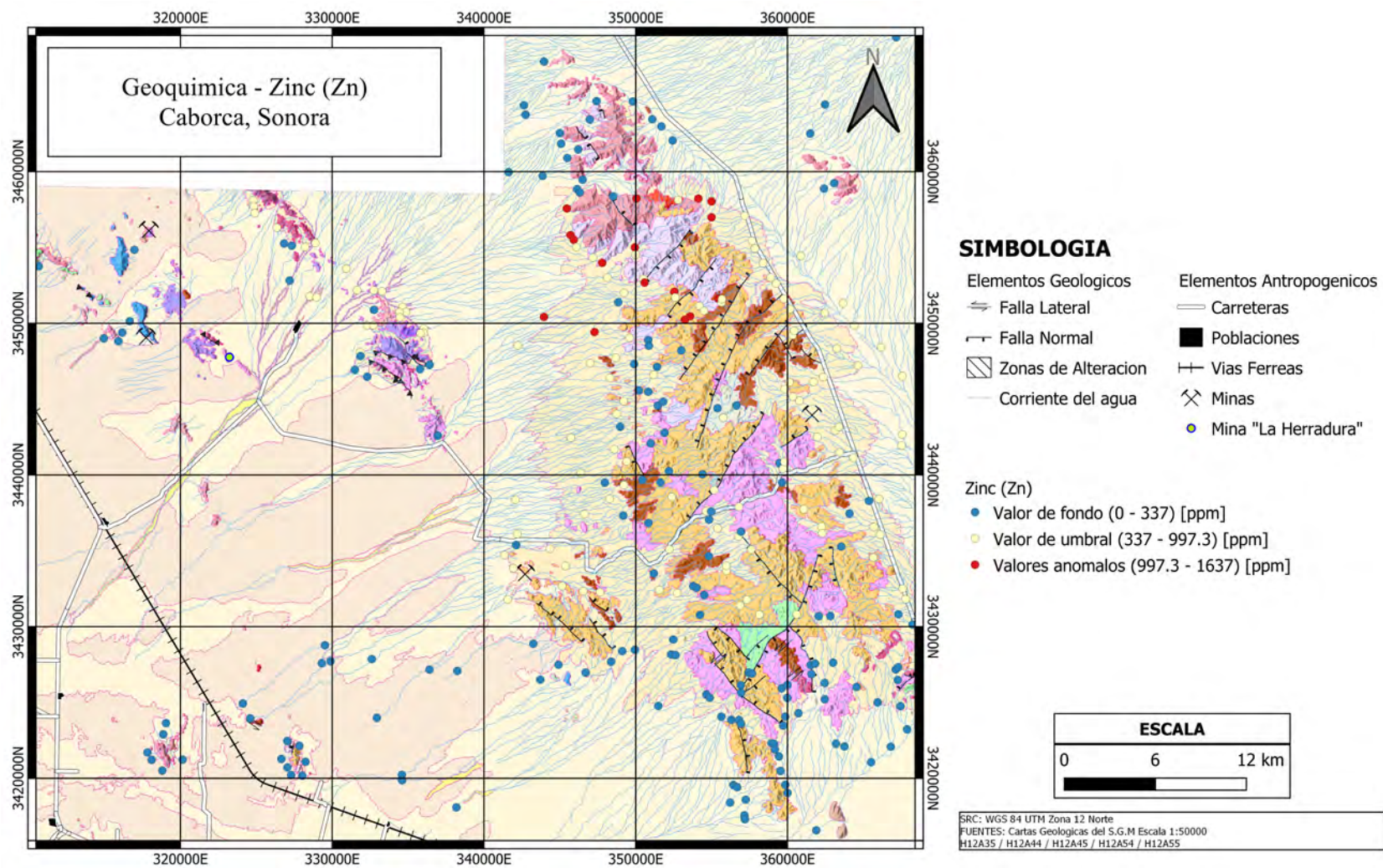
Figura 41: Mapa de la distribución del Zinc en los sedimentos de arroyo del área de estudio.
