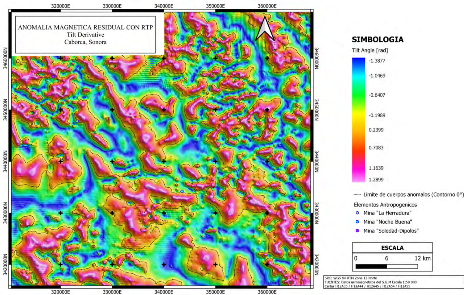
Figura 26: Derivada de Tilt (Tilt derivative) de la anomalía magnética residual reducida al polo.
