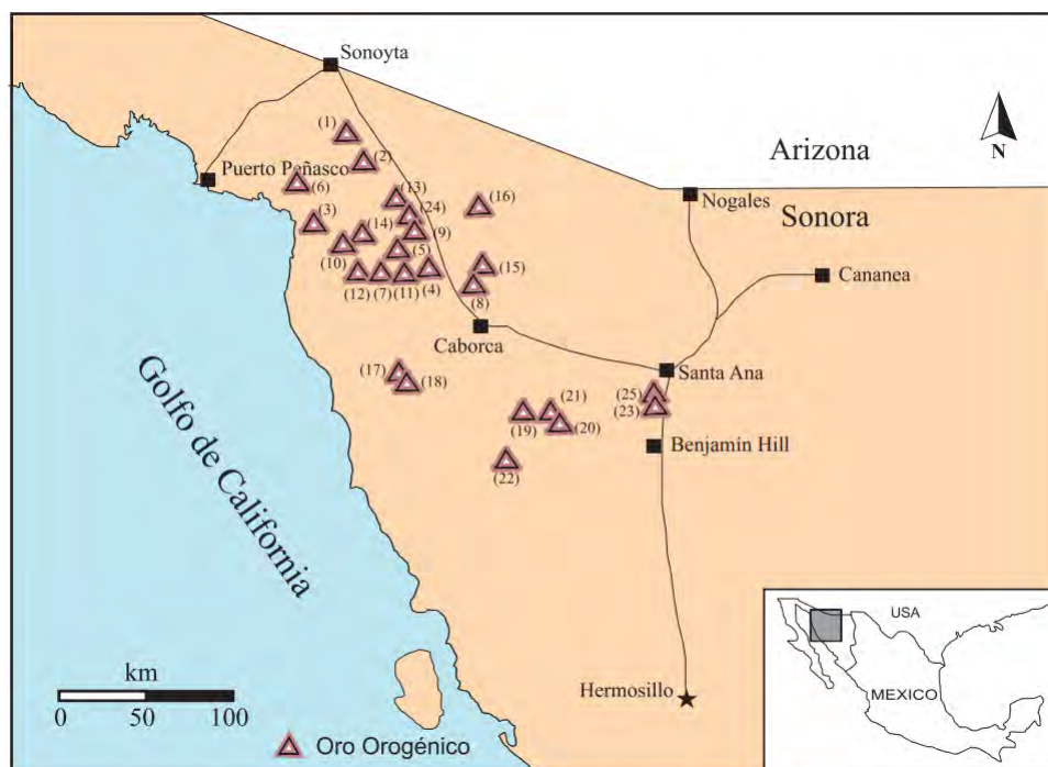
Figura 20: Ubicación aproximada de depósitos de oro orogénico al norte-noroeste del estado de Sonora. (1) Quitovac, (2) La Choya, (3) La Herradura, (4) Tajitos, (5) Juárez-San Francisco, (6) Sierra Pinta, (7) San Francisco, (8) El Chanate, (9) Cinco Hermanos, (10) Noche Buena, (11) Mexico Nuevo, (12) La Coronela, (13) La Union, (14) Carina, (15) La Joya, (16) San Miguel, (17) San Felix, (18) Veta Amarilla, (19) El Argonauta, (20) El Tiro, (21) El Boludo, (22) La Cienega, (23) San Francisco-Estacion Llano, (24) Banco de oro, (25) La Chicharra. (Ochoa Landin et al., 2011).
