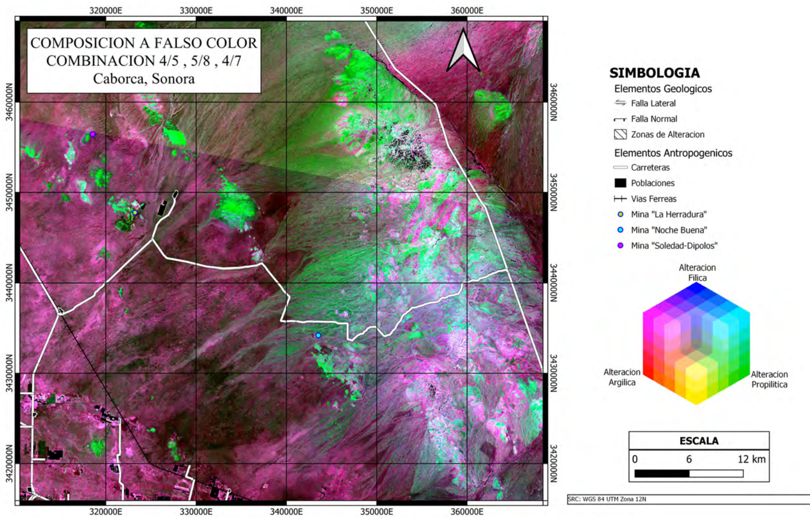
Figura 42: Composición a falso color con la alteración argílica en el rojo (R), la alteración propilítica en el verde (G) y la alteración filica en el azul (B).
