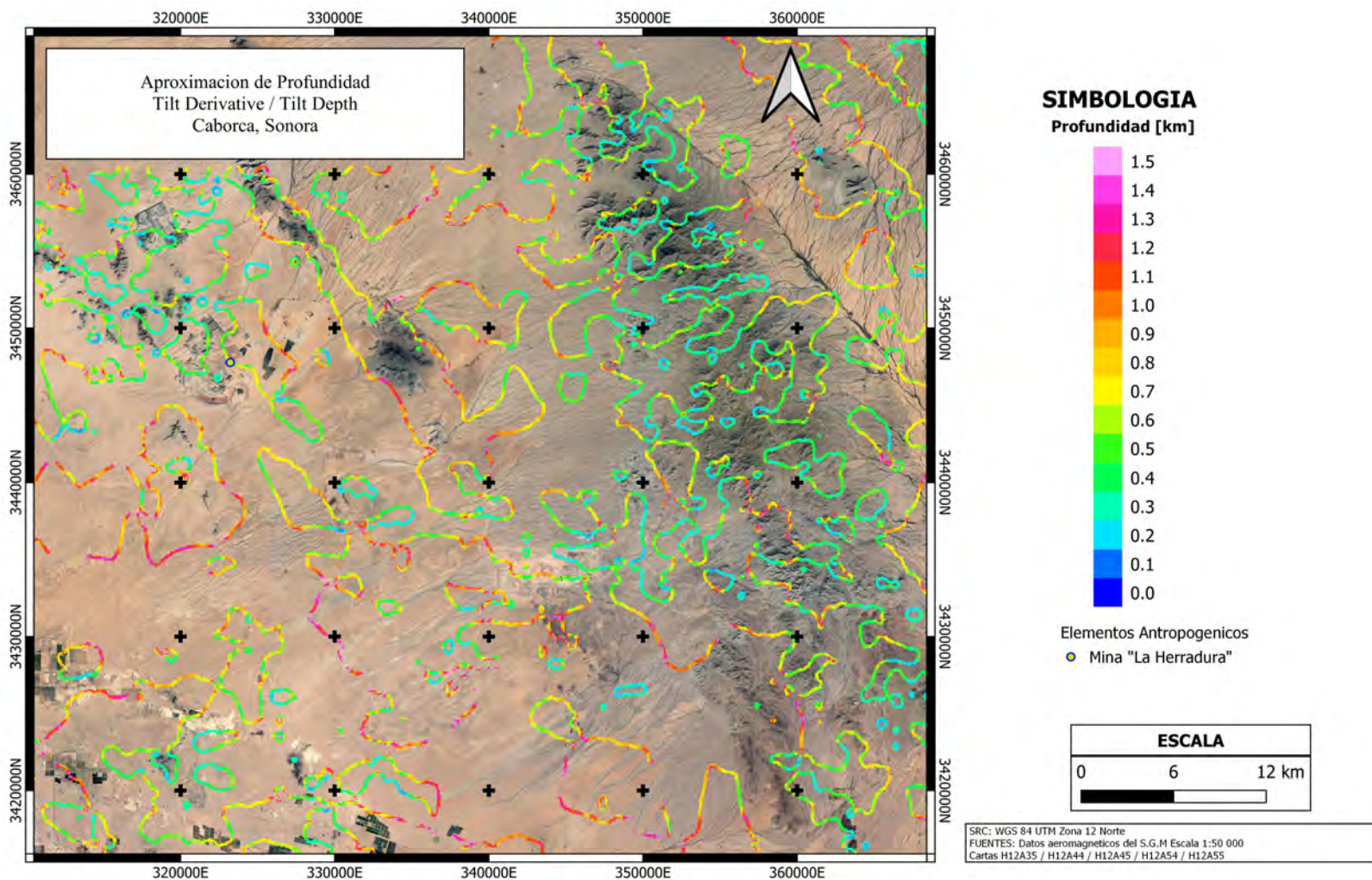
Figura 27: Estimación de profundidad de los bordes de las anomalías magnéticas, proveniente del tilt depth.
