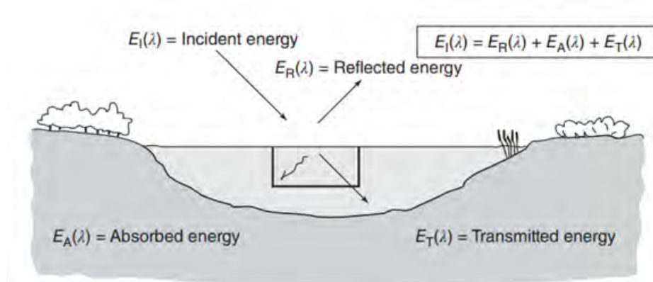
Figura 3: Diagrama de la interacción entre la energía incidente y la superficie, donde se muestra la separación en energía absorbida, reflejada y transmitida. (Lillesand et al., 2015)
