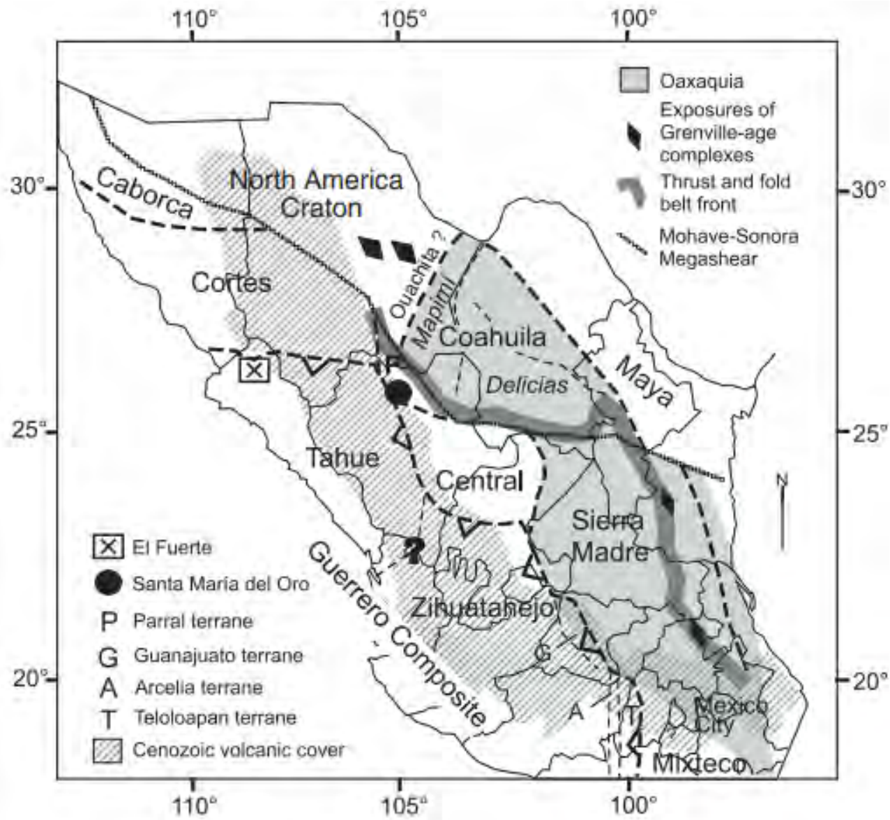
Figura 12: Terrenos Tectono-estratigráficos del norte de México (Centeno-García, 2005)
