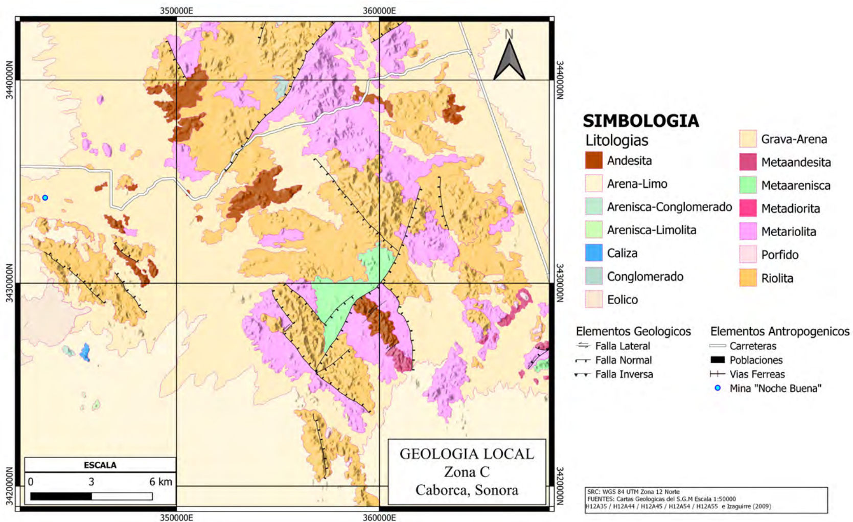
Figura 18: Ampliación del mapa geológico del área de estudio.
