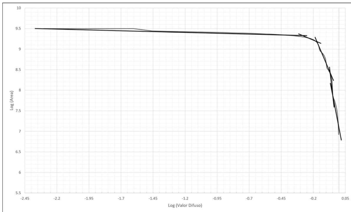
Figura 52: Gráfico de concentración-área del mapa de integración resultante con el operador gamma difuso.
