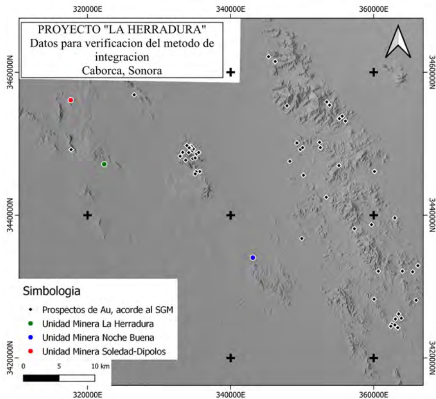
Figura 50: Ubicación de los depósitos y/o prospectos de oro reportados por el Servicio Geológico Mexicano (2012a, 2012b, 2015a, 2015b, 2015c).
