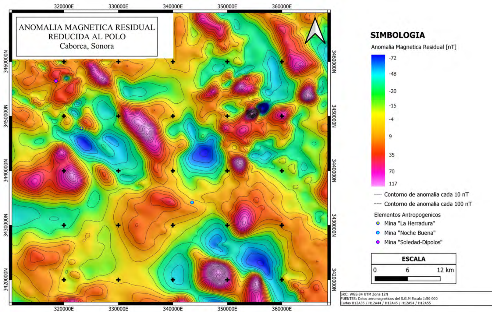
Figura 24: Anomalia magnética residual reducida al polo.
