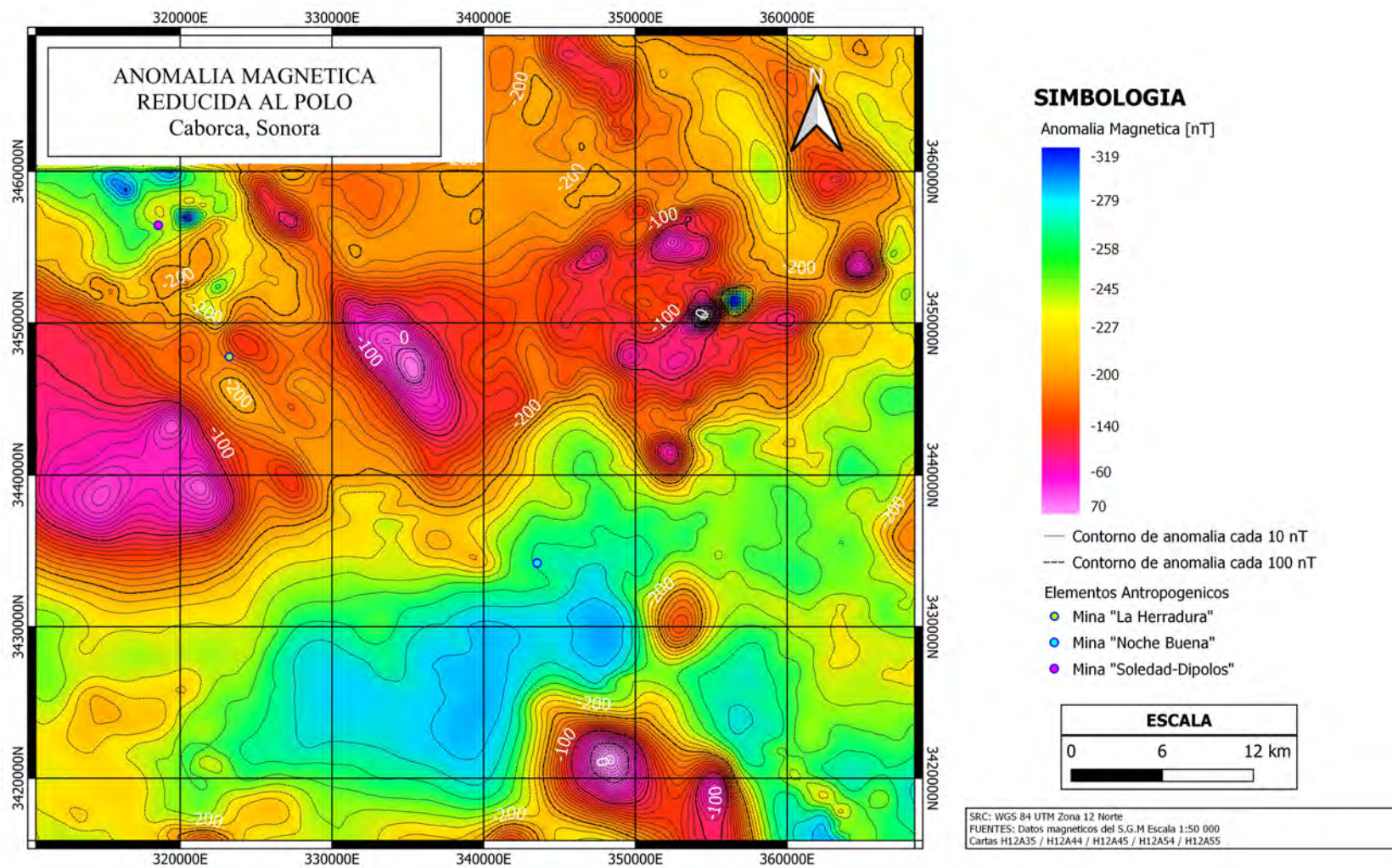
Figura 23: Anomalia magnética de campo total reducida al polo.
