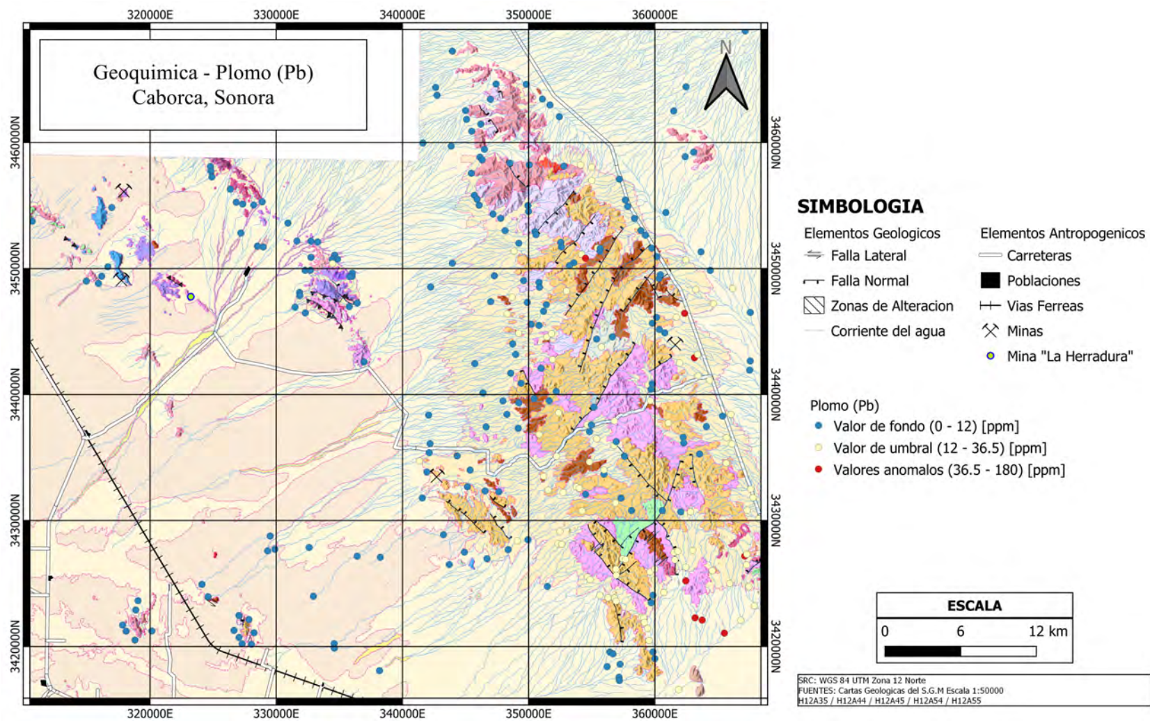
Figura 39: Mapa de la distribución del Plomo en los sedimentos de arroyo del área de estudio.
