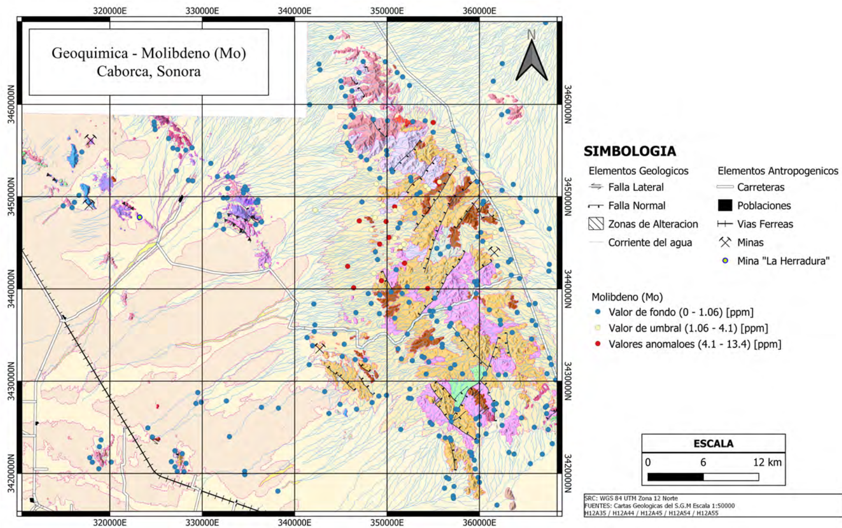
Figura 37: Mapa de la distribución del Molibdeno en los sedimentos de arroyo del área de estudio.
