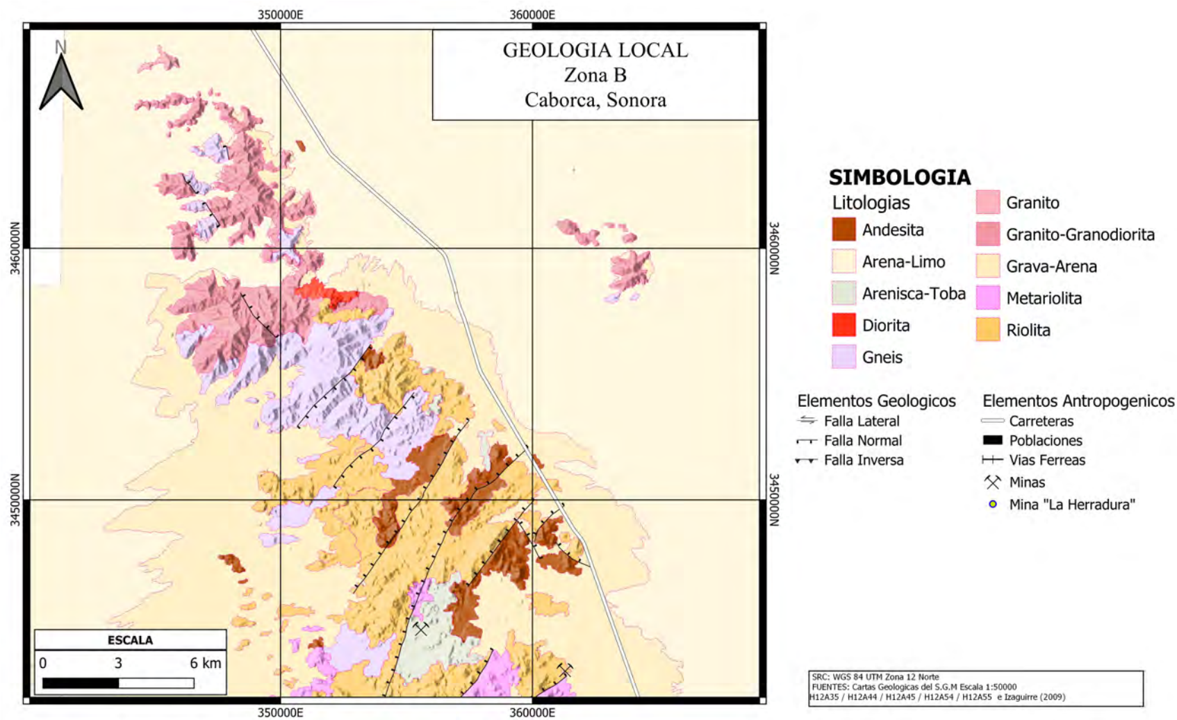
Figura 17: Ampliación del mapa geológico del área de estudio.
