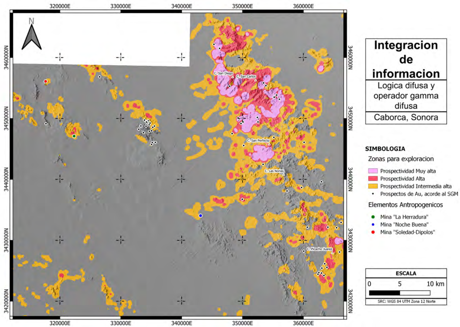
Figura 54: Zonas designadas para exploración, obtenidas con el sistema difuso y el operador gamma.
