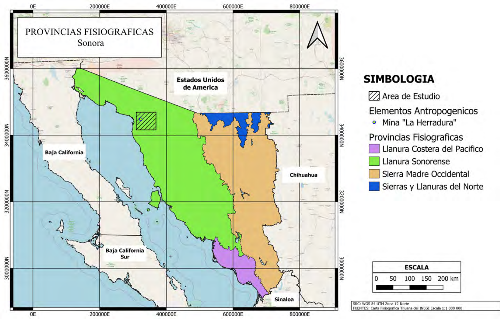
Figura 10: Provincias fisiográficas del estado de Sonora con la ubicación del área de estudio.
