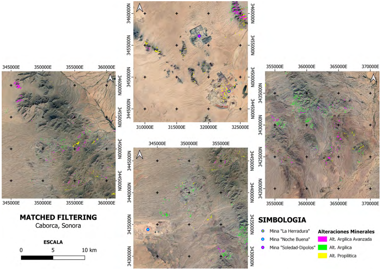
Figura 46: Acercamiento a las alteraciones minerales identificadas mediante el método Matched Filtering
