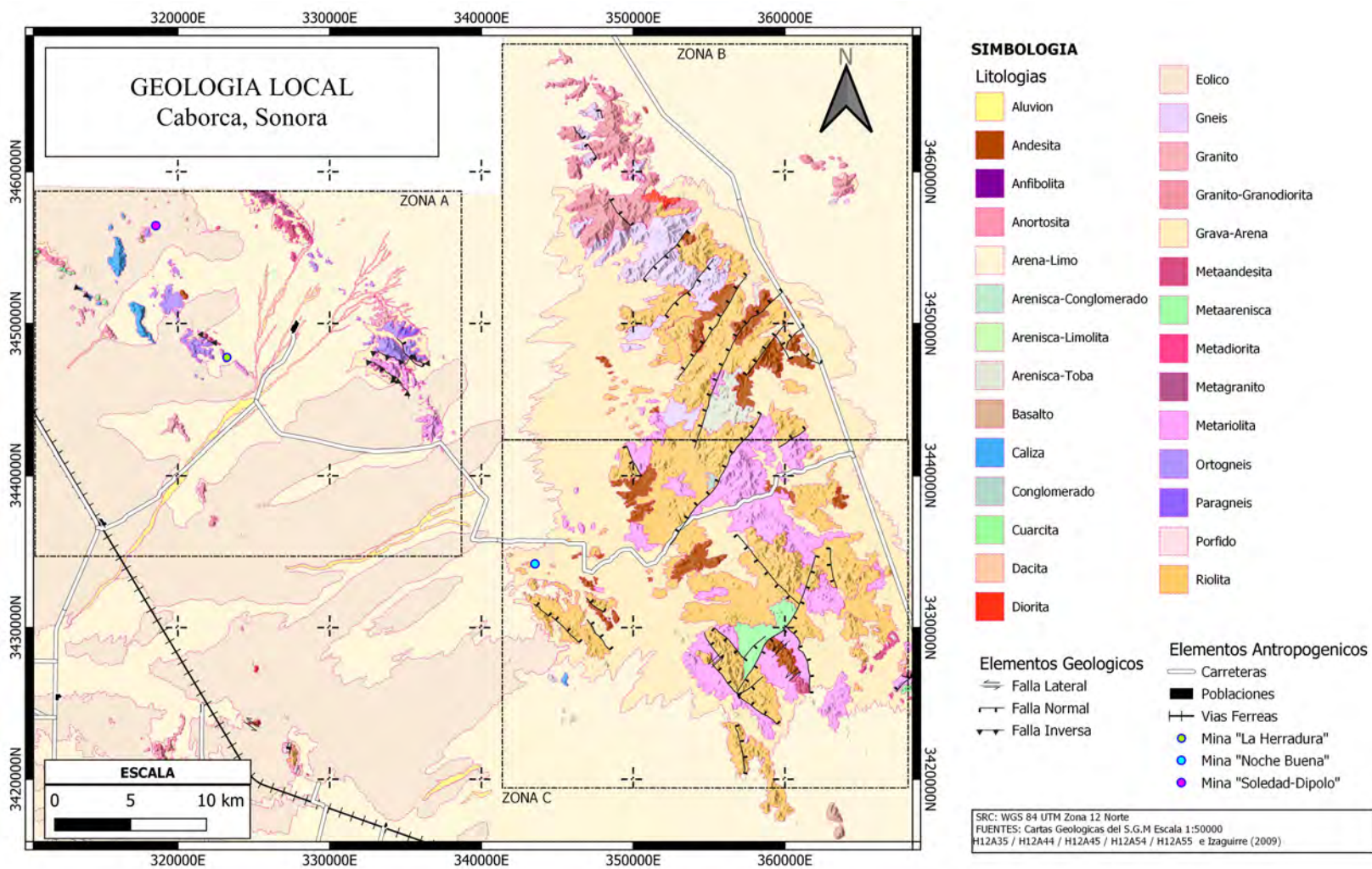
Figura 15: Mapa geológico del área de estudio.
