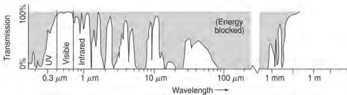
Figura 2: Longitudes de onda del espectro electromagnético con la señalización de las regiones afectadas por la absorción atmosférica en color gris y las ventanas atmosféricas en blanco. (Lillesand et al., 2015)
