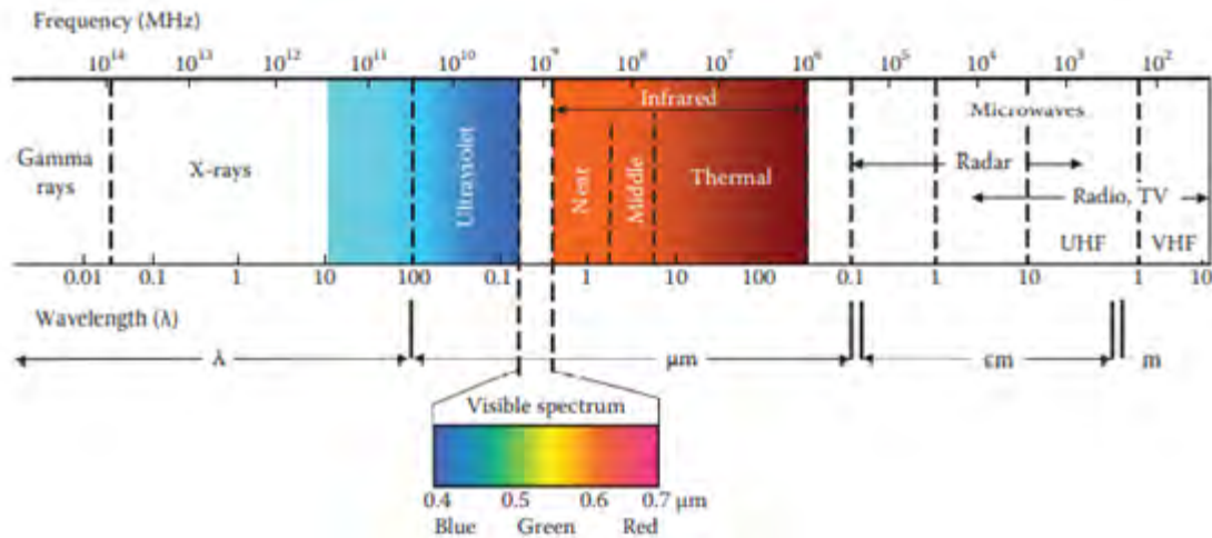
Figura 5: Espectro electromagnético indicando las subdivisiones en regiones principales, con énfasis en el ultravioleta (UV), el espectro visible (V) y el infrarrojo (IR). Se muestran las frecuencias en megahertz [MHz] y las longitudes de onda en ángstrom [Å], micrometros [ \mu m ], centímetros [cm] y metros [m]. (Chuvieco, 2016)
