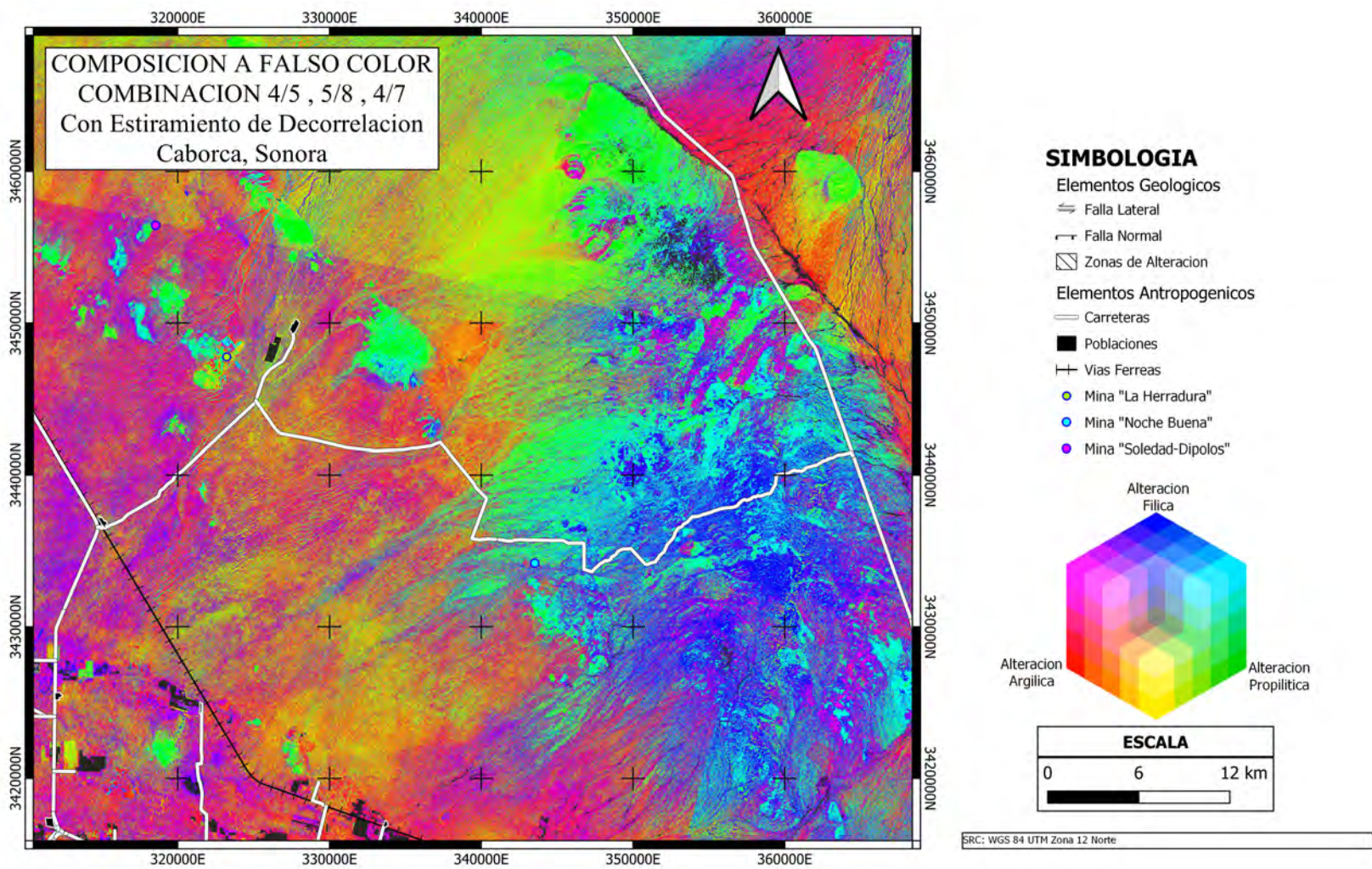
Figura 43: Composición a falso color con la alteración argílica en el rojo (R), la alteración propilítica en el verde (G) y la alteración fílica en el azul (B), a la cual se le aplico un estiramiento de decorrelación.
