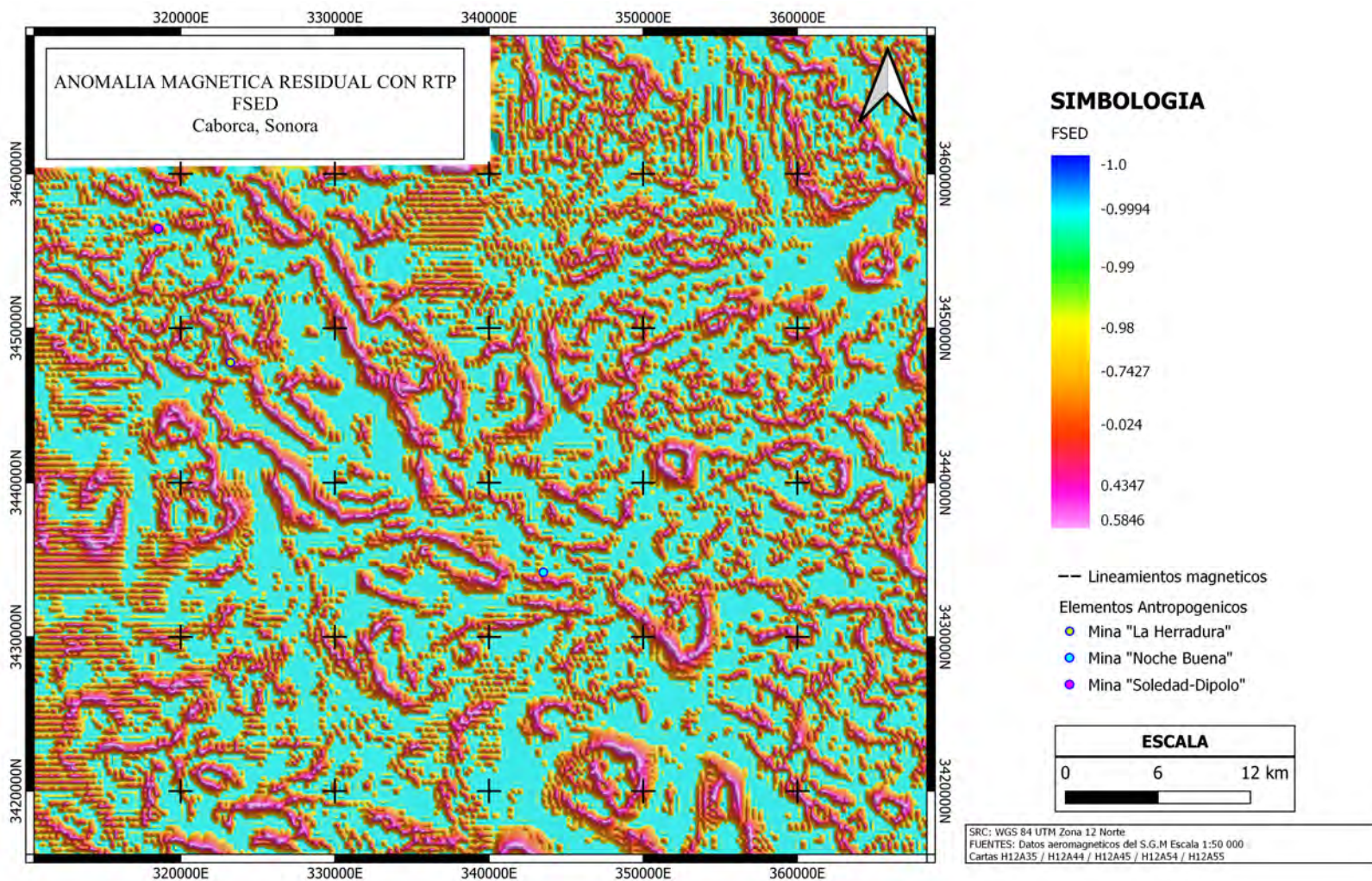
Figura 28: FSED de la anomalía magnética residual reducida al polo.
