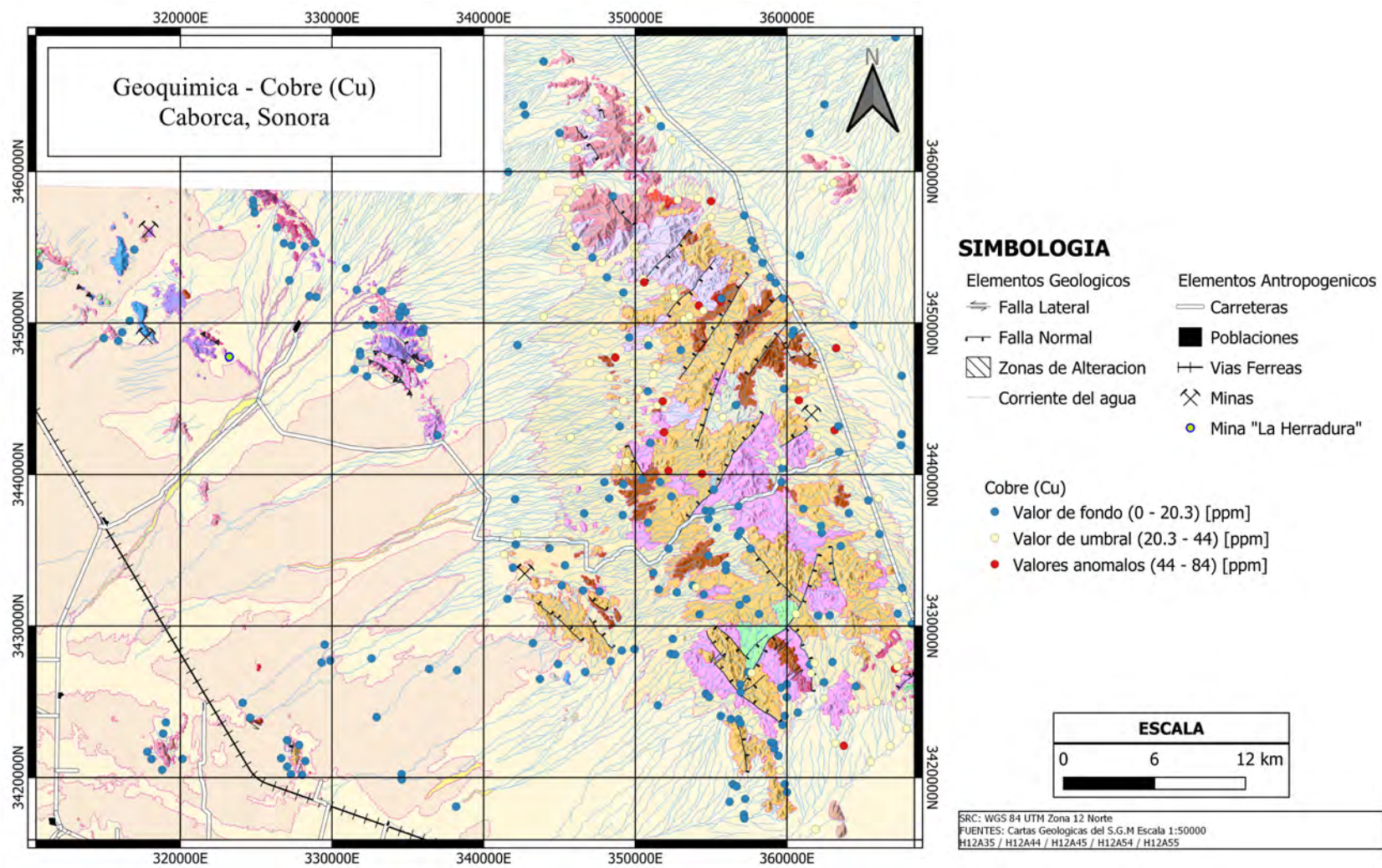
Figura 34: Mapa de la distribución del Cobre en los sedimentos de arroyo del área de estudio.
