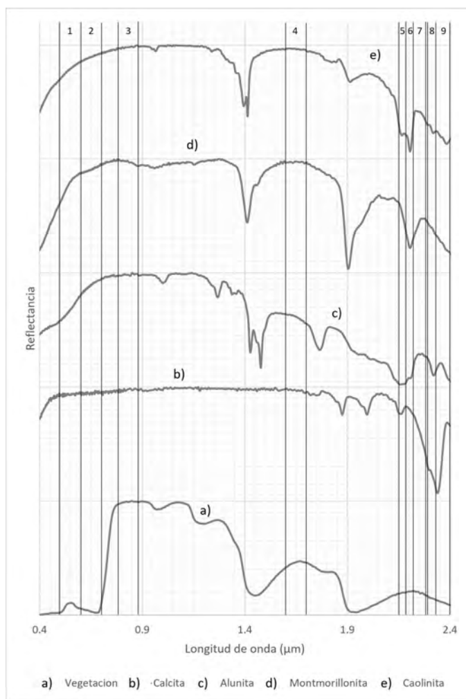
Figura 7: Bandas espectrales ASTER en VNIR y SWIR, y las firmas espectrales de minerales y vegetación común: a) Vegetación, b) Calcita c) Alunita, d) Montmorillonita, e) Caolinita.
