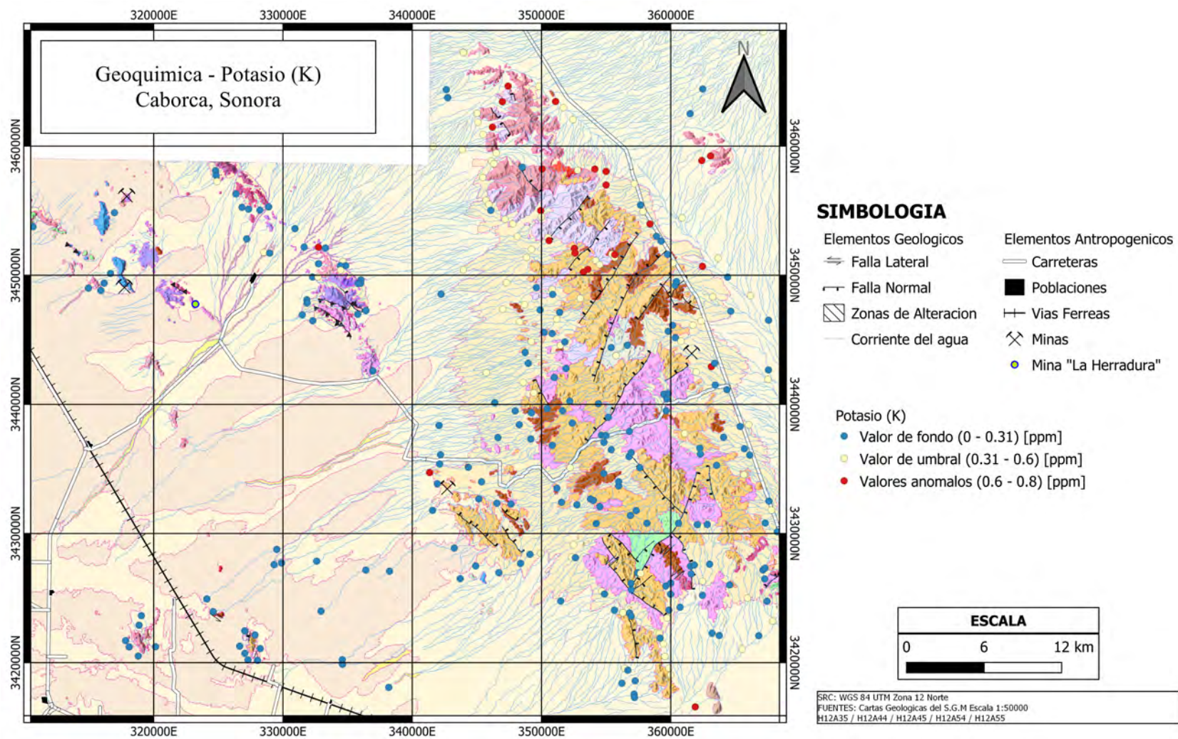
Figura 36: Mapa de la distribución del Potasio en los sedimentos de arroyo del área de estudio.
