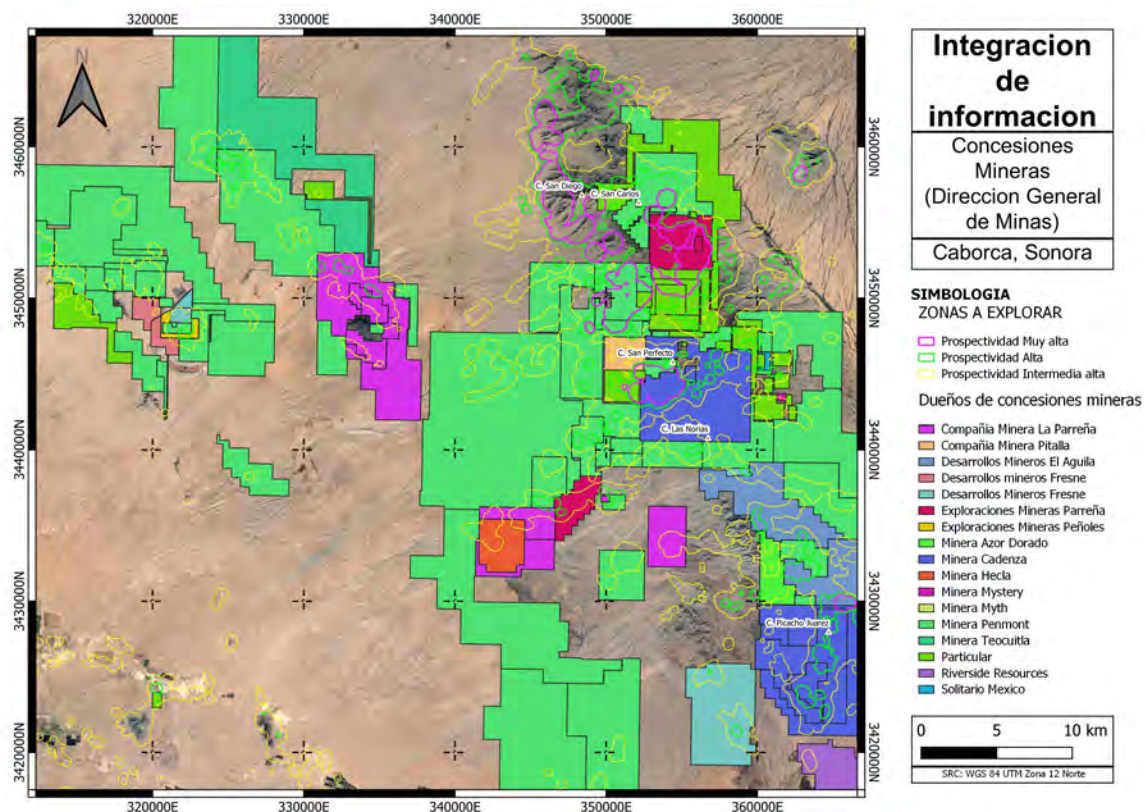
Figura 55: Concesiones mineras vigentes sobre las zonas propuestas para campañas de exploración, con información de la Dirección General de Minas (DGM).
