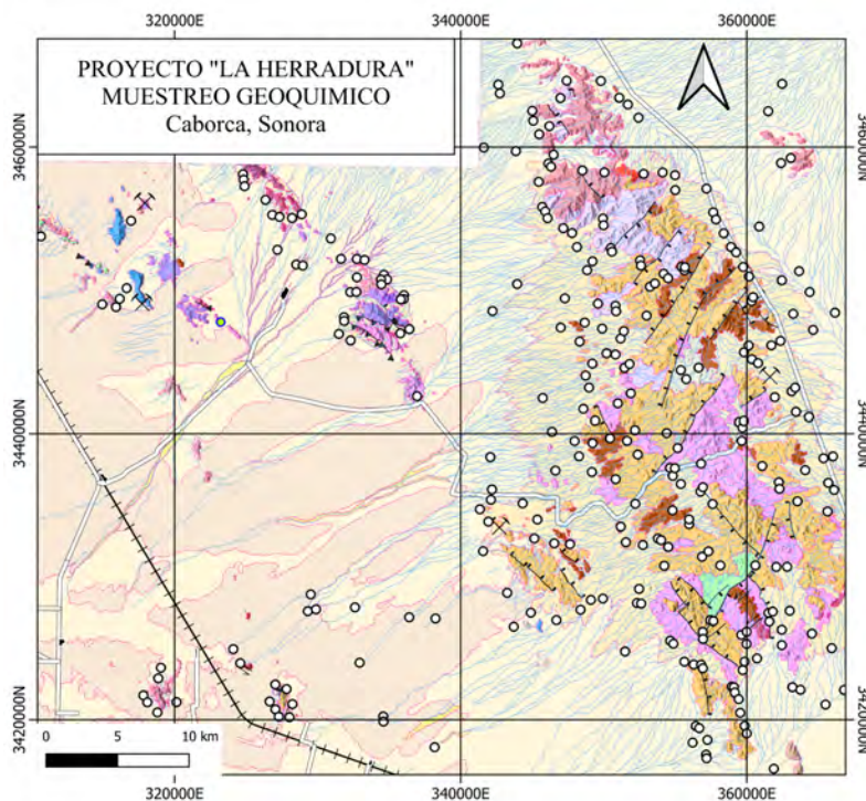
Figura 30: Ubicación de las muestras de sedimento de arroyo tomadas por el Servicio Geológico Mexicano.
