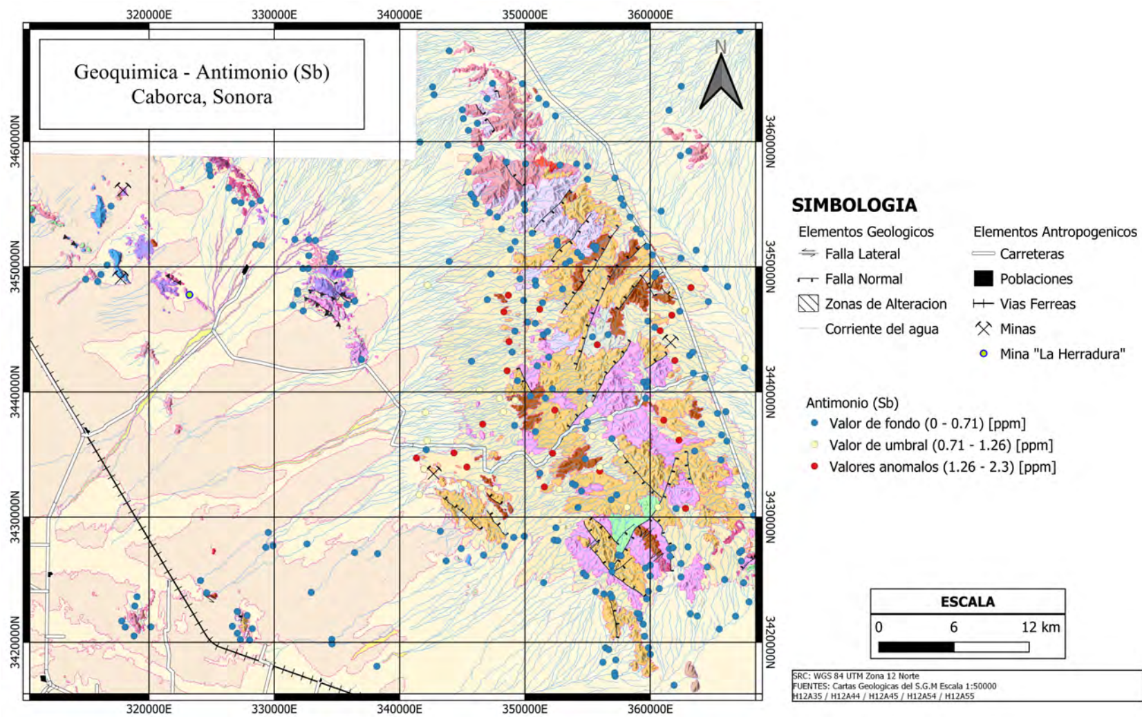
Figura 40: Mapa de la distribución del Antimonio en los sedimentos de arroyo del área de estudio.
