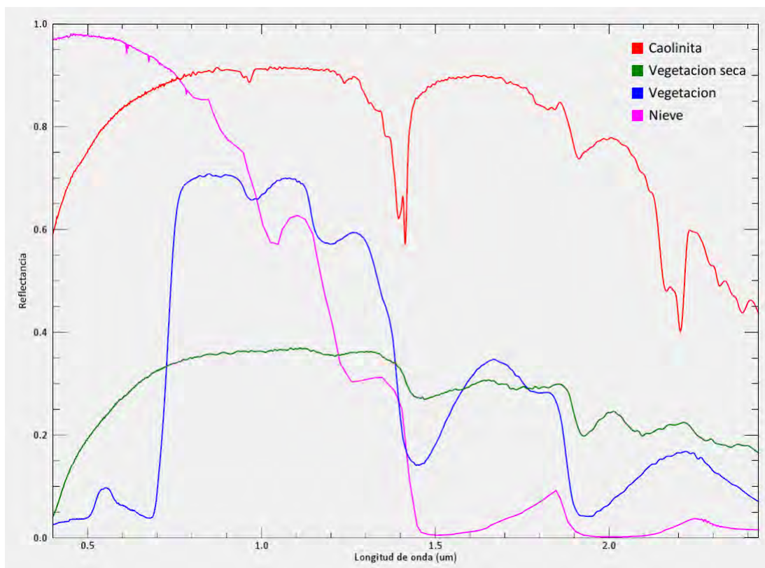
Figura 4: Firmas espectrales de vegetación, vegetación seca, nieve y caolinita. (Con información de Kokaly et al., 2017)
