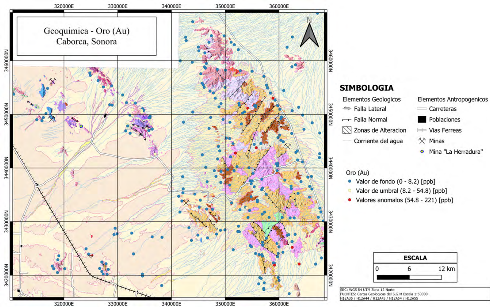
Figura 32: Mapa de la distribución del Oro en los sedimentos de arroyo del área de estudio.
