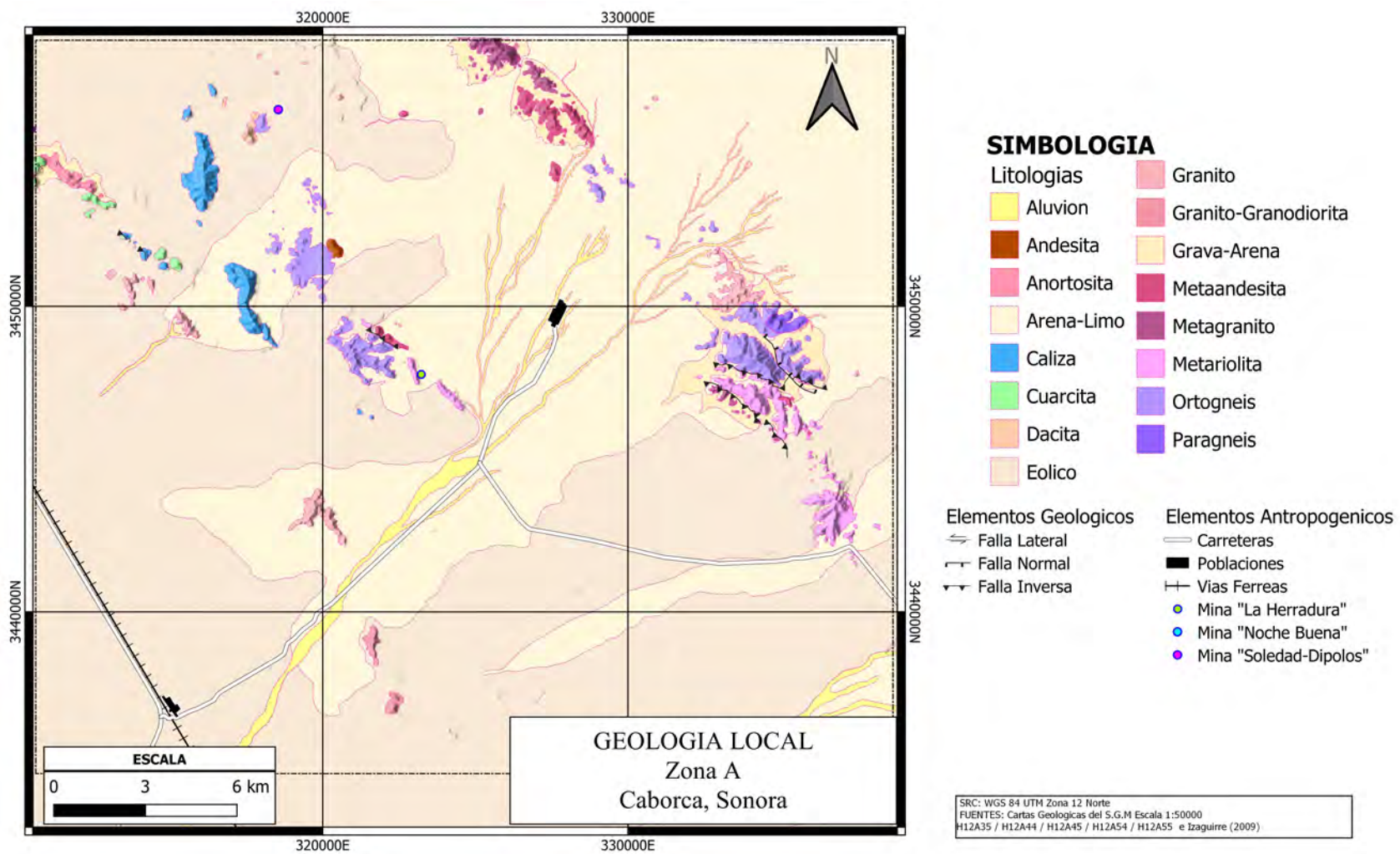
Figura 16: Ampliación del mapa geológico del área de estudio.
