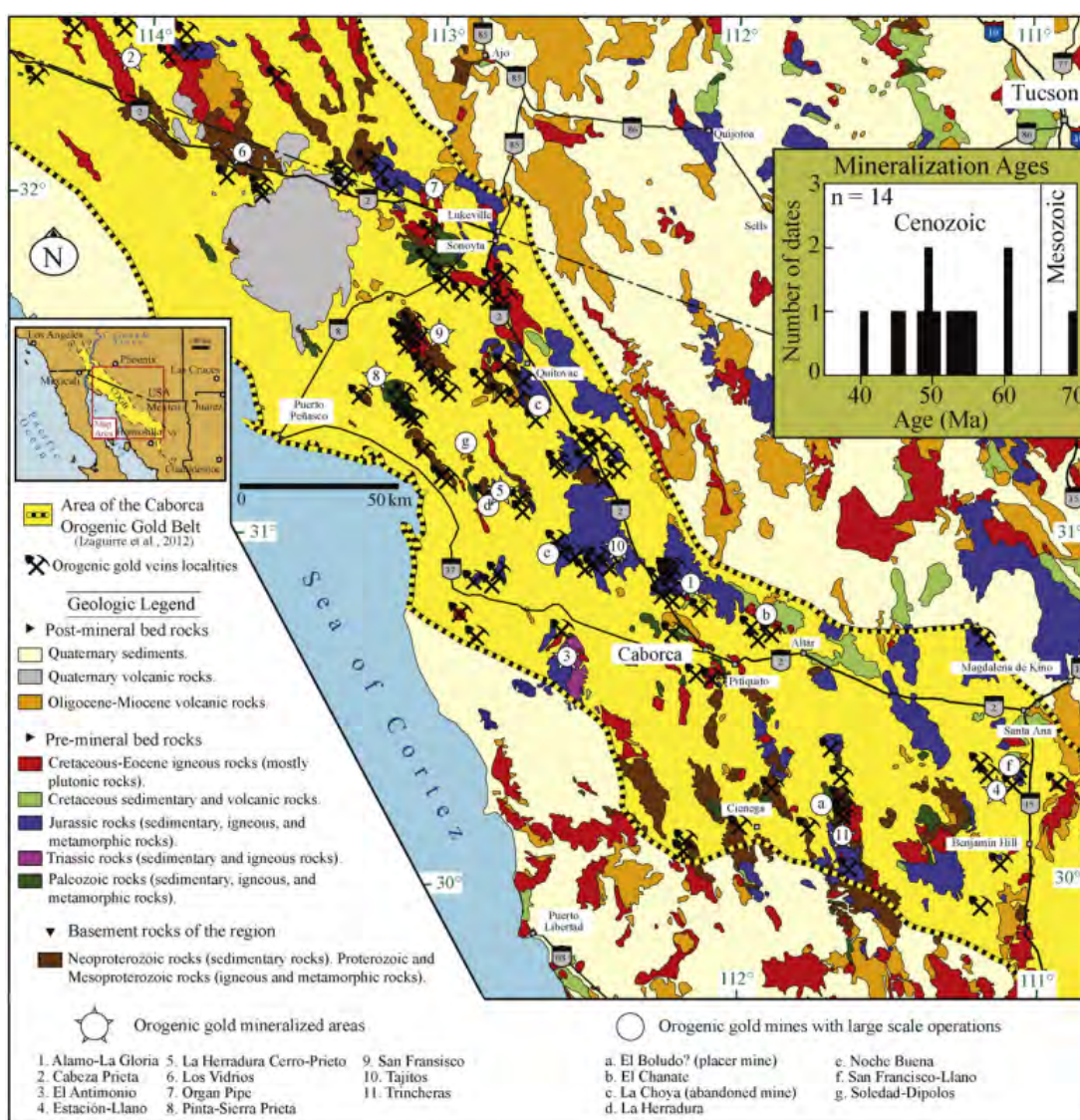
Figura 19: Ubicación y distribución del Cinturón de Oro orogénico de Caborca (Izaguirre et al., 2017).
