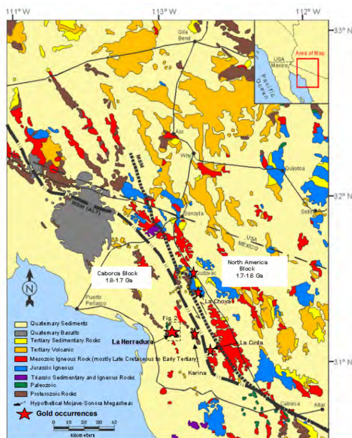
Figura 13: Mapa geológico regional con propuestas de la ubicación de la Megacizalla Mojave - Sonora (Quintanar Ruiz, 2008)
