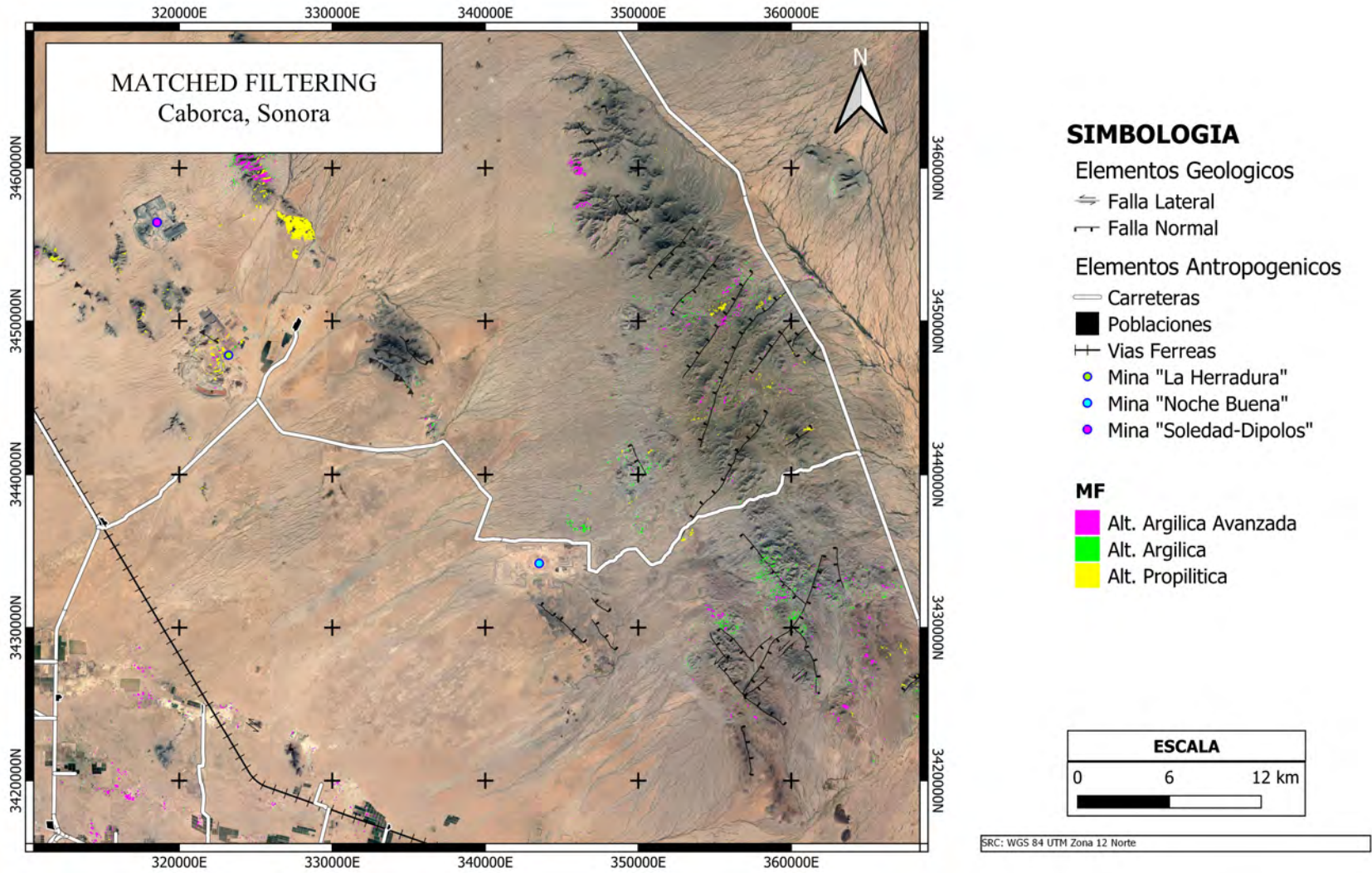
Figura 45: Identificación de alteraciones minerales mediante el método Matched Filtering
