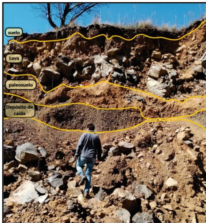
Figura 40. Fotografía del afloramiento STM-1904 (ver Fig. 16 para la ubicación) en donde se observa un depósito de caída de escoria, sobreyacido por un paleosuelo, que a su vez es cubierto por el flujo de lava III y el suelo moderno. La persona de la fotografía mide 1.80 m.
