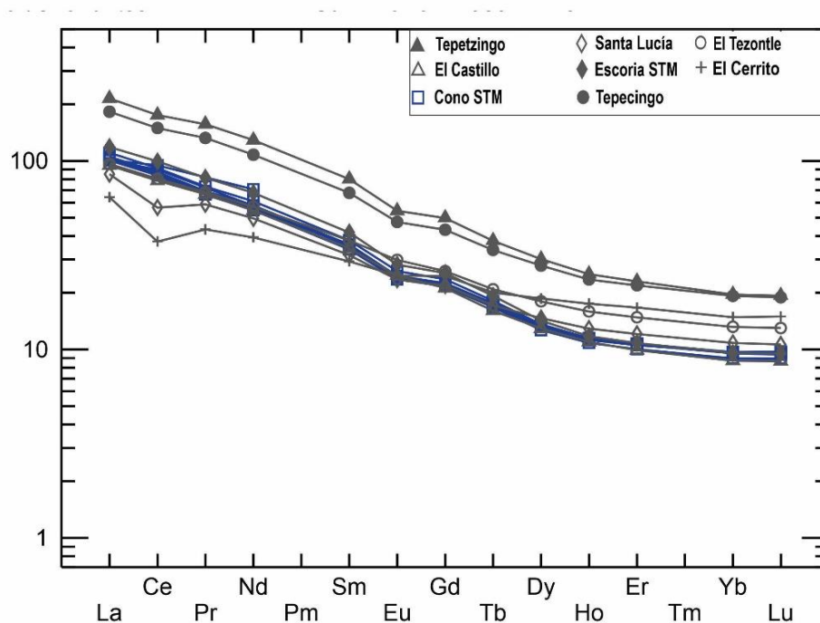
Figura 64. Diagrama de elementos de tierras raras normalizado con los valores de una condrita (Sun y McDonough, 1989) de las rocas estudiadas. Resalta el enriquecimiento de las tierras raras ligeras en comparación con las tierras raras pesadas para todas las muestras.
