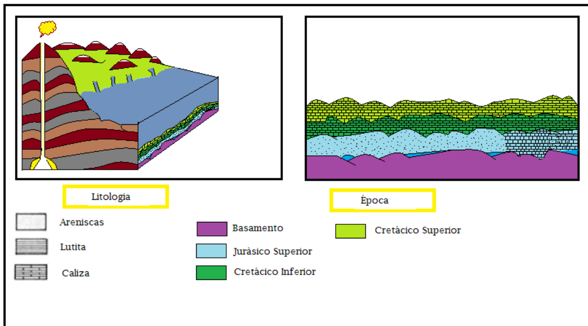
Figura 2.9. Paleoambiente del Cretácico (modificado de Echanove, 1986)
