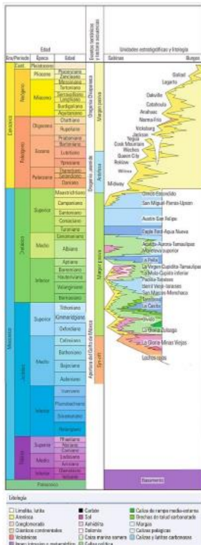
Figura 2.3. Cuenca de Sabinas y Burgos (modificado de WEC, 2009)
