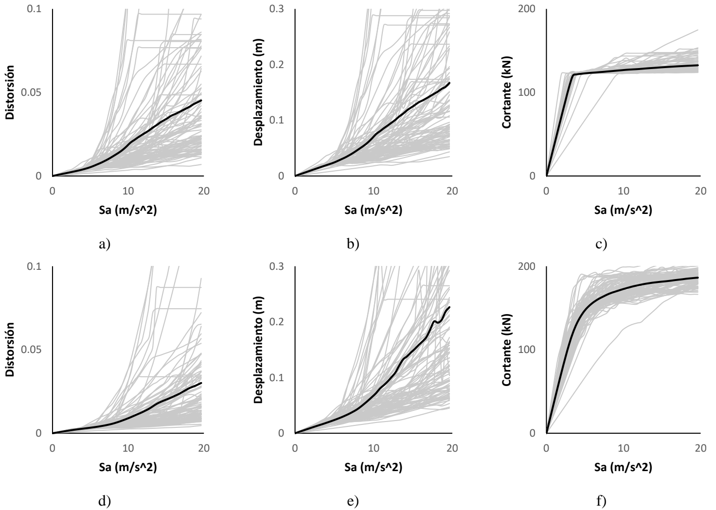
Figura 9. Curvas IDA para las escuelas originales de dos niveles diseñadas conforme a: MOC-CFE-1993 (a, b y c) y MOC-CFE-2008 (d, e, y f)
