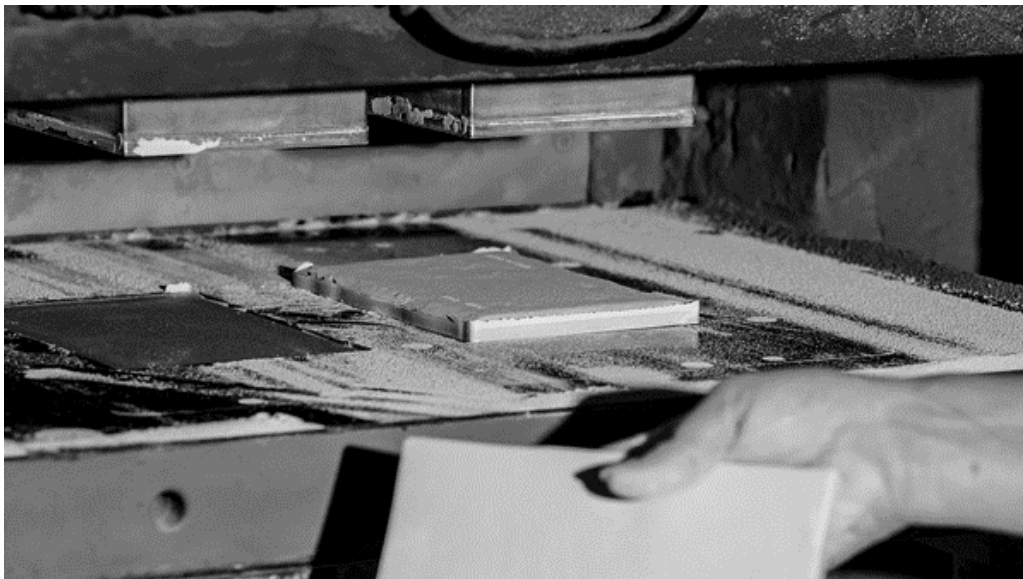
Figura 3.3 Prensado de la arcilla en seco (Bizpren , 2022)
