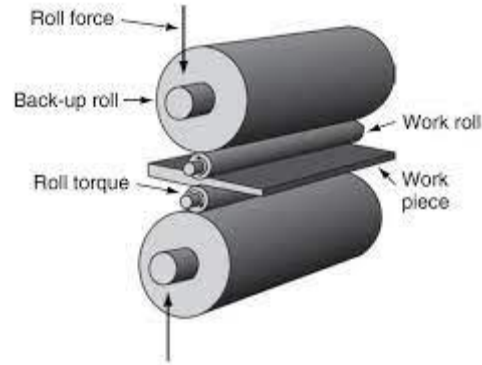
Figura 3.9 Diagrama esquemático mostrando la interacción de los rodillos y la lámina, J. G. Lenard, Primer on Flat Rolling , Elsevier., (2021).
