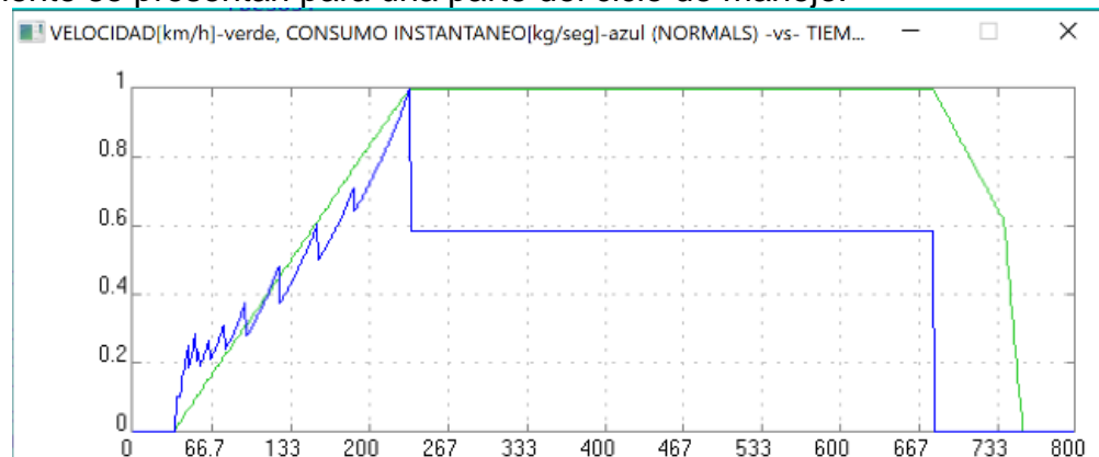
Figura 16. Rapidez y consumo instantáneo normalizados contra el tiempo (seg) para la tercera parte del ciclo de conducción. Motor 350 HP, M = 19.752 tons (carga 10 tons), inclinación 0^\circ .
