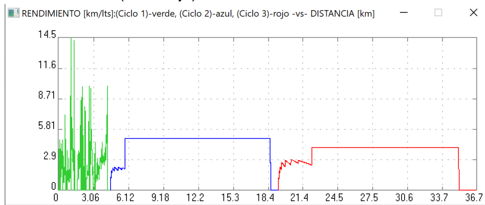
Figura 28. Rendimiento de combustible del vehículo pesado en km/lit contra el tiempo en segundos para la primera parte (línea verde), la segunda parte (línea azul) y la tercera parte (línea roja) del ciclo de manejo.
