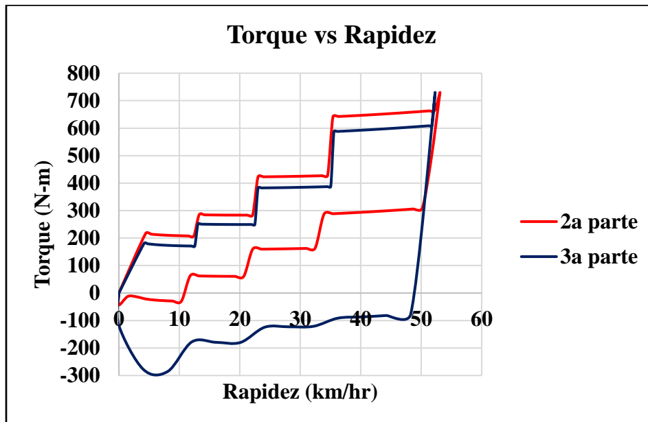
Figura 59. Torque contra la velocidad para la segunda y tercera partes del ciclo de manejo. Motor 200 HP, M = 6.407 tons (2 tons de carga), inclinación 6^\circ .
