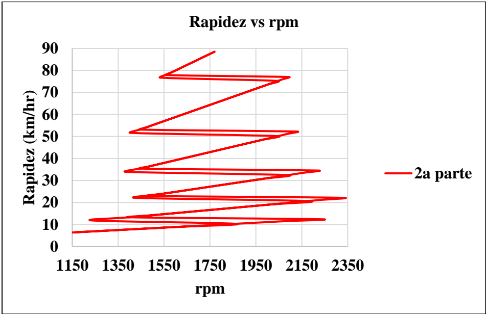
Figura 47. Rapidez del vehículo contra las rpm del motor para la segunda parte del ciclo de manejo. Motor 200 HP, M = 4.407 tons (sin carga), inclinación 0^\circ .
