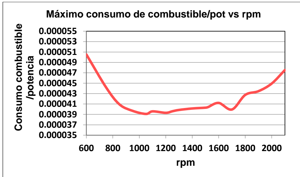
Figure 6. Valores del consumo específico del motor contra las rpm del motor para los valores máximos del torque.
