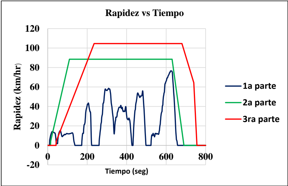
Figura 46. Rapidez del vehículo contra el tiempo. Se muestran las 3 partes del ciclo completo.
