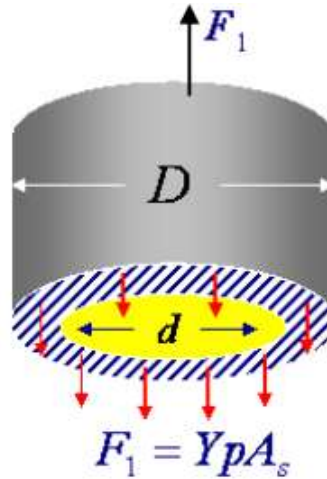
Figura 1.16 Tensión aplicada a la tubería de producción 16
