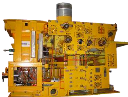
Figura 2.7 Árbol horizontal 33
