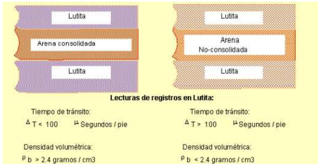
Figura 1.8 Arena consolidada 8
