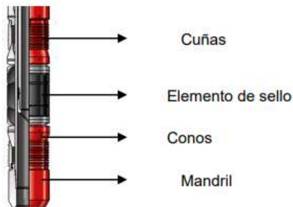
Figura 1.24 Empacadores permanentes 24
