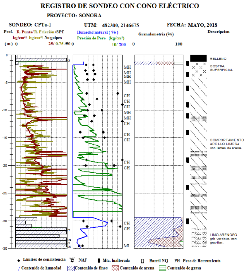
Figura 4.13. Perfil estratigráfico para la zona de estudio (Amezcue, 2019)
