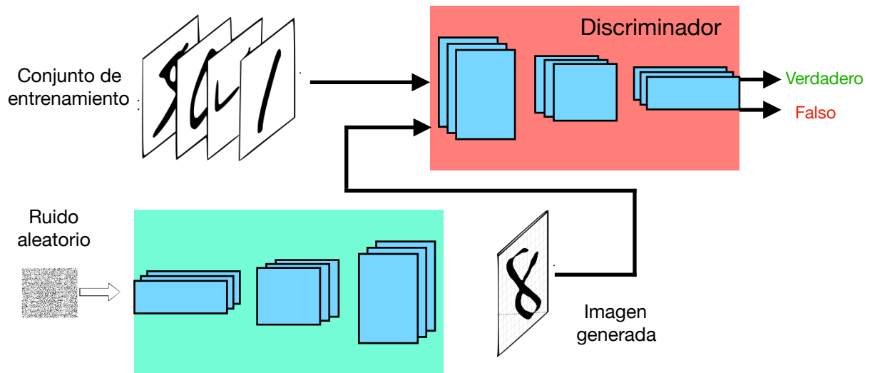
FIGURA 2.24 DIAGRAMA DE BLOQUES DE UNA RED ADVERSARIA GENERATIVA. (Figura inspirada en [22])
