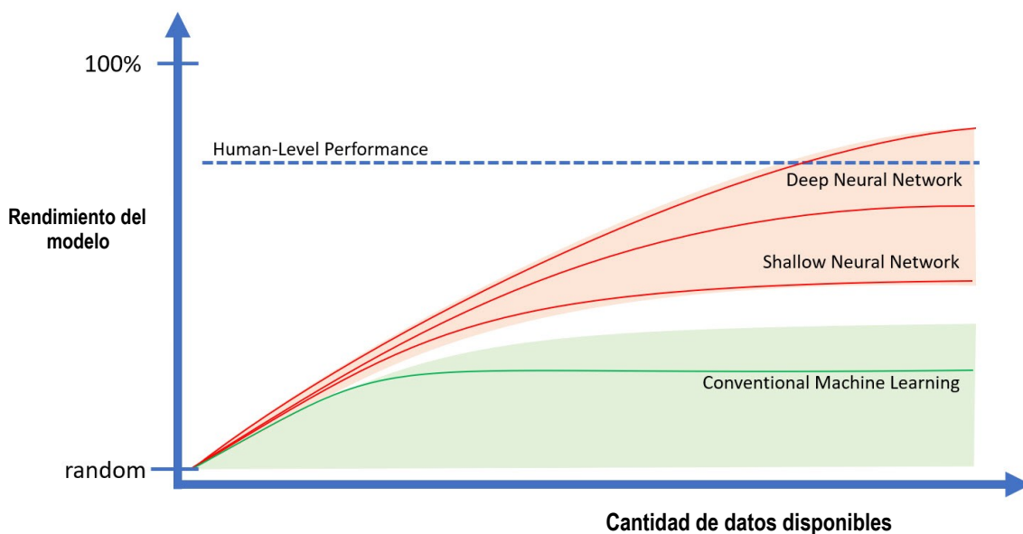
FIGURA 2.13 COMPARACIÓN DEL RENDIMIENTO DEL APRENDIZAJE PROFUNDO EN FUNCIÓN DE LA CANTIDAD DE DATOS DISPONIBLES. (Figura modificada de [13])
