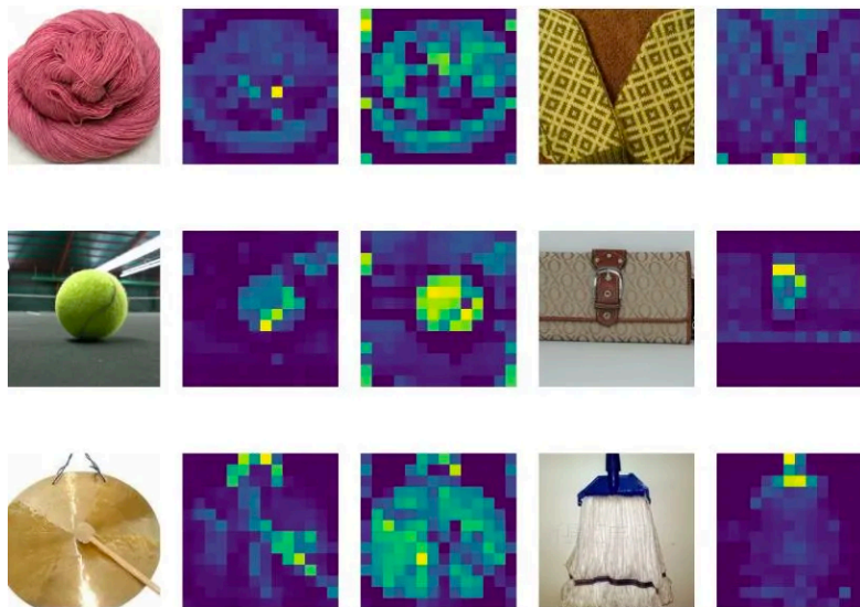
FIGURA 2.19 MAPAS DE ATENCIÓN QUE ILUSTRAN LA IMPORTANCIA QUE LE DA UNA CAPA DEL ViT A UNA REGIÓN EN ESPECÍFICO DE LA IMAGEN DE ENTRADA.
