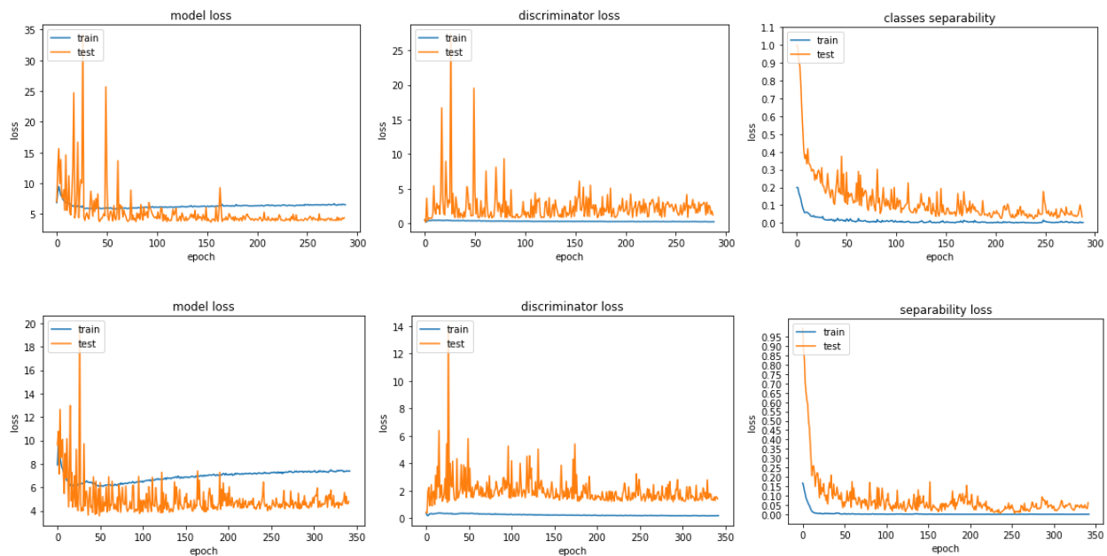
FIGURA 4.1 GRÁFICAS DEL ERROR TOTAL DEL MODELO (IZQUIERDA), DEL ERROR POR PARTE DEL DISCRIMINADOR(CENTRO) Y DEL ERROR DE SEPARABILIDAD DEL MODELO(DERECHA) PARA LOS ENTRENAMIENTOS EN EL QUE SOLO SE BUSCA LA SEPARABILIDAD DE LA MEDIA PARA EL DATASET DE FIGURAS GEOMÉTRICAS(SUPERIOR) Y EL DATASET DE OBJETOS DE MANUFACTURA(INFERIOR).
