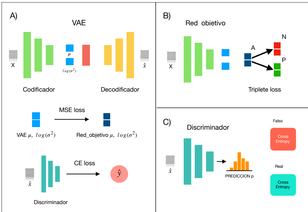
FIGURA 3.13 ELEMENTOS QUE COMPONEN A EL MODELO G-VAE.
