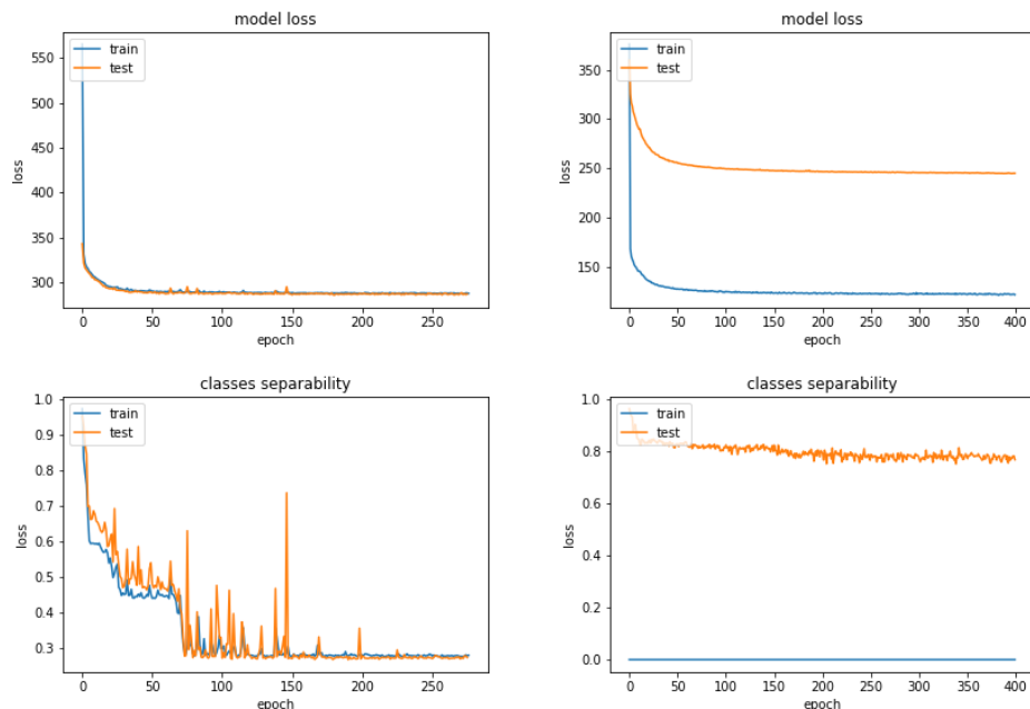
FIGURA 3.12 GRÁFICAS DE LAS FUNCIONES DE PERDIDA(SUPERIOR) Y SEPARABILIDAD(INFERIOR) DEL MODELO PARA LOS ENTRENAMIENTOS DE ESTE SIN OPTIMIZAR LA SEPARABILIDAD(IZQUIERDA) Y OPTIMIZANDO LA SEPARABILIDAD(DERECHA)
