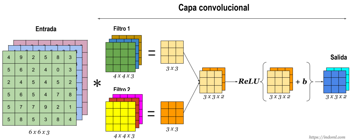
FIGURA 2.16 PROCESAMIENTO DE UNA IMAGEN DE ENTRADA POR UNA CAPA CONVOLUCIONAL. (Figura modificada de [16])
