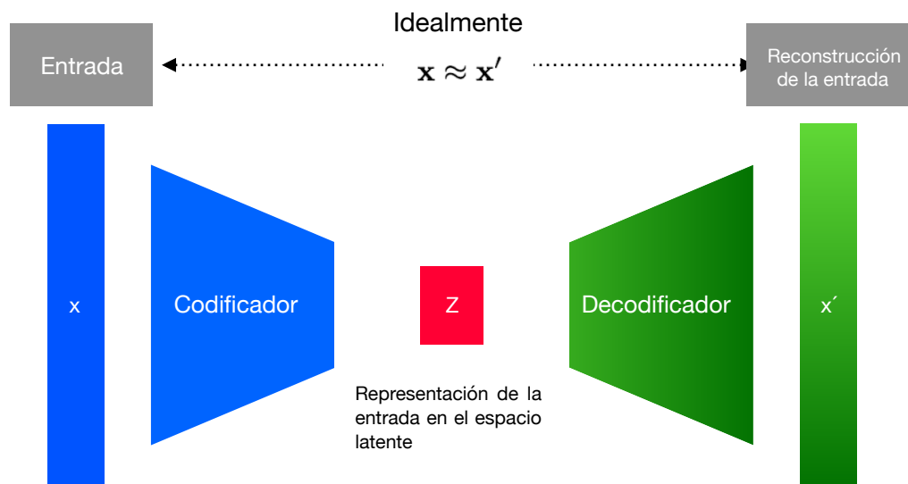
FIGURA 2.22 DETALLE DE LOS BLOQUES Y FUNCIONAMIENTO DE UN AUTOCODIFICADOR. (Figura inspirada en [21])
