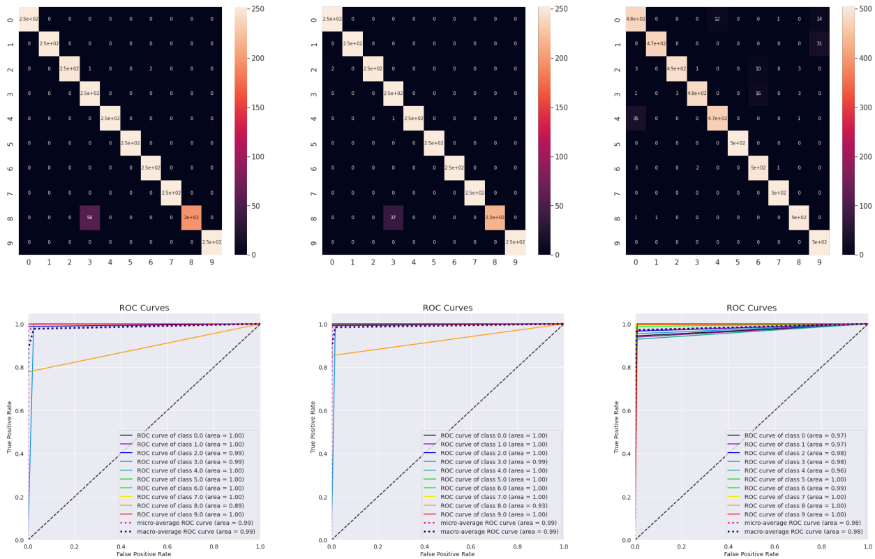
FIGURA 4.6 RESULTADOS DEL PROCESO DE CLASIFICACIÓN DE IMÁGENES DEL MODELO CNN(IZQUIERDA), DEL MODELO QUE USA A LAS REPRESENTACIONES APRENDIDAS(CENTRO) Y DEL MODELO BOF+NN(DERECHA).
