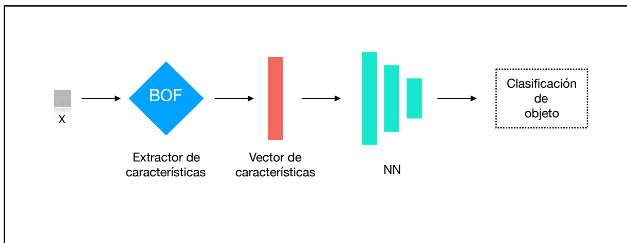
FIGURA 3.15 PROCESO DE INFERENCIA MEDIANTE EL USO DEL MODELO BOF+NN
