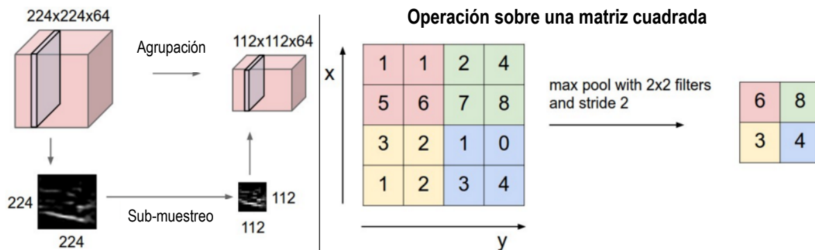
FIGURA 2.17 APLICACIÓN DE UNA CAPA DE SUB-MUESTREO A DIFERENTES ENTRADAS. (Figura modificada de [17])
