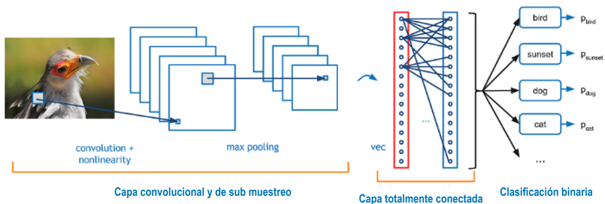
FIGURA 2.14 COMPOSICIÓN INTERNA DE UNA RED CONVOLUCIONAL. (Figura modificada de [14])
