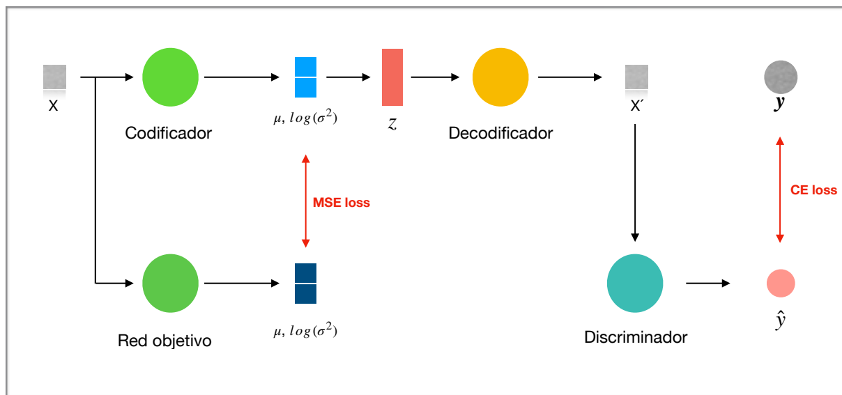
FIGURA 3.14 CICLO DE ENTRENAMIENTO DE EL AUTOCODIFICADOR VARIACIONAL.
