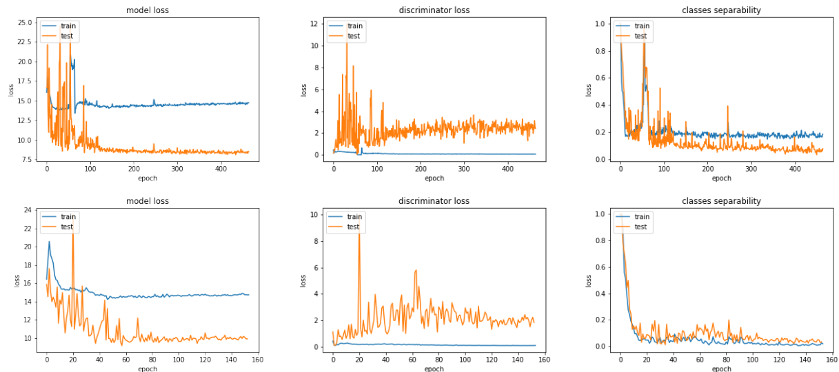
FIGURA 4.4 GRÁFICAS DEL ERROR TOTAL DEL MODELO (IZQUIERDA), DEL ERROR POR PARTE DEL DISCRIMINADOR(CENTRO) Y DEL ERROR DE SEPARABILIDAD DEL MODELO(DERECHA) PARA LOS ENTRENAMIENTOS EN LOS QUE SE BUSCA LA SEPARABILIDAD DE TODOS LOS PARÁMETROS DE LAS DISTRIBUCIONES PARA EL DATASET DE FIGURAS GEOMÉTRICAS(SUPERIOR) Y EL DATASET DE OBJETOS DE MANUFACTURA(INFERIOR).
