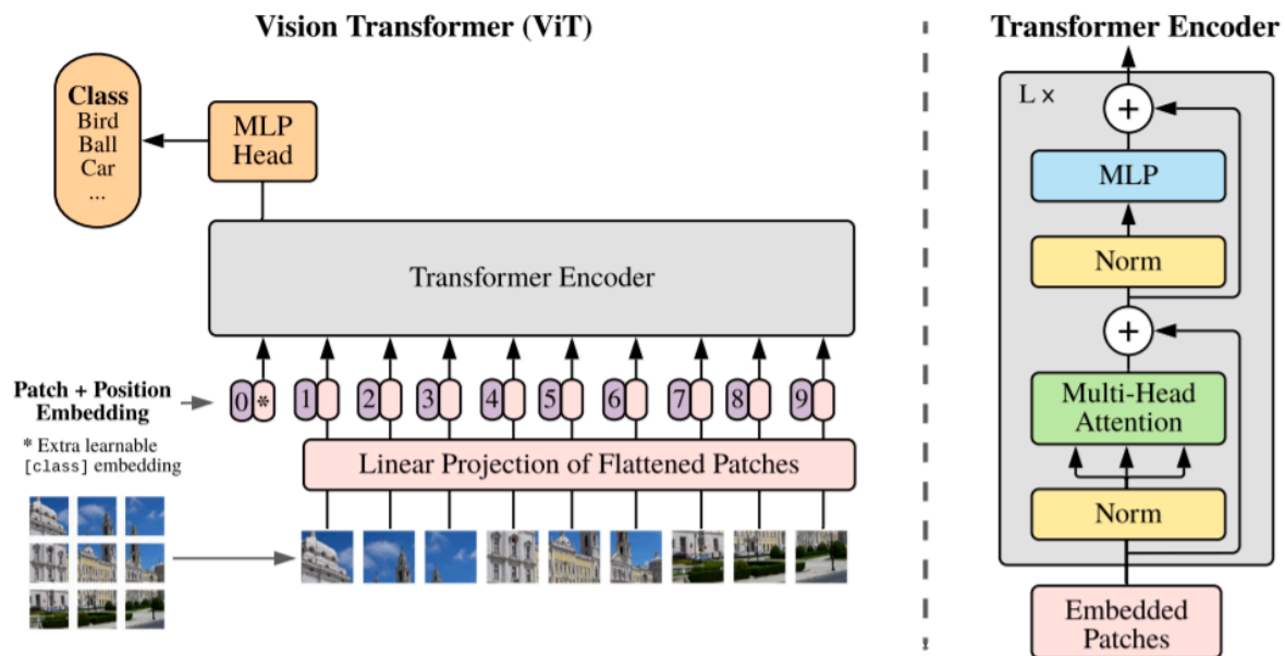
FIGURA 2.20 (IZQUIERDA) ARQUITECTURA GENERAL DE UN VISION TRANSFORMER, (DERECHA) COMPONENTES INTERNOS QUE COMPONEN A EL CODIFICADOR. (Figura tomada de [20])
