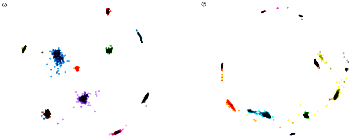
FIGURA 4.5 VISUALIZACIÓN DE LOS PARÁMETROS DEL ESPACIO LATENTE DEL MODELO HACIENDO USO DE UNA REDUCCIÓN PCA PARA EL CASO EN EL QUE SE REGULARIZA LA SEPARABILIDAD DE LOS PARÁMETROS DE MEDIA(IZQUIERDA) Y EN LA CUAL SE REGULARIZA A TODOS LOS PARÁMETROS DE LAS DISTRIBUCIONES(DERECHA) .
