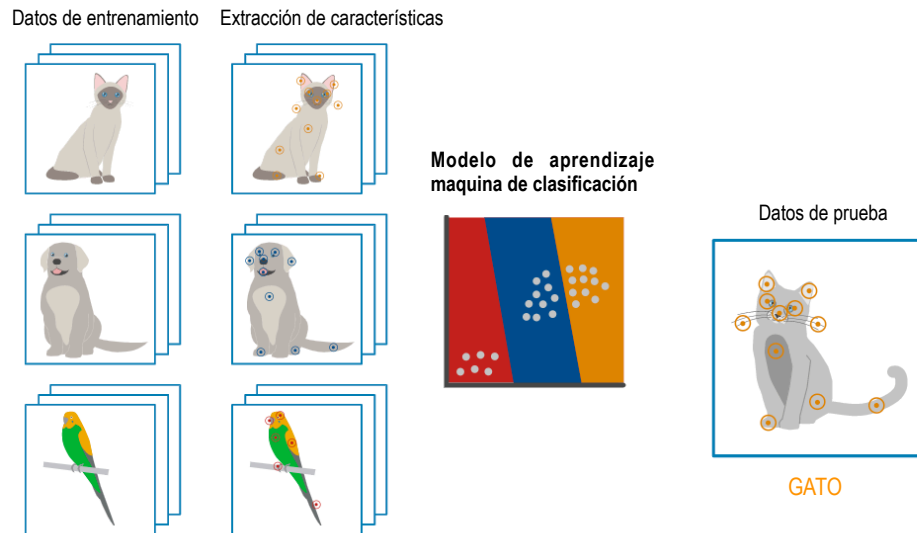
FIGURA 2.6 PROCESO DE CLASIFICACIÓN DE IMÁGENES MEDIANTE CARACTERÍSTICAS Y UN MODELO DE APRENDIZAJE MÁQUINA.
