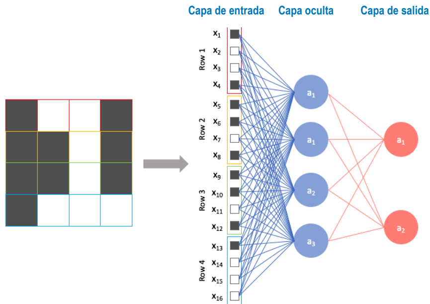
FIGURA 2.18 PROCESAMIENTO DE UNA MATRIZ DE ENTRADA POR PARTE DE UNA CAPA TOTALMENTE CONECTADA. (Figura modificada de [18])
