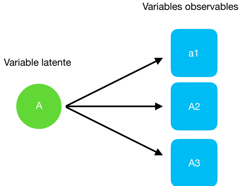
FIGURA 2.21 RELACIÓN ENTRE LAS VARIABLES LATENTES Y LAS VARIABLES OBSERVABLES.
