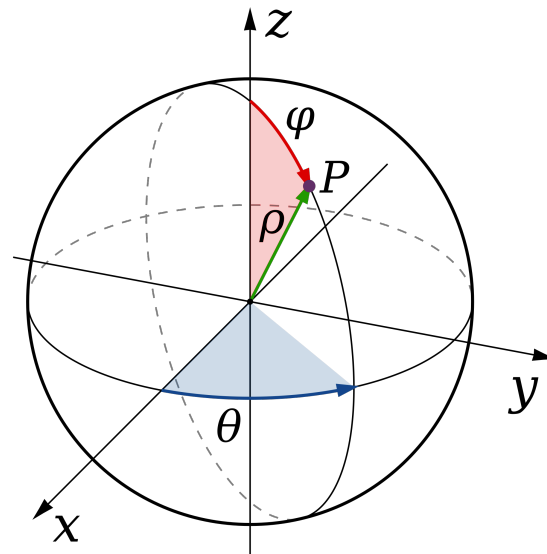
FIGURA 3.3 RELACIÓN ENTRE LAS COORDENADAS ESFÉRICAS Y LAS CARTESIANAS. (Figura tomada de [22])
