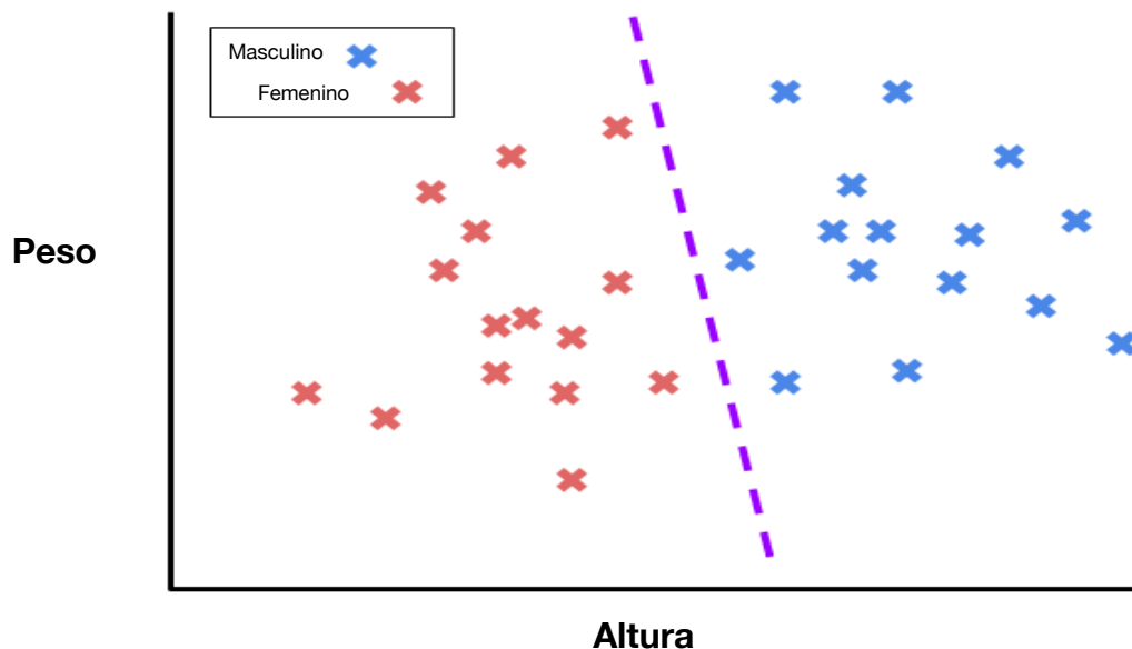
FIGURA 2.10 EJEMPLO DE UN ALGORITMO DE APRENDIZAJE SUPERVISADO. (Figura modificada de [10])
