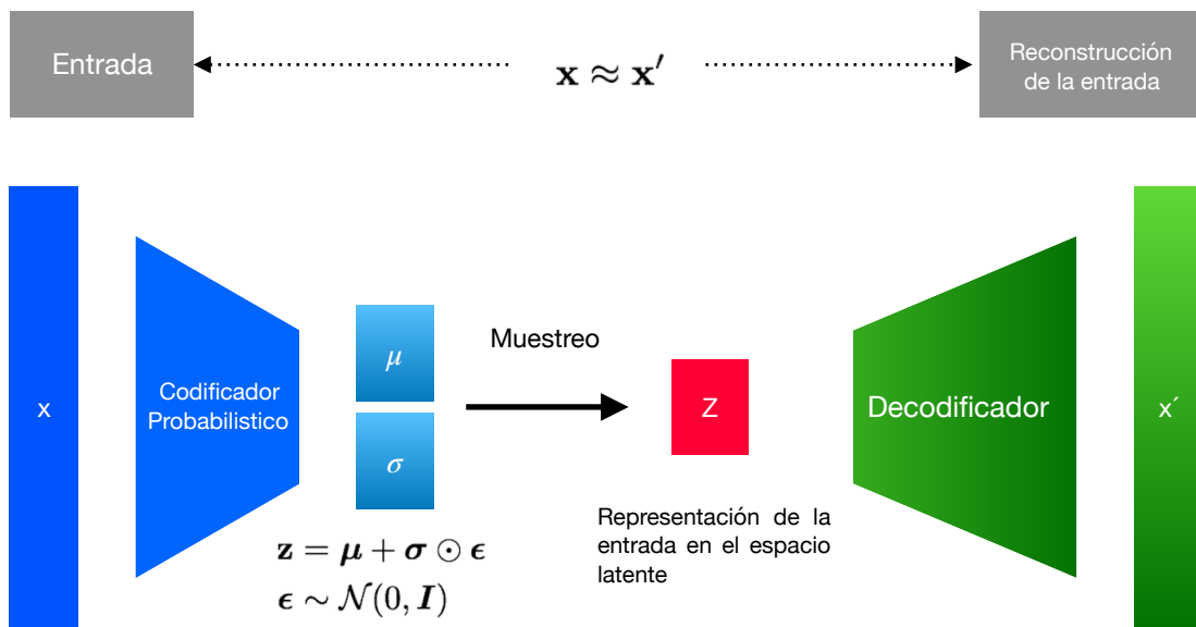
FIGURA 2.23 DETALLE DE LOS BLOQUES Y FUNCIONAMIENTO DE UN AUTOCODIFICADOR VARIACIONAL.
