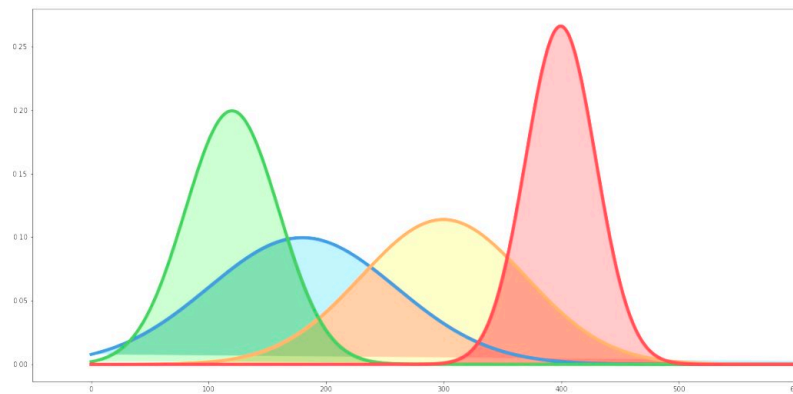
FIGURA 3.6 MÚLTIPLES DISTRIBUCIONES GAUSSIANAS.
