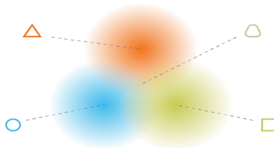
FIGURA 3.7 MUESTREO DESDE LAS DISTRIBUCIONES.
