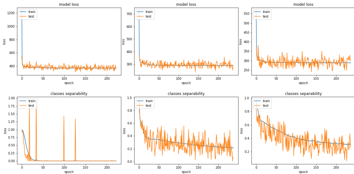
FIGURA 3.10 GRÁFICAS DE LAS FUNCIONES DE PÉRDIDA(SUPERIOR) Y SEPARABILIDAD(INFERIOR) DEL MODELO PARA DIFERENTES ENTRENAMIENTOS DE ESTE SOBRE EL DATASET USANDO DOS CLASES(IZQUIERDA), CINCO CLASES(CENTRO) Y DIEZ CLASES(DERECHA) .
