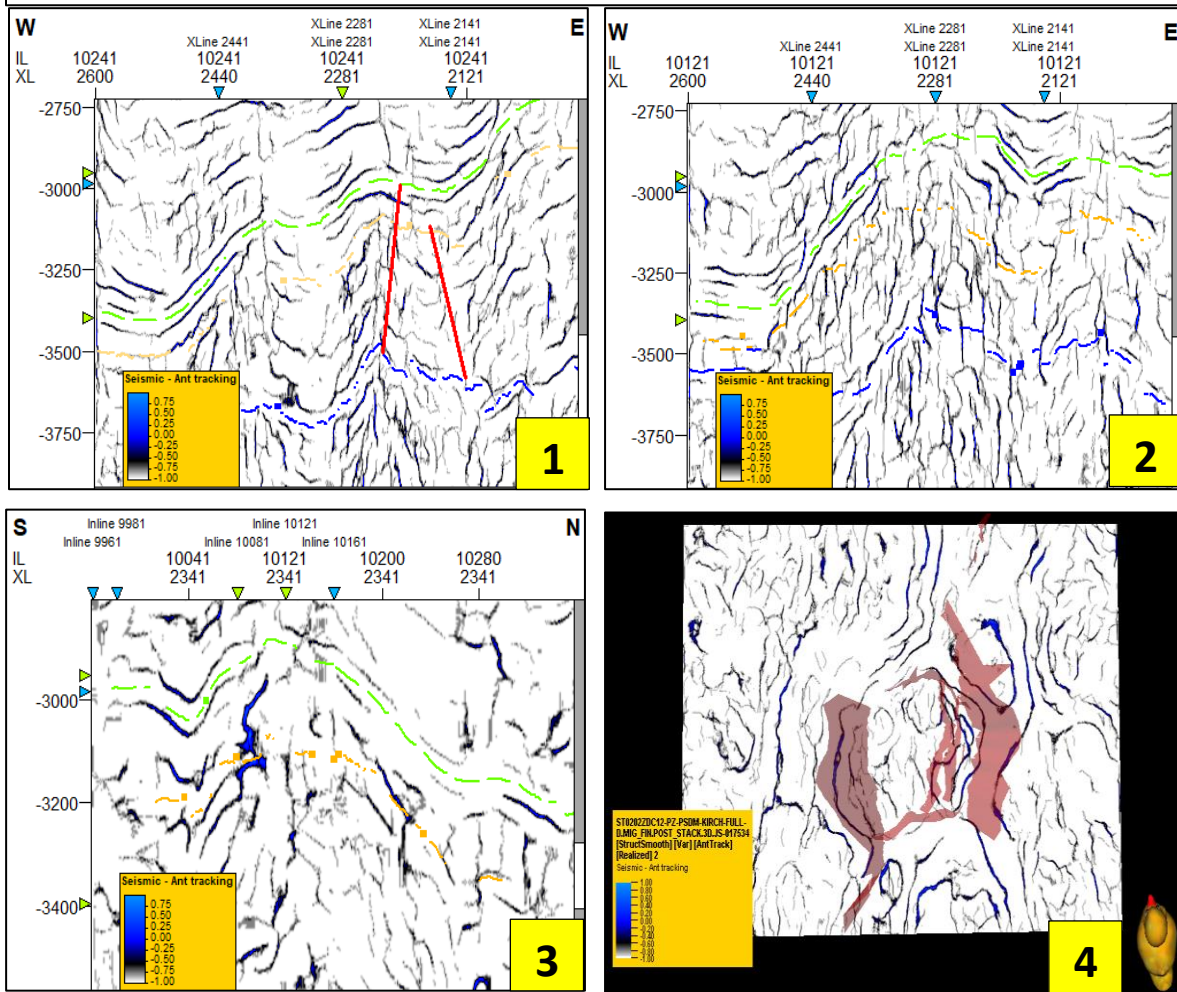
FIGURA 4-7. ATRIBUTO ANT-TRACKING APLICADO A LA SÍSMICA DE VOLVE.
