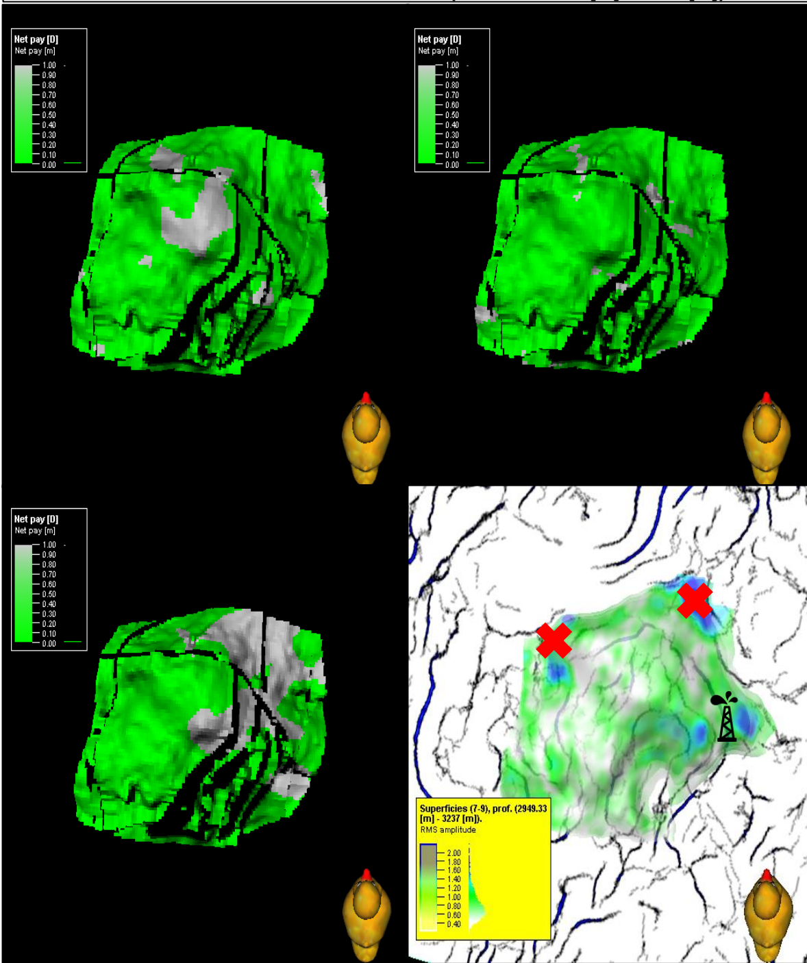
FIGURA 4-16. ANÁLISIS DE FRACTURAMIENTO (PROF. 2949.33 [M] - 3237 [M]).
