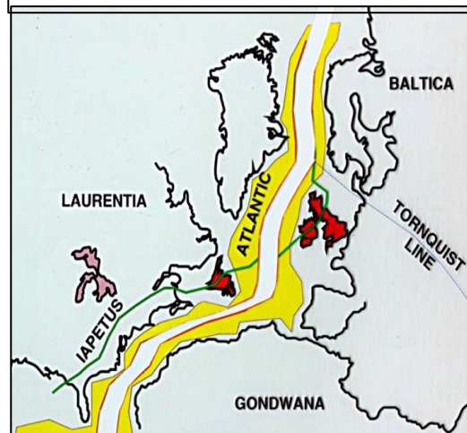
FIGURA 1-14. PROTO-OCÉANO-ATLÁNTICO.
