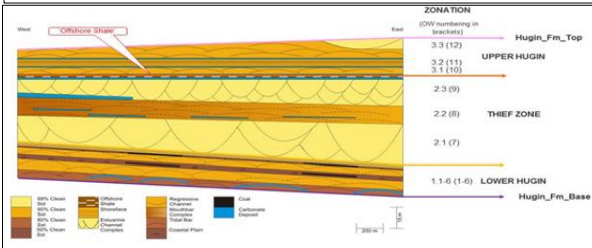
FIGURA 1-20. ESTRATIGRAFÍA DE HUGIN EN EL ÁREA DEL GAMMA HIGH.
