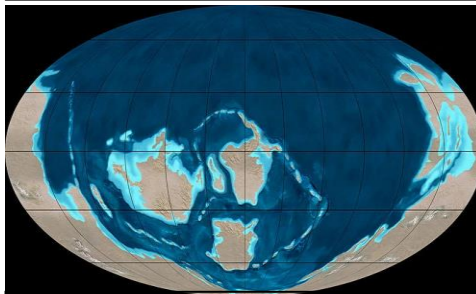
FIGURA 1-9. PLANETA EN EL CÁMBRICO.
