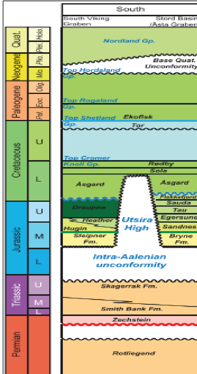
FIGURA 1-18. COLUMNA ESTRATIGRÁFICA DEL SUR DEL MAR DEL NORTE.
