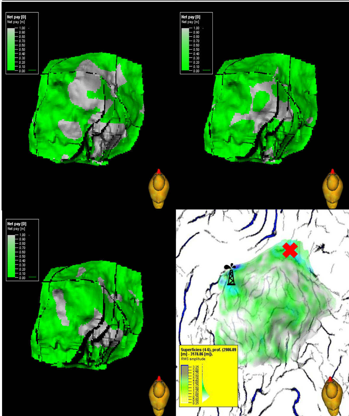
FIGURA 4-15. ANÁLISIS DE FRACTURAMIENTO (PROF. 2906.09 [M] - 3178.86 [M]).
