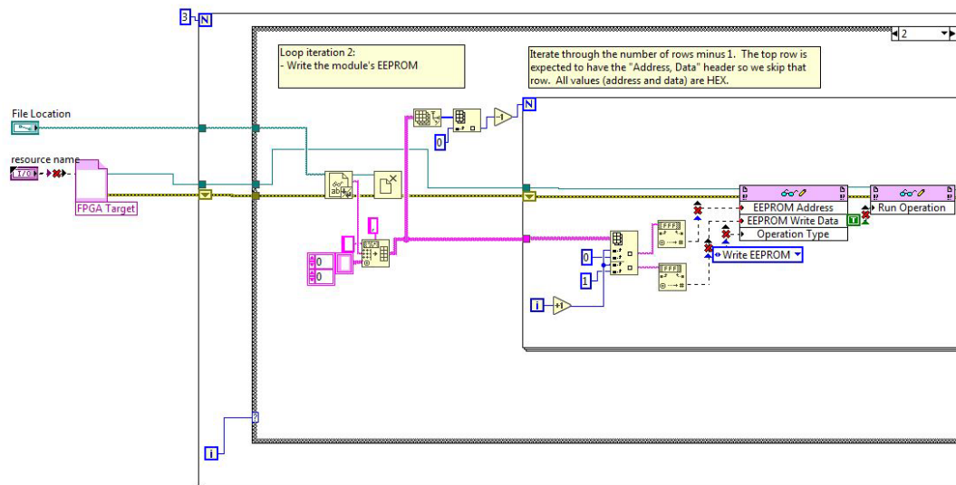
Figura 55. Diagrama de Bloques Del VI – Write EEPROM con errores
