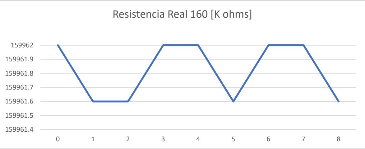
Figura 104. Resultados obtenidos del módulo C teniendo una resistencia de 160 [K ohms] empleando el potenciómetro de precisión
