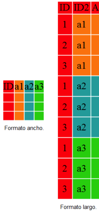
Figura 10: Formatos tidyr. Fuente: https://swcarpentry.github.io/r-novice-gapminder-es/14-tidyr/
