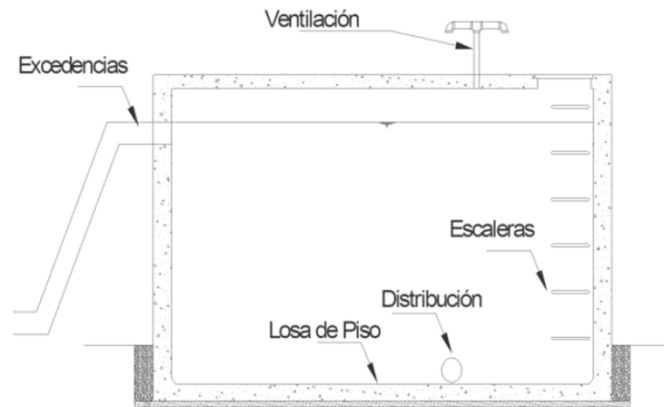
Figura 53. Tanque superficial.
