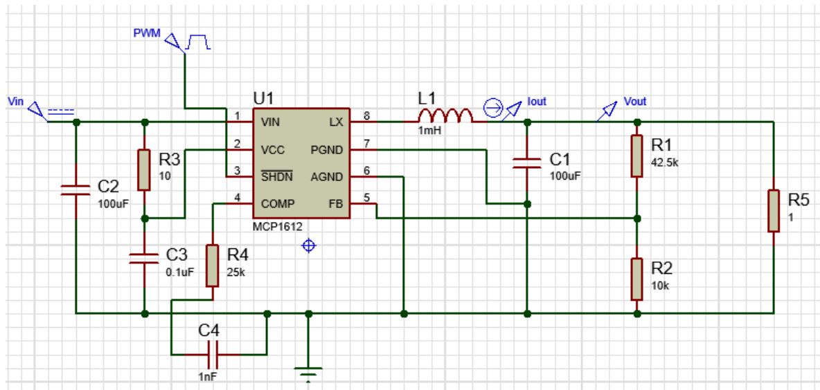
Figura 47. Circuito del convertidor reductor.
