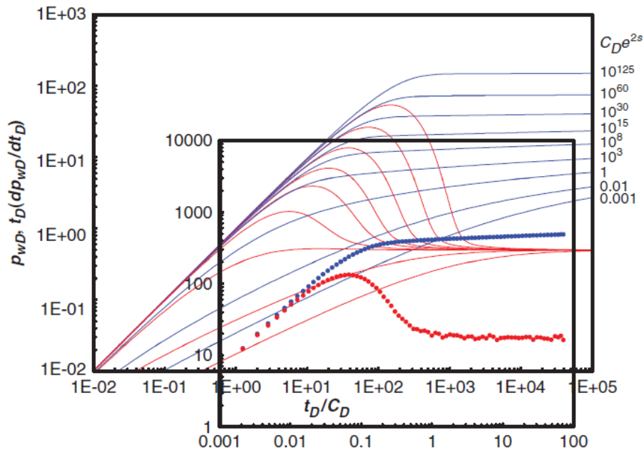
Ilustración 5 Gráfica de datos de campo sobre gráfica de curva tipo. (de Applied Well Test Interpretation, 2013)
