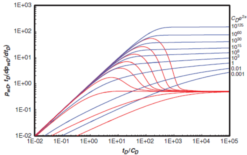
Ilustración 2 Curva tipo de Gringarten-Bourdet para un pozo vertical con un almacenamiento y daño constante en un yacimiento infinito. (de Bourdet et al. 1983)
