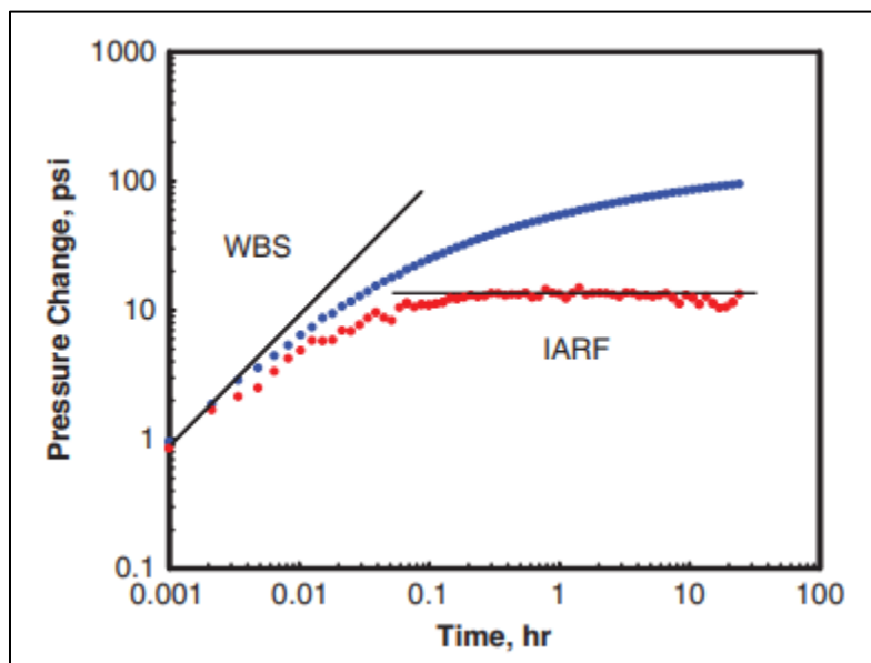
Ilustración 25 Prueba obtenida de un ejemplo de aplicación de Applied Well Test Interpretation , 2013).
