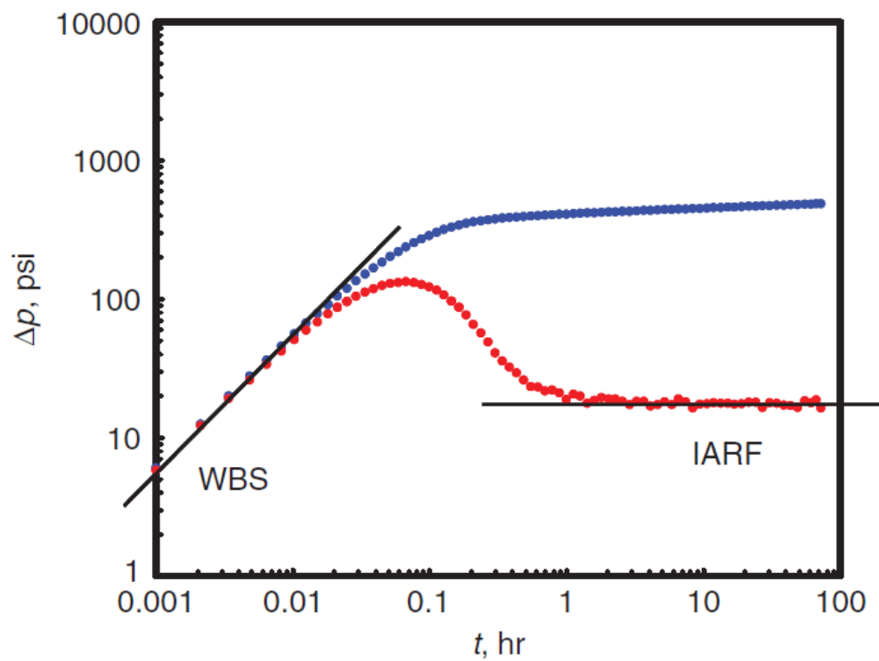
Ilustración 4 Gráfica de datos de campo. (de Applied Well Test Interpretation, 2013)
