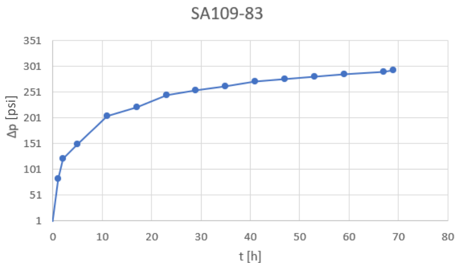
Ilustración 26 Diferencia de presión contra tiempo del pozo SA109 - 83.
