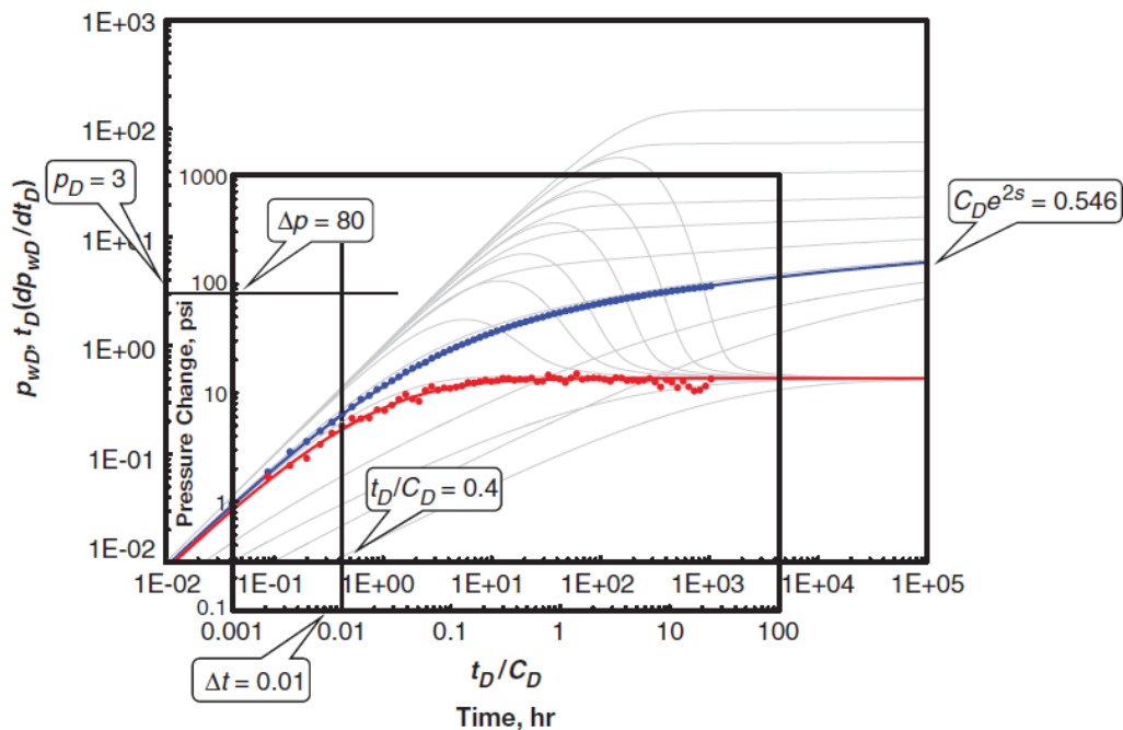
Ilustración 8 Análisis de prueba de incremento. (de Applied Well Test Interpretation, 2013)
