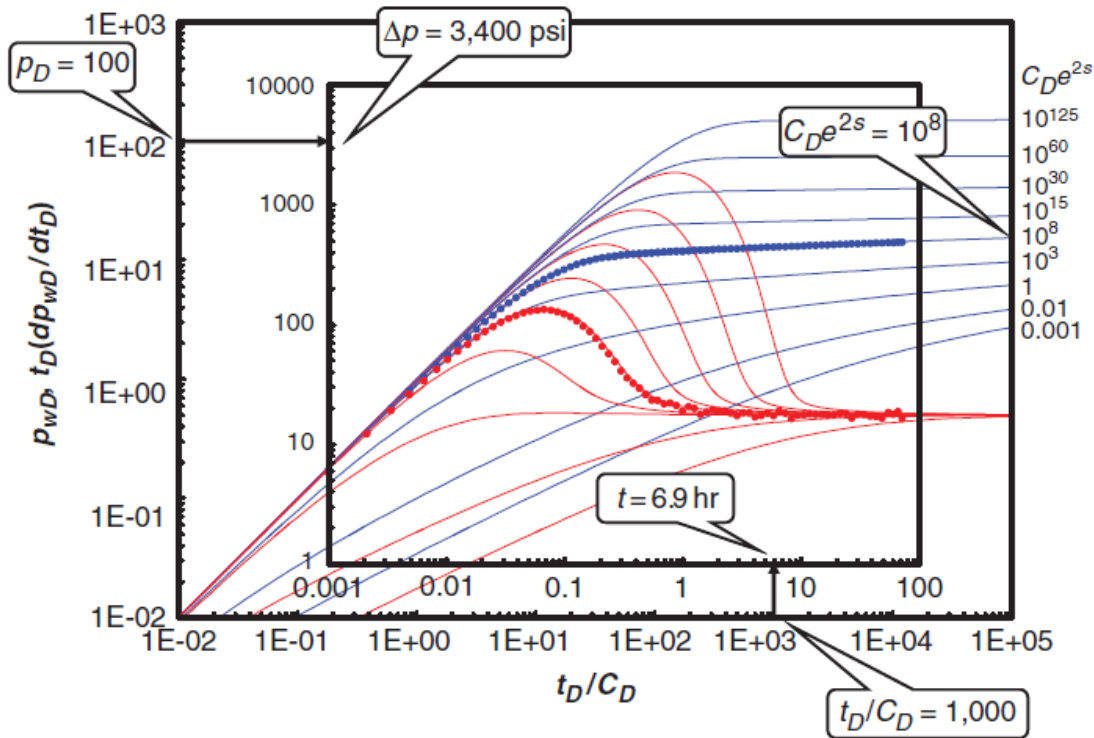
Ilustración 6 Obtención de datos que se alinean entre ambas gráficas. (de Applied Well Test Interpretation, 2013)
