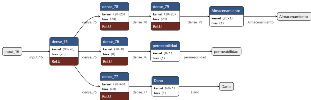
Ilustración 24 Mejor red neuronal del proceso de Grid Search.
