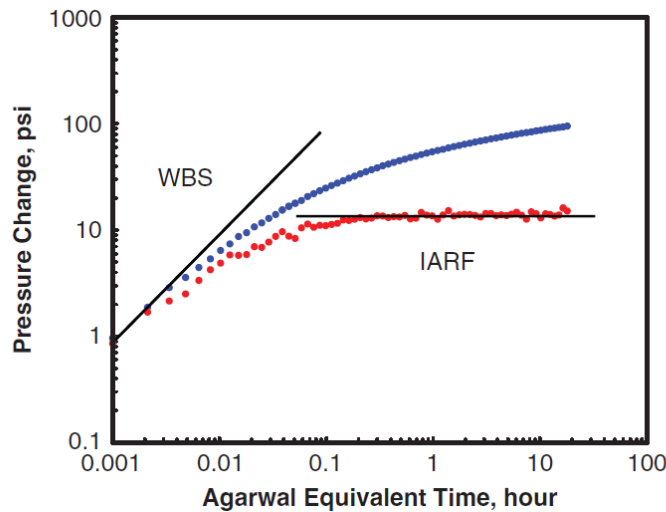
Ilustración 9 Gráfica de datos de campo usando el tiempo equivalente de Agarwal. (de Applied Well Test Interpretation, 2013)
