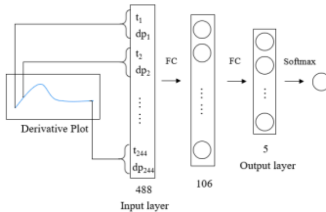
Ilustración 21 Diagrama que representa los datos de entrada en la red neuronal. (de Hongyang Chu et. al.)
