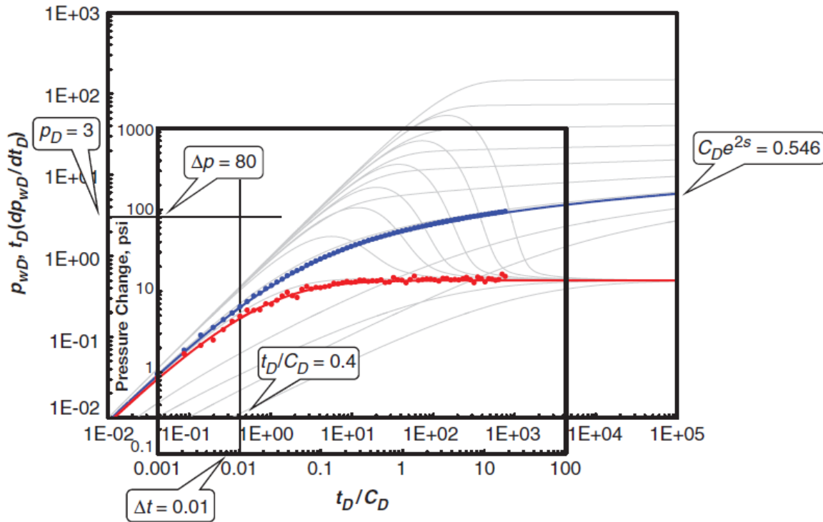
Ilustración 10 Superposición de gráfica de datos de campo sobre gráfica de curvas tipo. (de Applied Well Test Interpretation, 2013)
