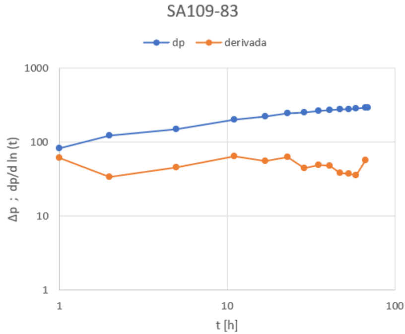
Ilustración 27 Gráfica log-log del pozo SA109 - 83.
