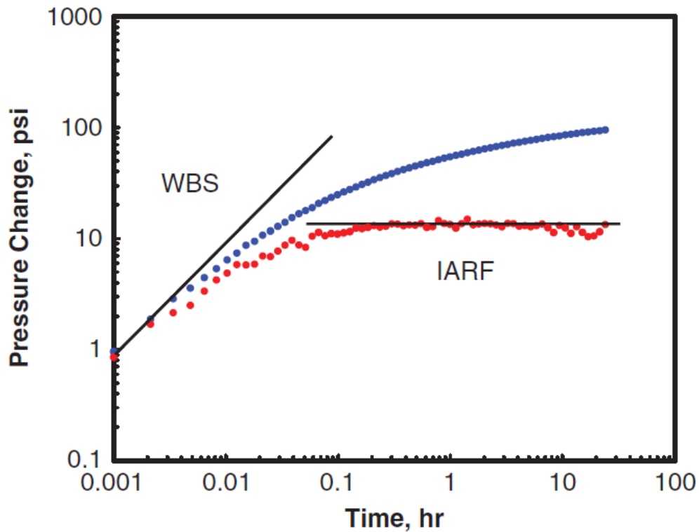
Ilustración 7 Gráfica de datos de campo usando el tiempo de cierre. (de Applied Well Test Interpretation, 2013)
