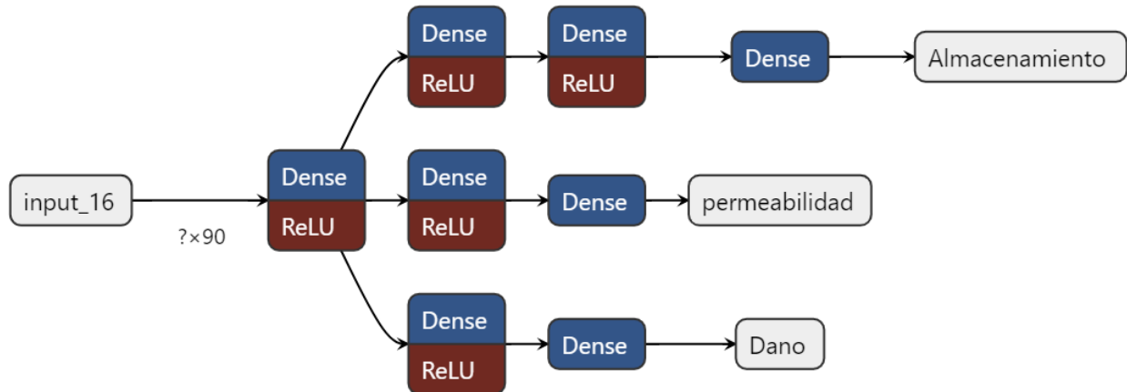
Ilustración 22 Esquema que representa la estructura de la red neuronal construida.
