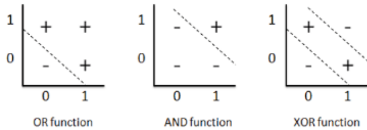
Ilustración 12 Ejemplificación de funciones de clasificación (John Mueller, 2021)
