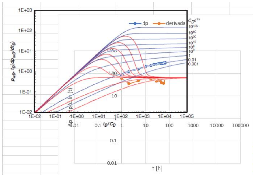
Ilustración 28 Análisis de la prueba del pozo SA109 - 83 con curva tipo Gringarten - Bourdet.
