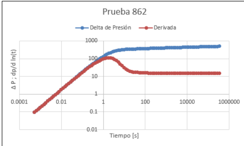
Ilustración 17 Curva generada por nosotros a través de la solución de la ecuación de Gringarten.
