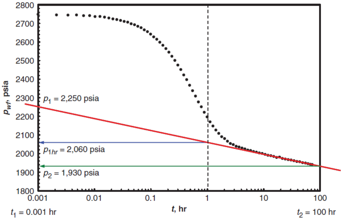
Ilustración 3 Análisis semilogarítmica de una prueba de decremento. (de Applied Well Test Interpretation, 2013)
