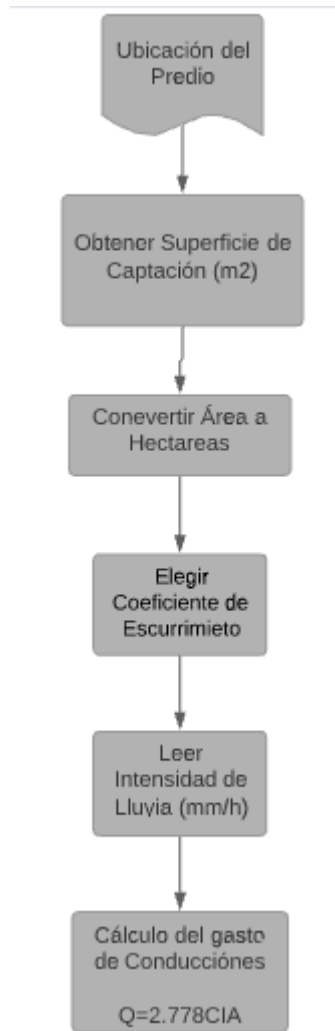
Figura 1 Diagrama de flujo Guía de Elaboración de Sistemas Alternativos, SACMEX.
