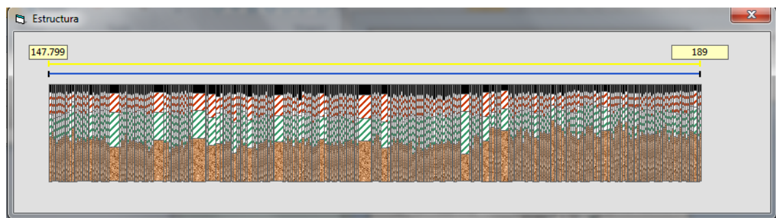
ILUSTRACIÓN 37 ANÁLISIS DE ESPESORES GPR CON EL PROGRAMA ELMOD. FUENTE: ELABORACIÓN PROPIA/YUTAVE
