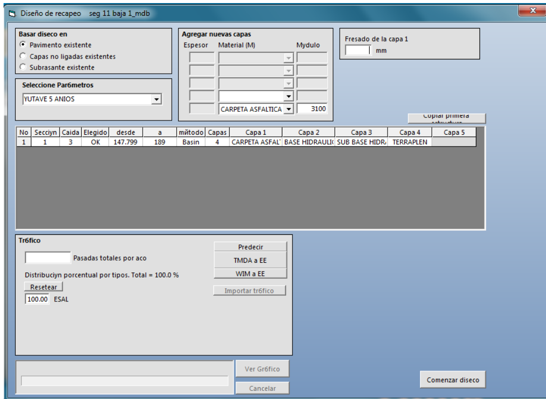
ILUSTRACIÓN 46 REVISIÓN DE LA ESTRUCTURA DEL PAVIMENTO CON EL PROGRAMA ELMOD. FUENTE: ELABORACIÓN PROPIA/YUTAVE
