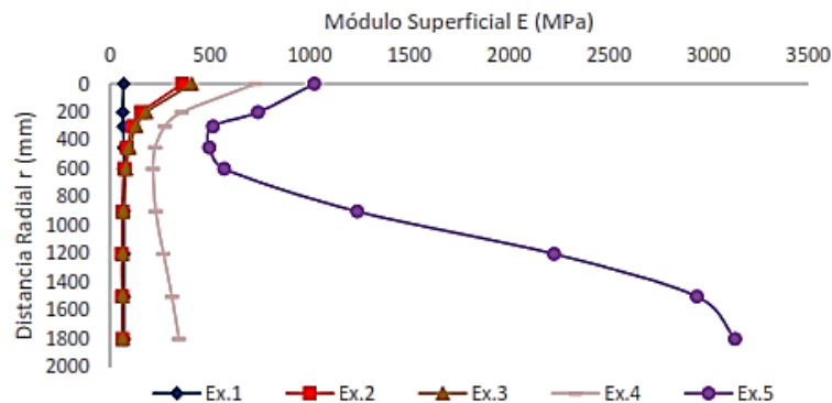
ILUSTRACIÓN 30 EJEMPLOS DE GRÁFICOS DE MÓDULO SUPERFICIAL; FUENTE: (BAZI, 2012).
