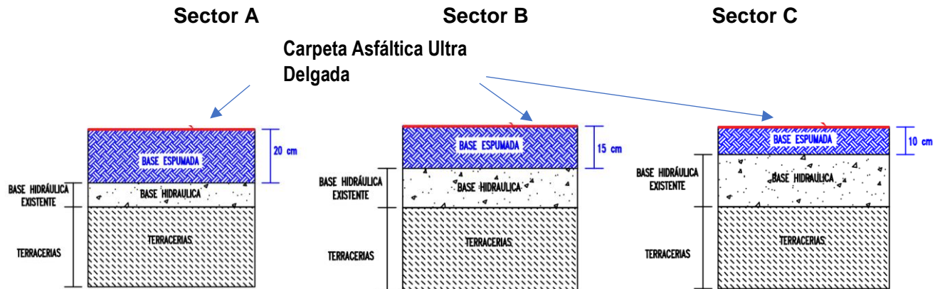
ILUSTRACIÓN 81.- SECTORES PARA EL TRATAMIENTO PROFUNDO. FUENTE: ELABORACIÓN PROPIA
