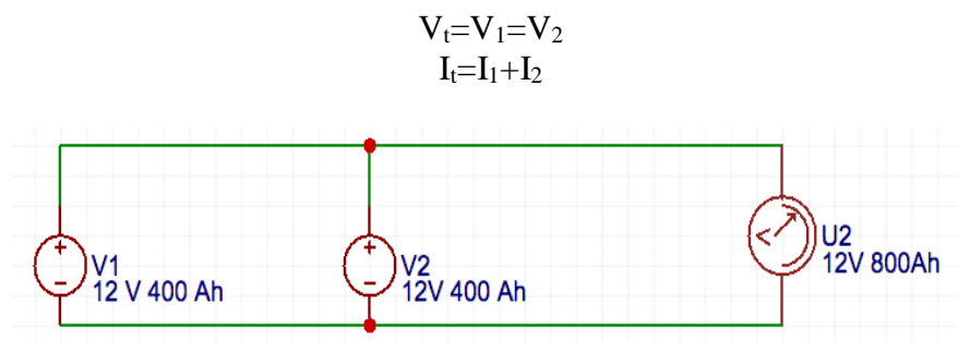
Figura 1- 18 Conexión en paralelo de dos baterías idénticas.
