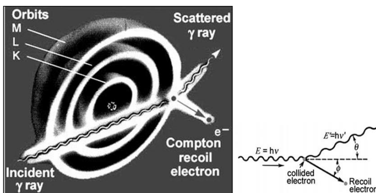
Figura 1.7. Esquema del proceso de Compton y las relaciones geométricas en dicho proceso (cortesía de Schlumberger). Recuperado de Serra, O. (2008).
