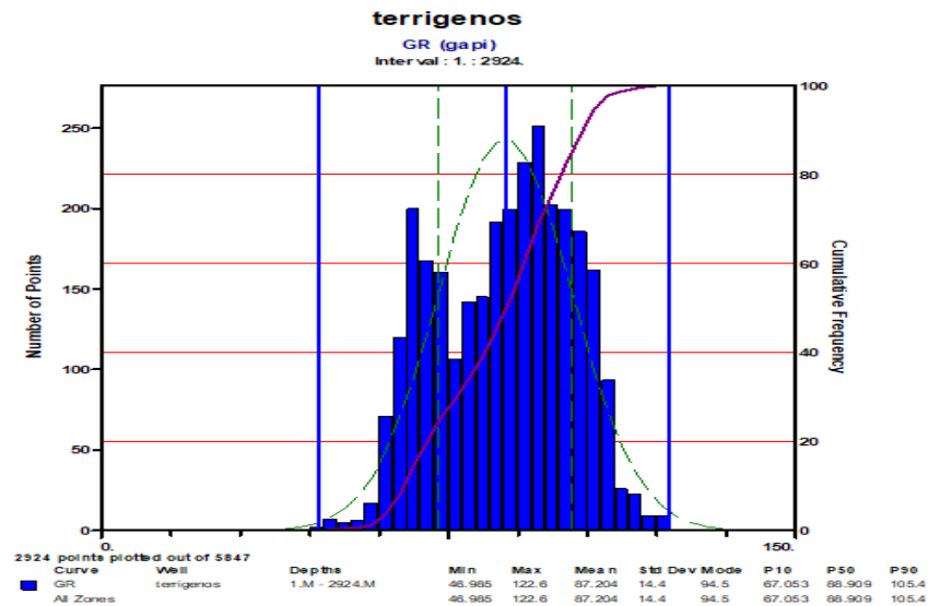
Figura 3.2. Histograma del registro de Rayos Gamma del pozo Terrígeno-1.
