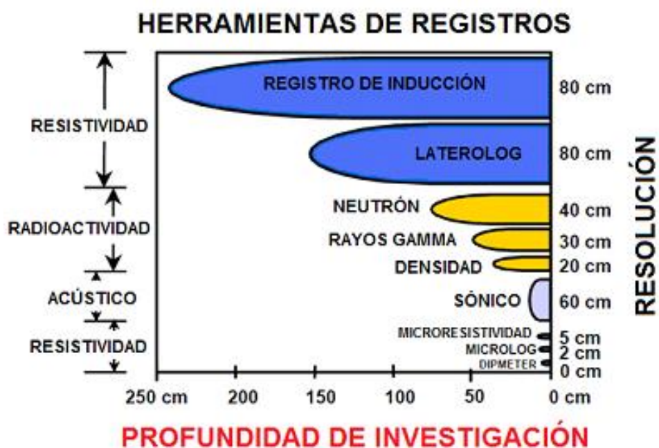
Figura 1.11. Diagrama comparativo de las diferentes herramientas en la toma de registros mostrando las diferentes propiedades físicas, su resolución vertical y la profundidad de investigación con la que trabajan (IMP,2019).
