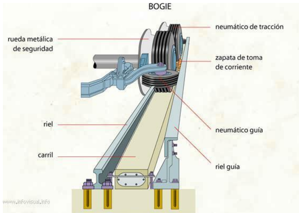
Ilustración 27. Esquema de funcionamiento de bogie con rieles electrificados. https://infovisual.info/es/transporte/bogie
