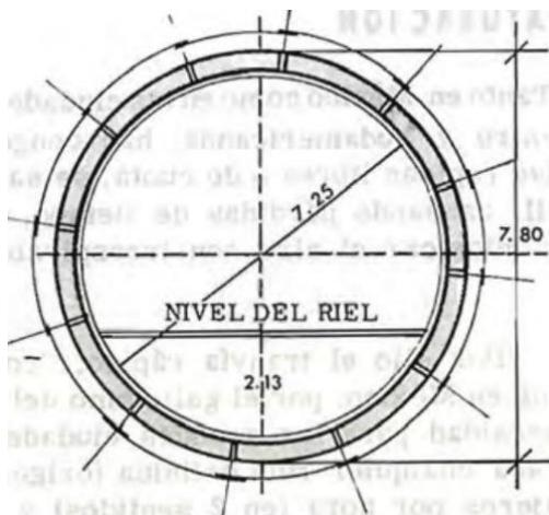
Ilustración 15. Túnel excavado en forma de escudo. Fuente: Ferrocarriles, por Ing. Francisco M Tognó; Facultad de Ingeniería.
