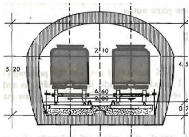
Ilustración 16. Túnel convencional de trenes de pasajeros. Fuente: Ferrocarriles, por Ing. Francisco M Tognó; Facultad de Ingeniería.
