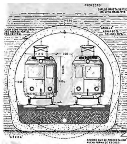
Ilustración 18. Sección tipos de túneles para F.C. subterráneo electrificado con doble vía en CDMX, Julio de 1963. Fuente: Ferrocarriles, por Ing. Francisco M Togno; Facultad de Ingeniería.
