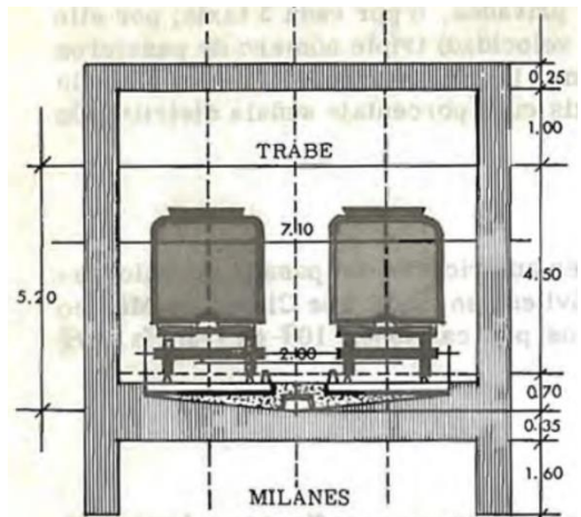
Ilustración SEQ Ilustración \* ARABIC 17. Túnel en forma de caja por Milanes. Fuente: Ferrocarriles, por Ing. Francisco M Togno; Facultad de Ingeniería.
