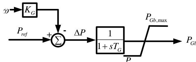
Figura 2.10 Modelo del gobernador de velocidad de una central termoeléctrica
