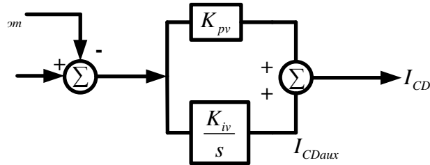
Figura 2.21 Control de voltaje de CD en el inversor
