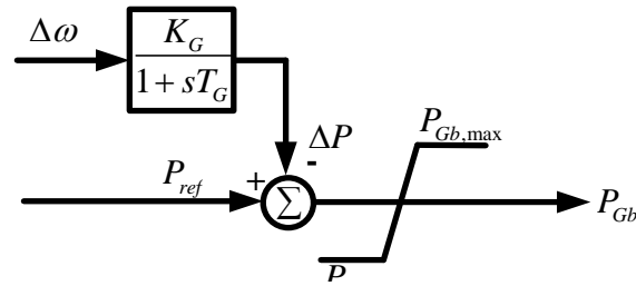
Figura 2.11 Modelo del gobernador de velocidad de la central hidroeléctrica
