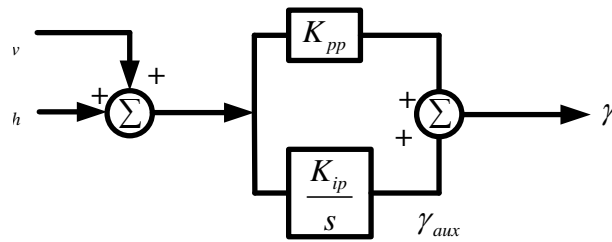
Figura 2.20 Control de potencia activa en el rectificador
