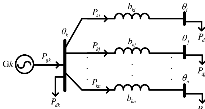
Figura 3.2 Nodo genérico de un SEP de CA
