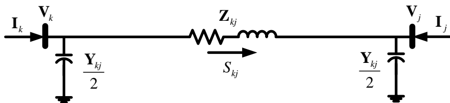
Figura 2.1 Modelo \pi de la línea de transmisión
