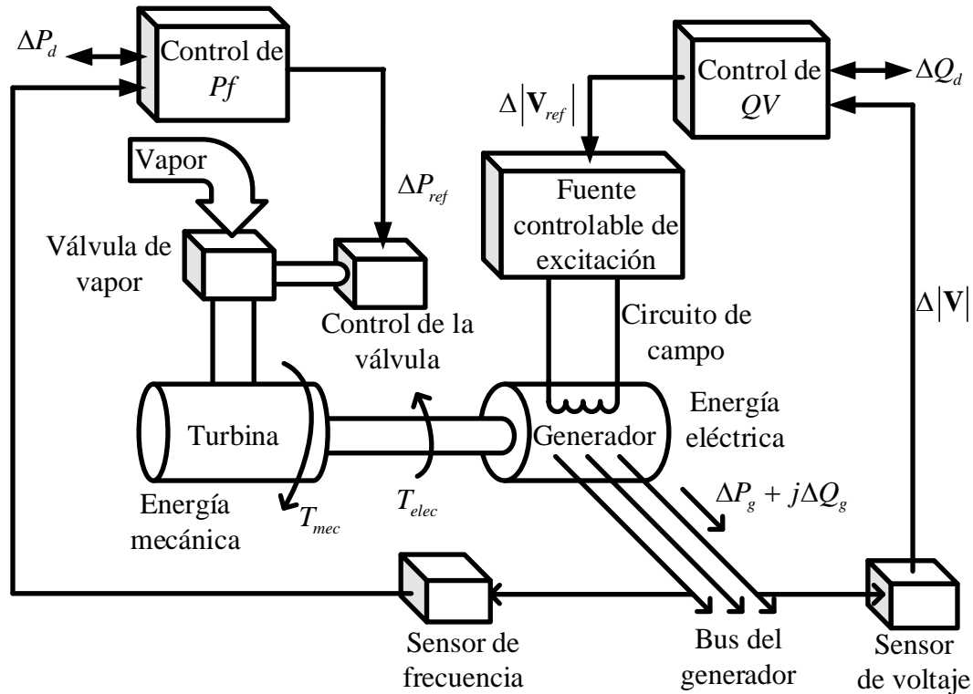
Figura 2.6 Unidad de generación con controles de voltaje y frecuencia [29]
