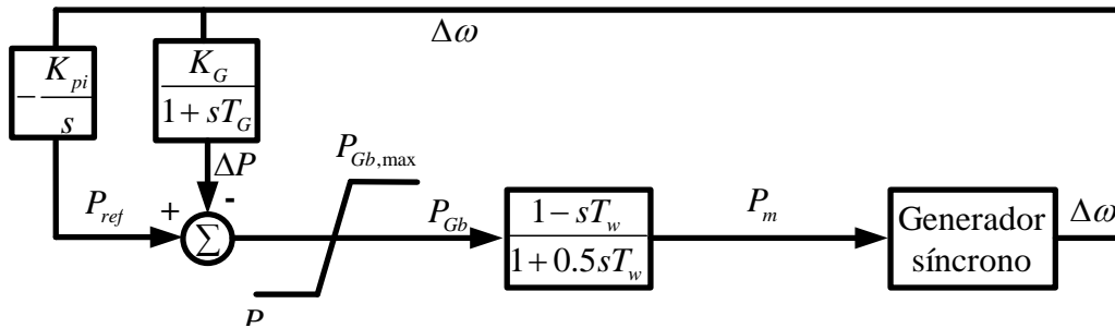
Figura 2.14 Diagrama de bloques de una planta hidroeléctrica
