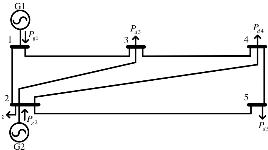
Figura 4.1 Red de 5 nodos de IEEE [52]
