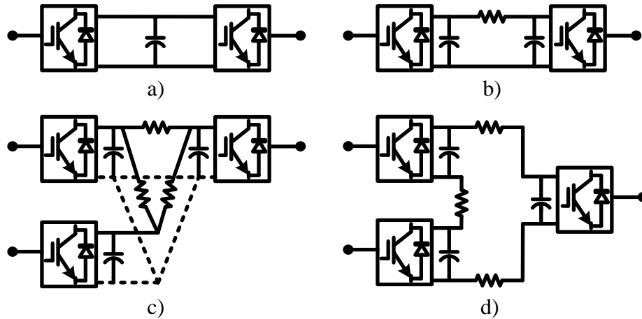
Figura 1.2 Configuraciones de los sistemas VSC-HVDC, a) Back-to-back , b) Point-to-point , c) Multiterminal paralelo y c) Multiterminal serie
