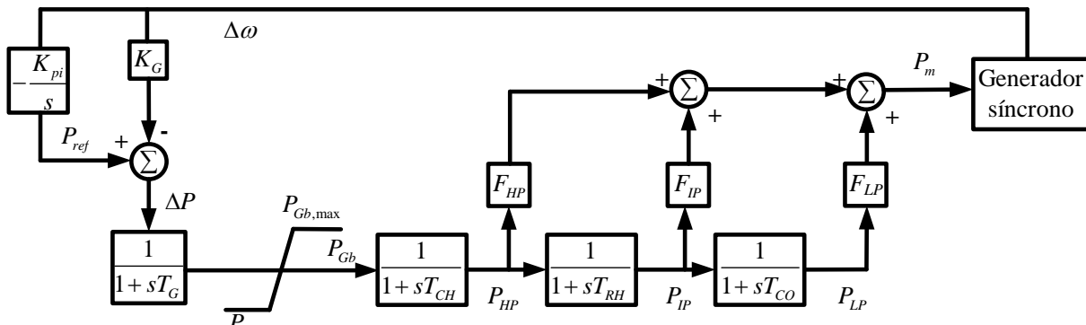
Figura 2.13 Diagrama de bloques de una central termoeléctrica
