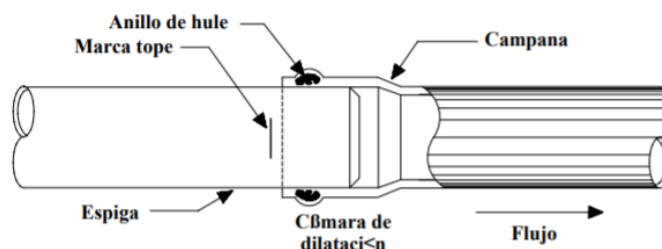
Figura 2.1. Unión espiga-campana en tuberías de PVC 18
