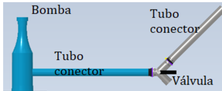
Figura 5.23. Bomba, válvula y conector a caja de WC.
