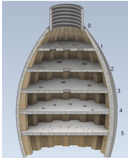
Figura 5.24. Reducciones de área para el cabezal.
