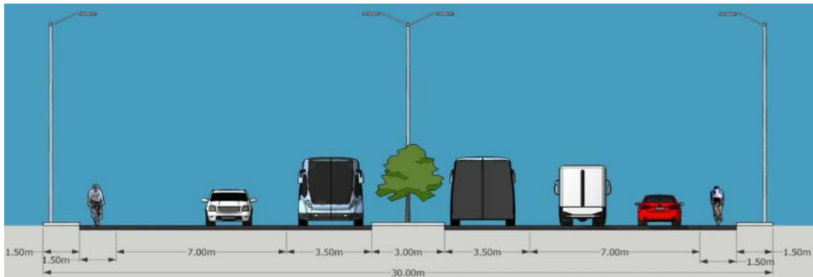
Figura 27. Sección tipo del corredor vial en prolongación 20 de noviembre y avenida Eucaliptos (Elaboración propia, 2021).
