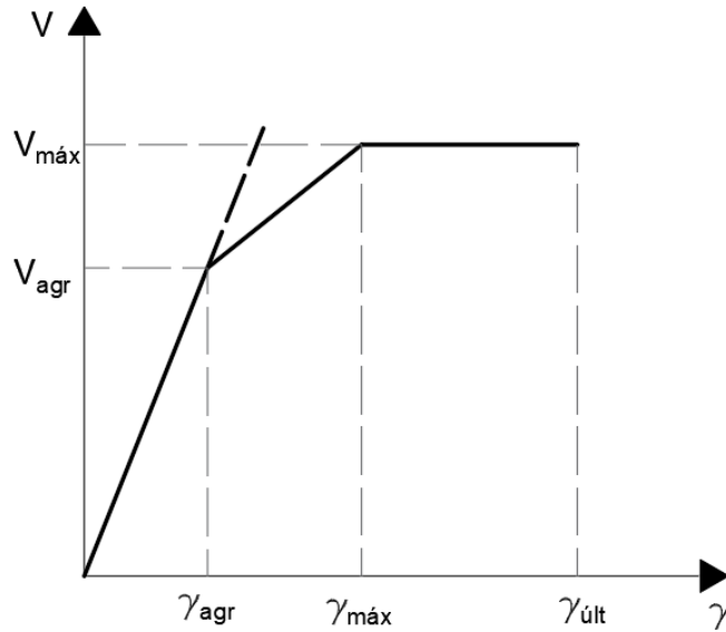
Figura 2.9. Curva trilineal propuesta por Meli (adaptada de [ 10 ]).
