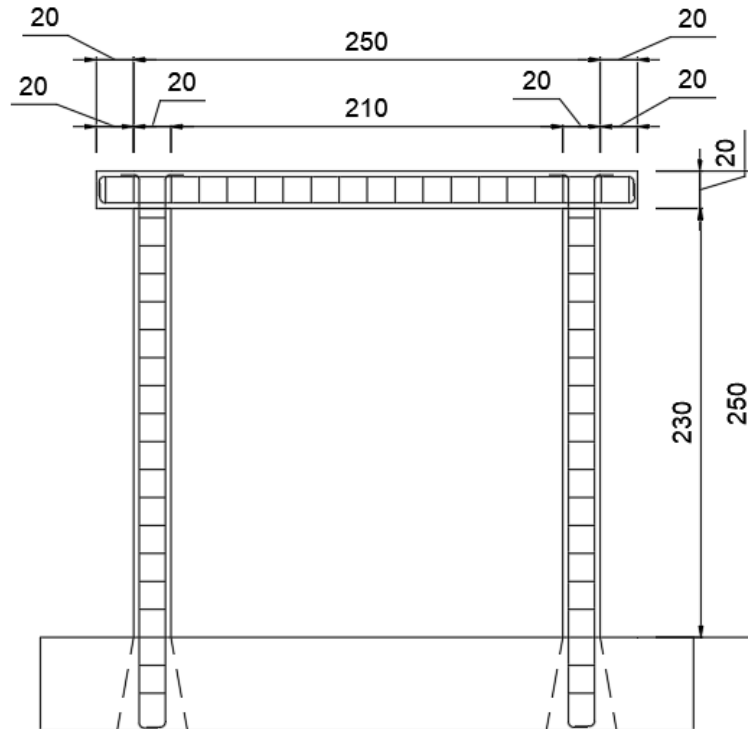
Figura 3.4. Armado general del muro de prueba (dimensiones en cm).
