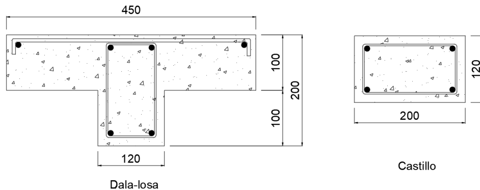
Figura 3.5. Detalles típicos de dala-losa y castillo (dimensiones en mm).
