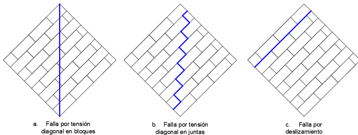
Figura 2.5. Fallas en ensayos de muretes a compresión diagonal (adaptada de [ 9 ])
