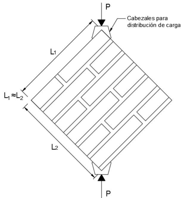
Figura 2.4. Ensayo de compresión diagonal (adaptada de [ 10 ]).
