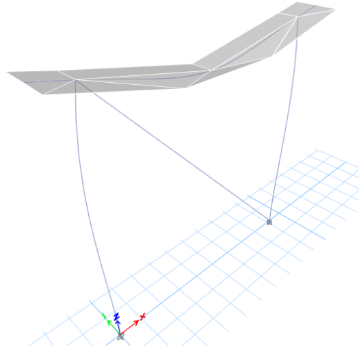
Figura 4.5. Diagonal equivalente.
