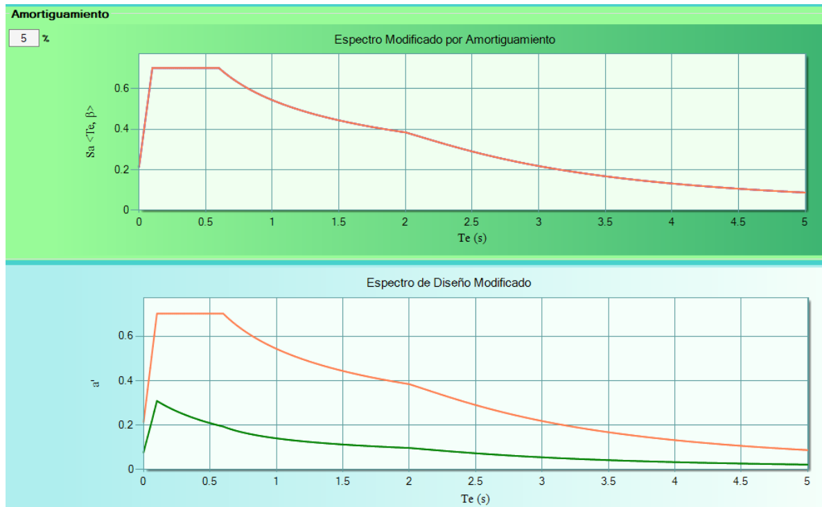
Figura 5.3. Espectros elástico y de diseño.
