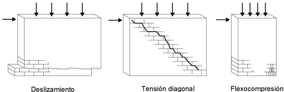
Figura 2.7. Fallas en muros de mampostería confinados (adaptada de [ 1 ]).
