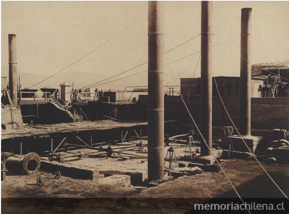
Calderos y acendreras de la Oficina Salitrera de Agua Santa, 1889.
