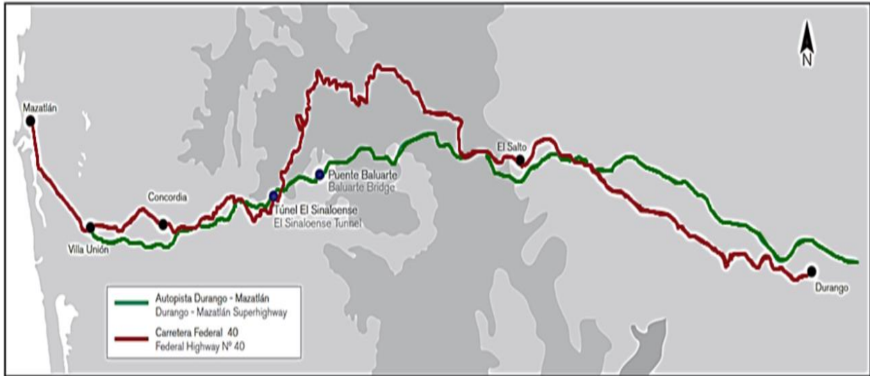
Figura 4 Carretera Durango-Mazatlán (Poon, 2012).
