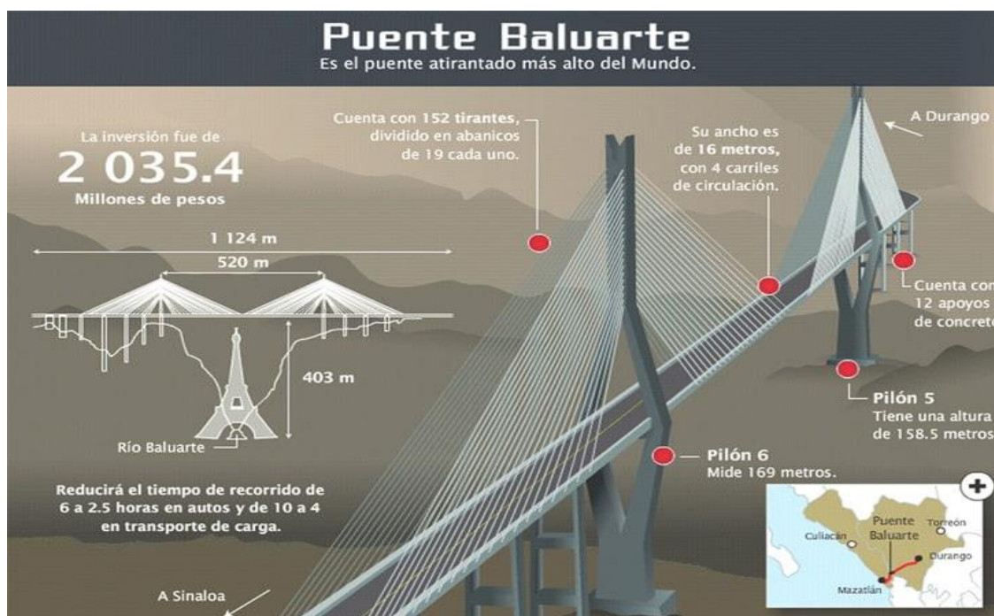
Figura 6 Características del Puente Baluarte (Durango Oficial, 2019).
