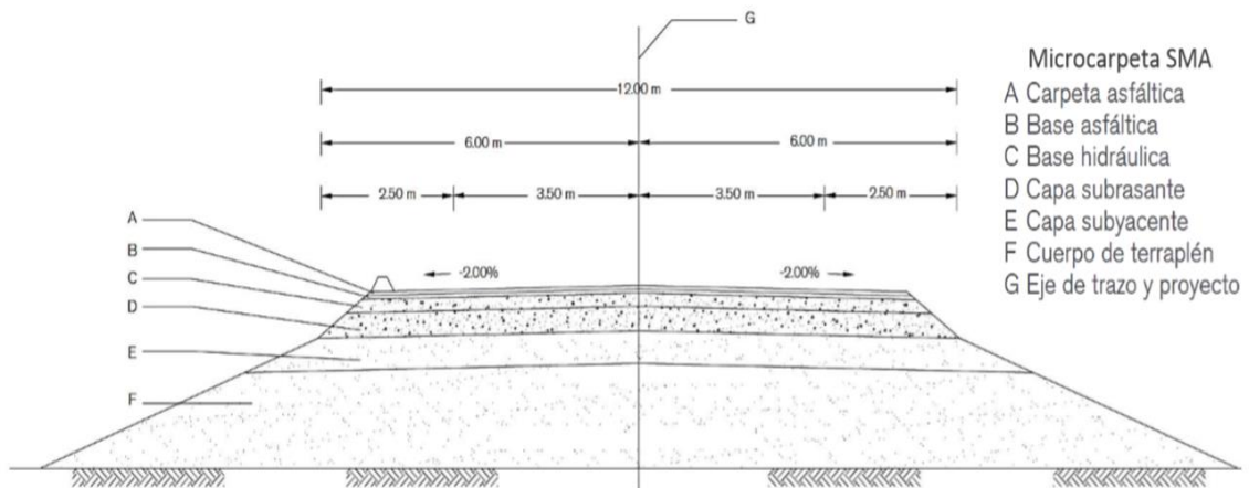
Figura 5 Estructura de Pavimento Carretera Durango-Mazatlán (Poon, 2012).
