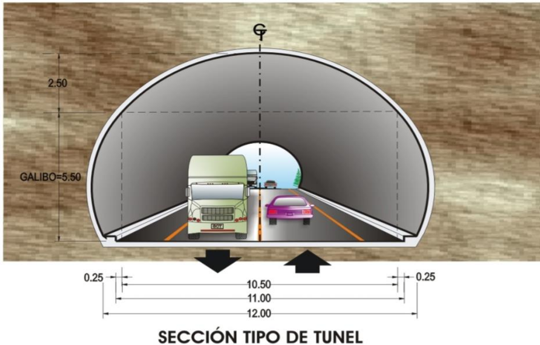
Figura 7 Sección tipo de los túneles de la carretera (Poon, 2012).
