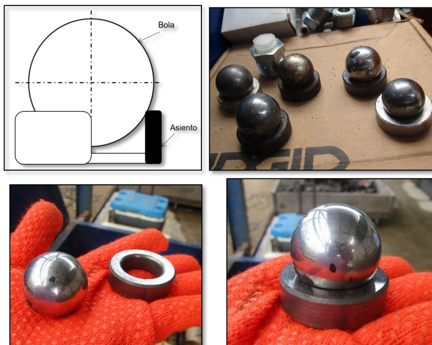
Figura 2.17 Bola y asiento de las válvulas
