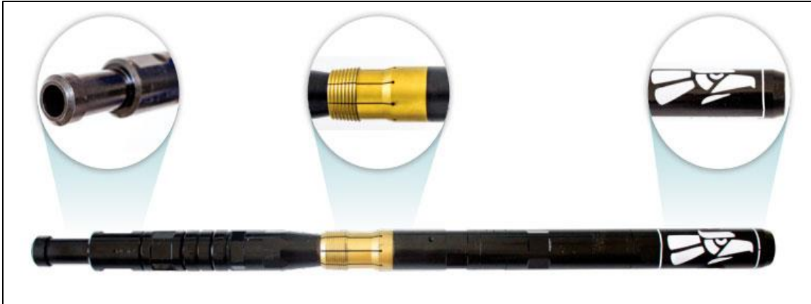
Figura 1.17 Estrangulador de fondo tipo Venturi
