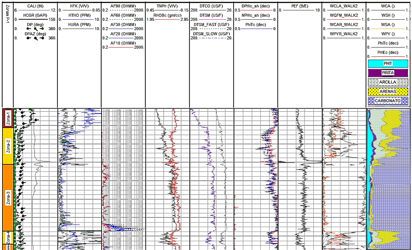
Figura 7. Despliegue de registros del Pozo-1.
