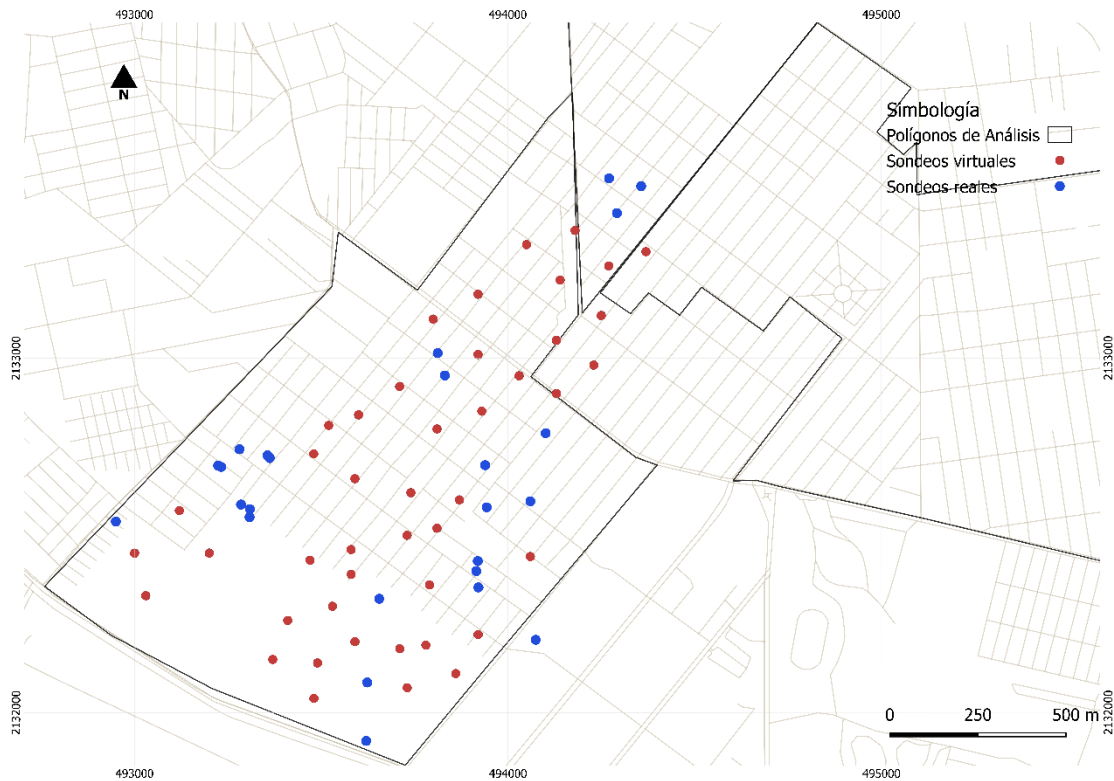
Figura 3. 28 Ubicación de los sondeos virtuales y reales.
