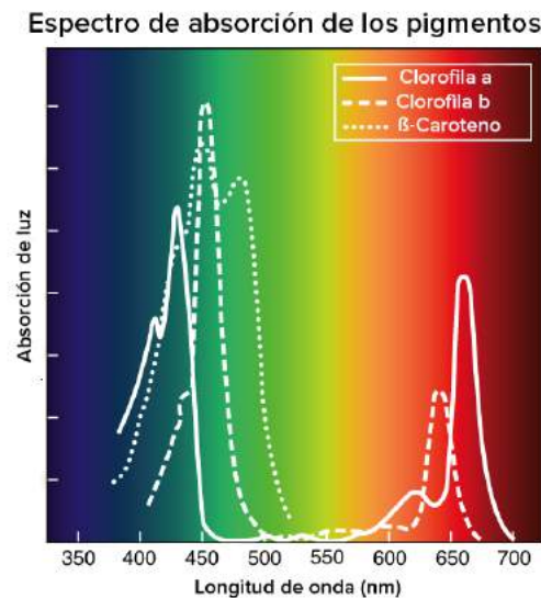
Figura 4.2: Espectro de absorbancia de la clorofila a, clorofila b y betacaroteno [29].
