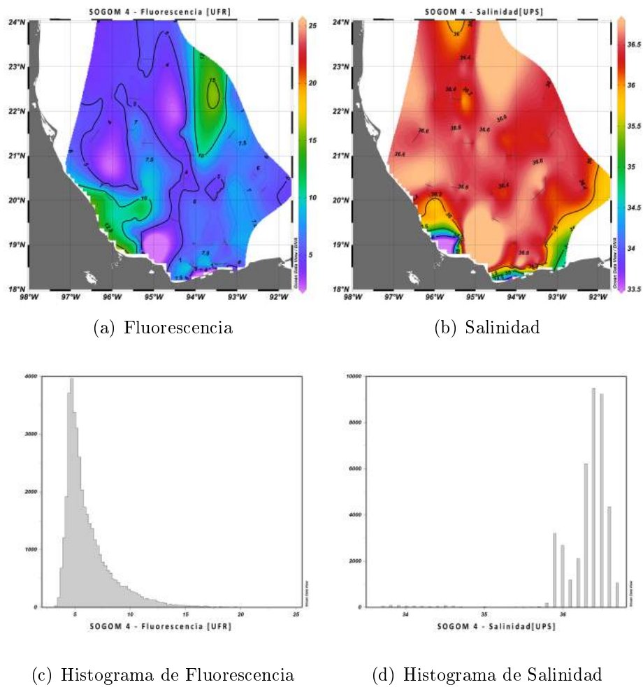
Figura A.9: SOGOM 4 Mapa e histograma de Fluorescencia y Salinidad (Transito de Noche)
