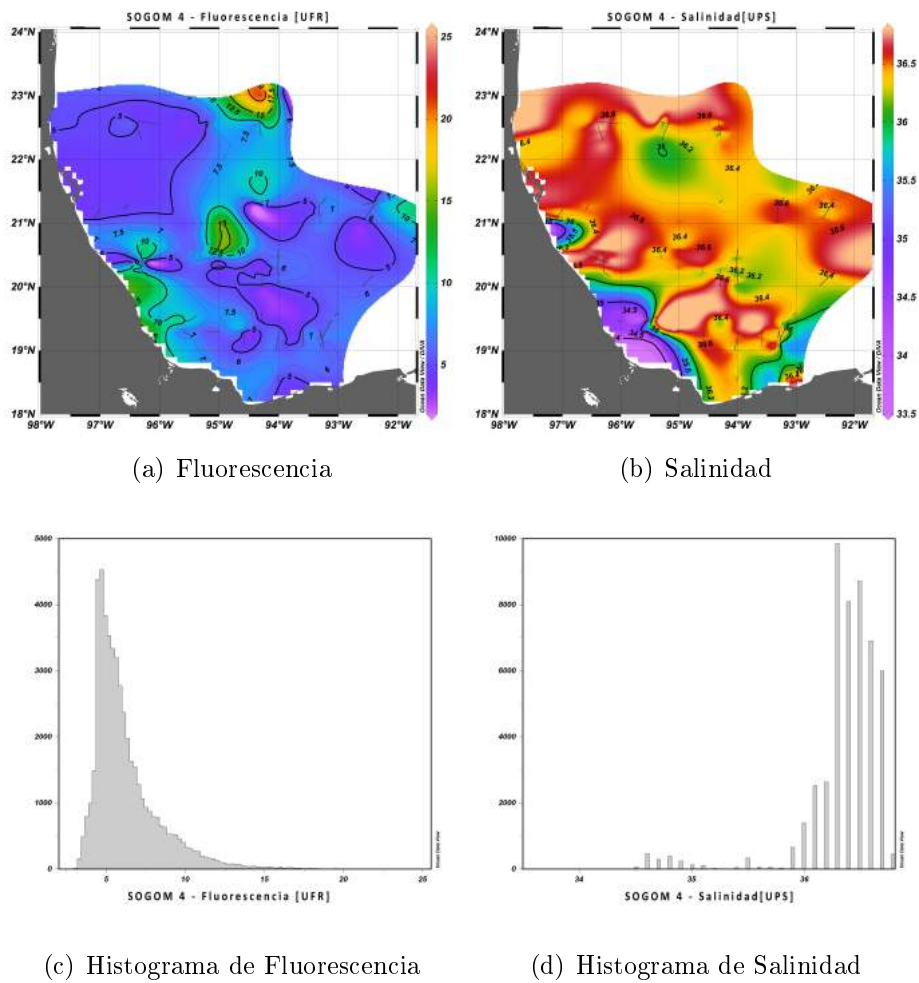
Figura A.5: SOGOM 4 Mapa e histograma de Fluorescencia y Salinidad (Transito de Día)
