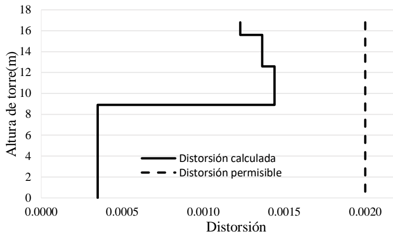
Figura 4.23. Comparación de las distorsiones calculadas y las permitidas para estado límite de servicio en dirección transversal
