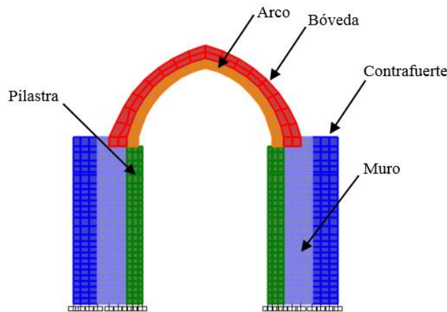
Figura 4.4. Sección E del modelo numérico
