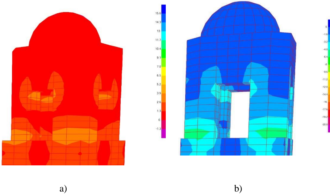
Figura 4.17. Esfuerzos axiales ( S_{33} ) en campanarios: a) Esfuerzos de tensión, b) Esfuerzos en compresión (en \text{kg/cm}^2 )
