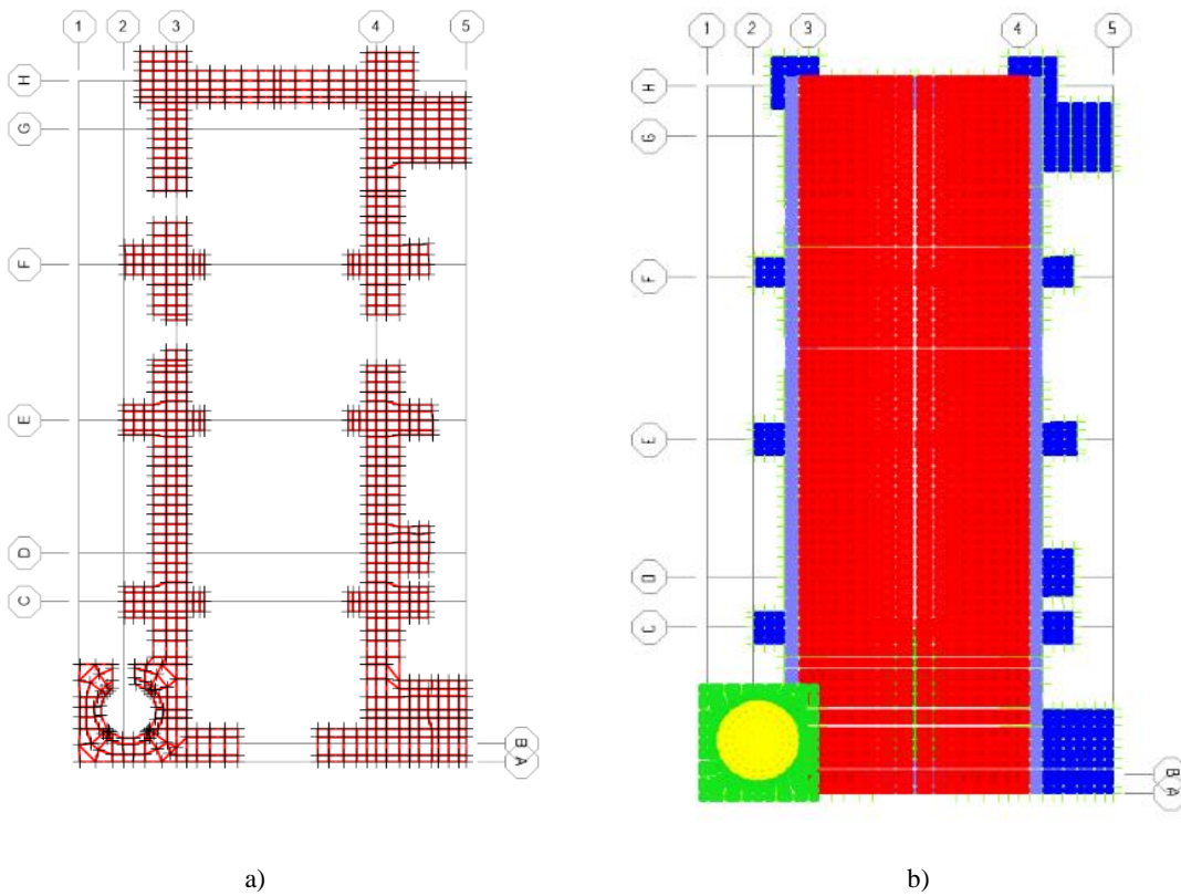
Figura 4.2. Planta del modelo numérico: a) Ejes de referencia en la base b) Vista en planta hasta altura de muros
