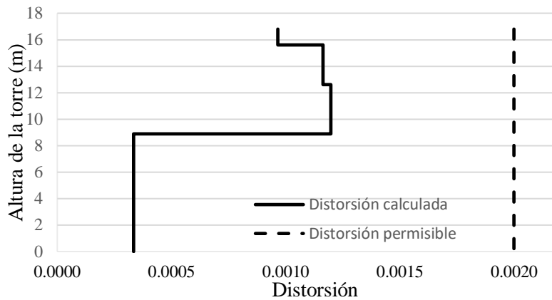
Figura 4.24. Comparación de las distorsiones calculadas y las permitidas para estado límite de servicio en dirección longitudinal
