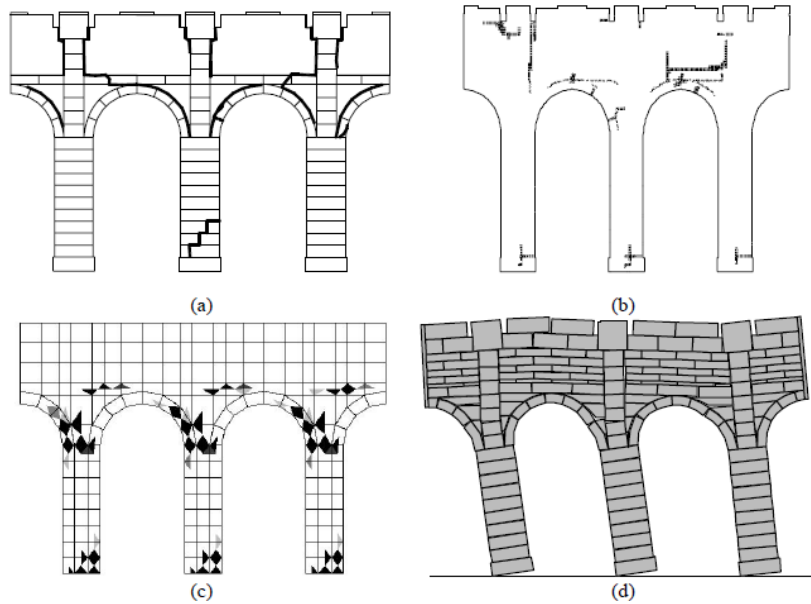
Figura 2.14. Patrones de agrietamiento: a) agrietamiento en el modelo experimental, b) MEF, deformaciones plásticas principales mayores, c) MER, daño por tensión, y d) ALBR, mecanismo de colapso (Orduña et al., 2007)
