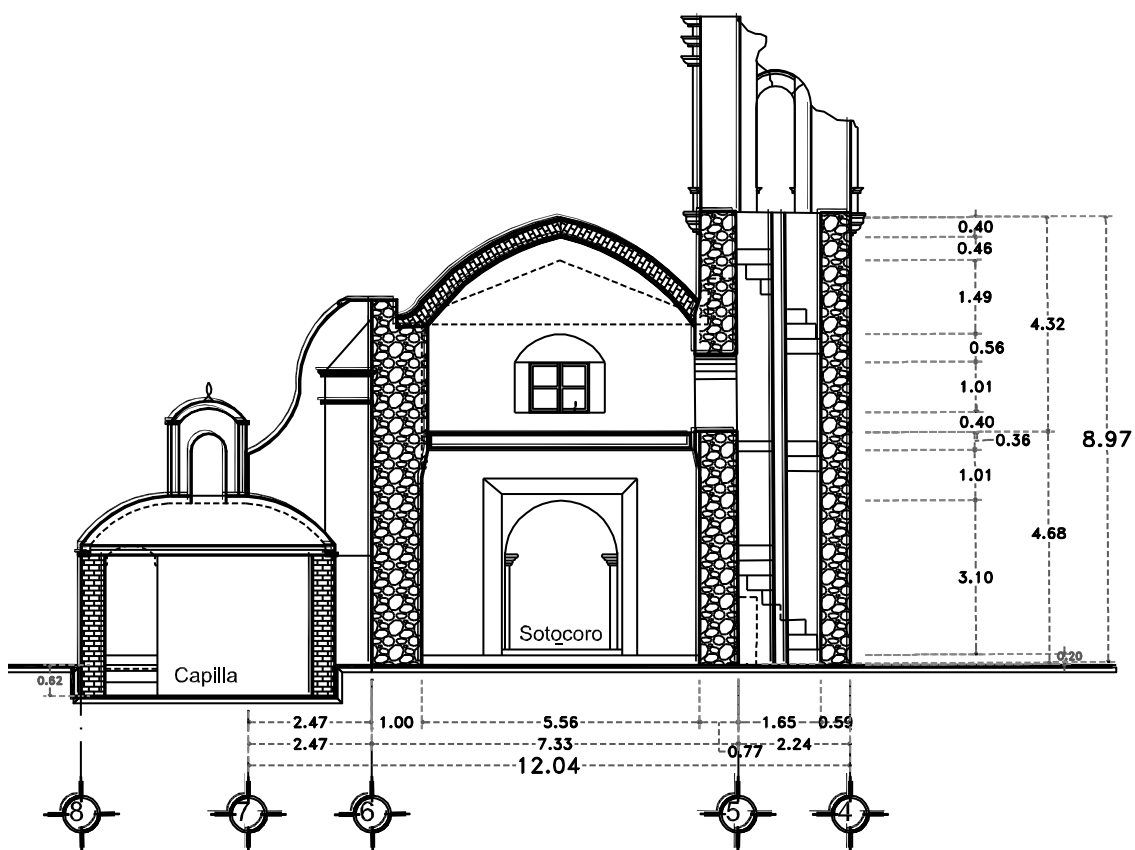
Figura 3.16. Corte transversal X-X' de la iglesia de Pilcaya
