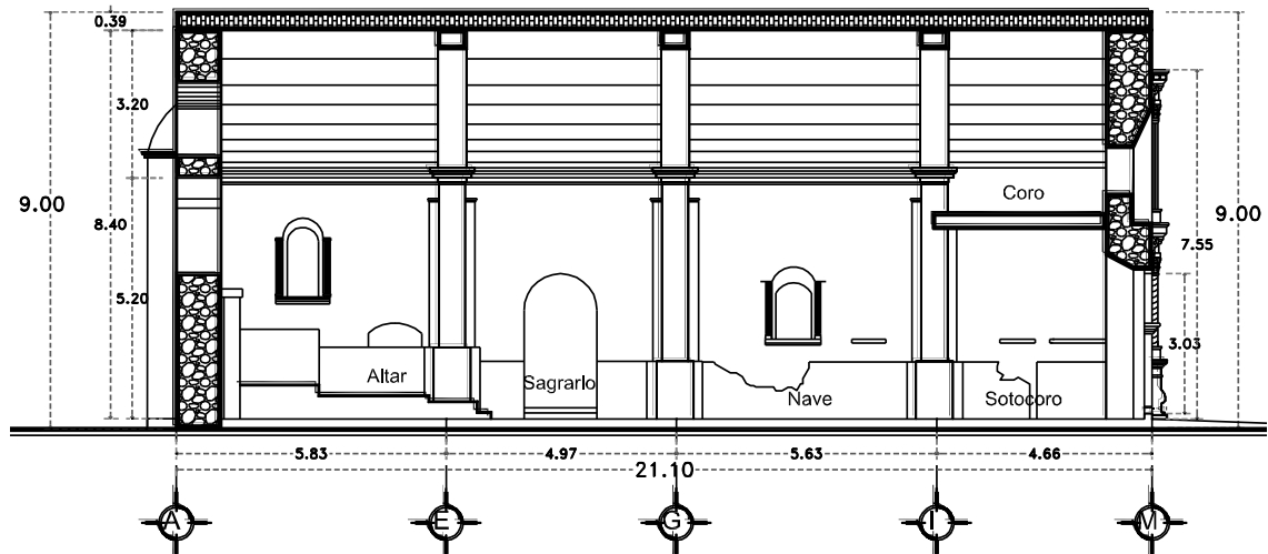
Figura 3.13. Corte longitudinal Y-Y' de la iglesia de Pilcaya
