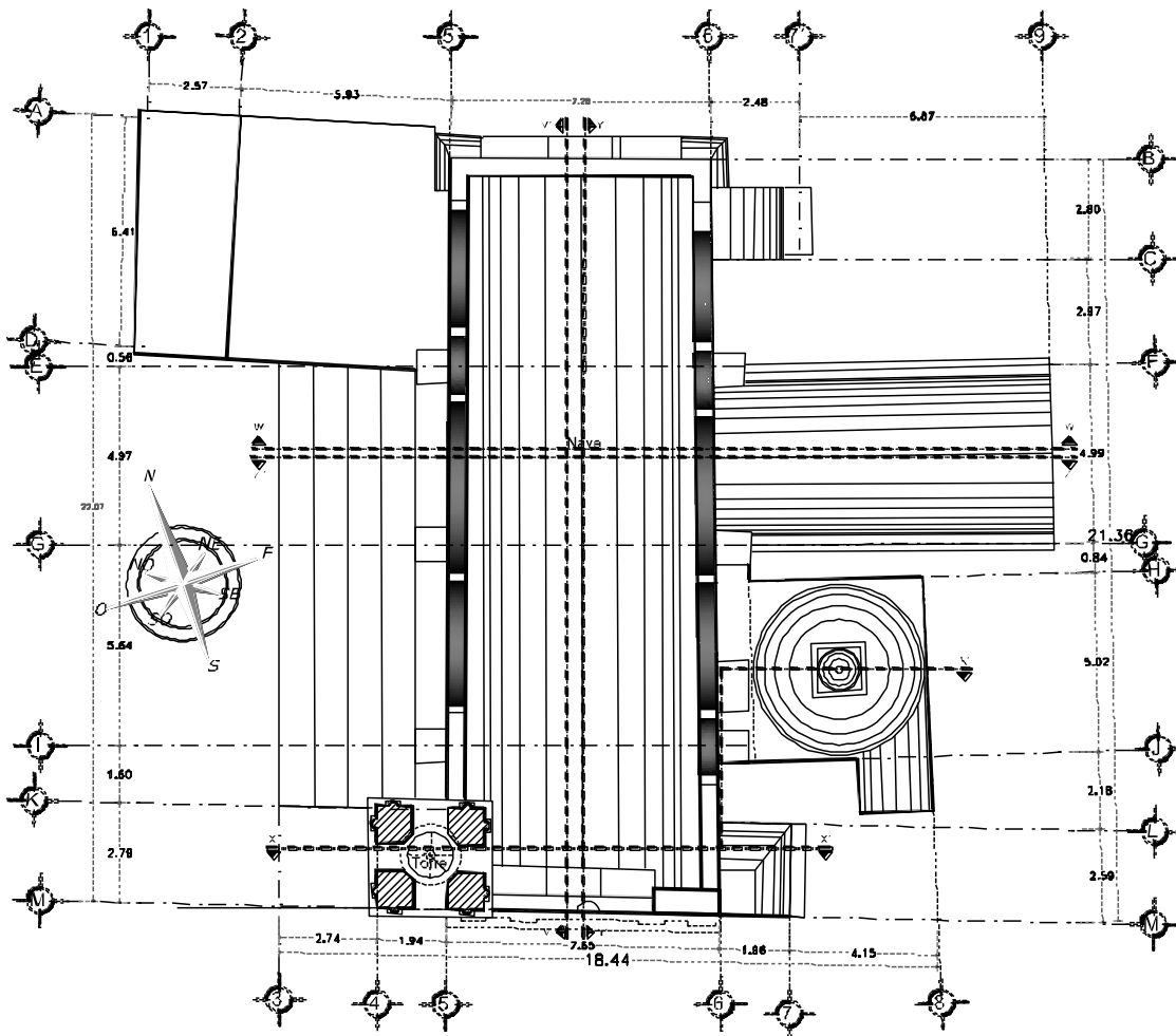
Figura 3.7. Planta de la iglesia de Pilcaya, Puebla (N.P.T. +9.30 m).
