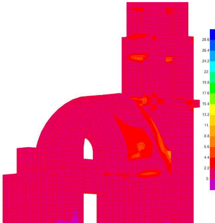
Figura 4.20. Concentración de esfuerzos axiales longitudinales (S22, en kg/cm 2 )
