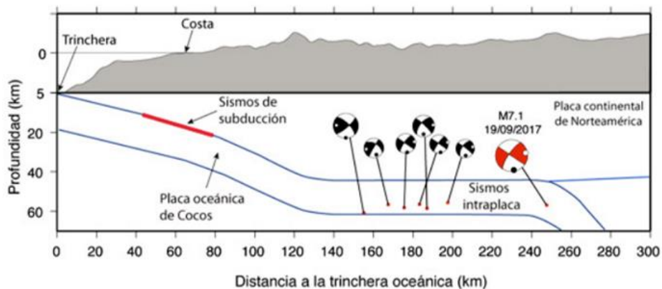
Figura 1.1. Localizaciones del sismo de magnitud 7.1 del 19 de septiembre de 2017 y algunos otros del mismo tipo en la región (Cruz-Atienza et al., 2017)
