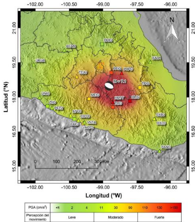
Figura 1.2. Mapa de intensidades instrumentales para el sismo de Puebla-Morelos (Valencia, 2019)
