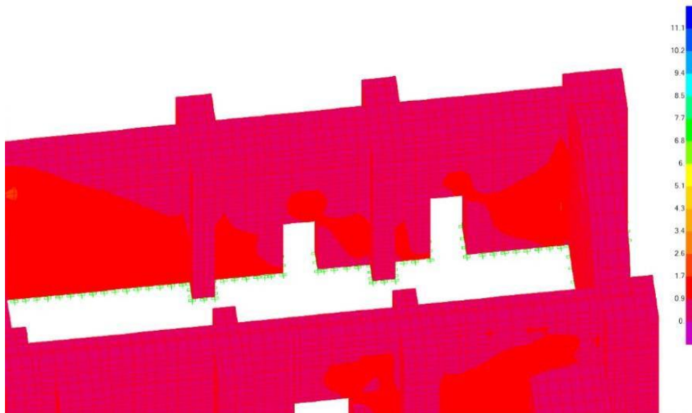
Figura 4.21. Esfuerzos cortantes S23 en los muros de las fachadas Oriente y Poniente (en la cara perpendicular al eje longitudinal con dirección vertical, en kg/cm 2 )
