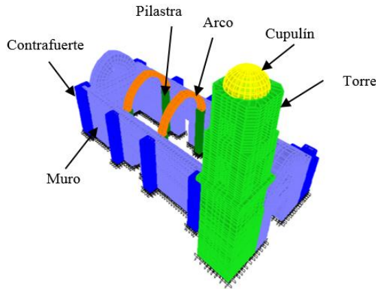
Figura 4.3. Nombres de los elementos del modelo numérico en vista tridimensional
