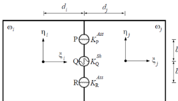
Figura 2.9. Conexión de dos elementos rígidos (Orduña, Roeder y Peña, 2007)
