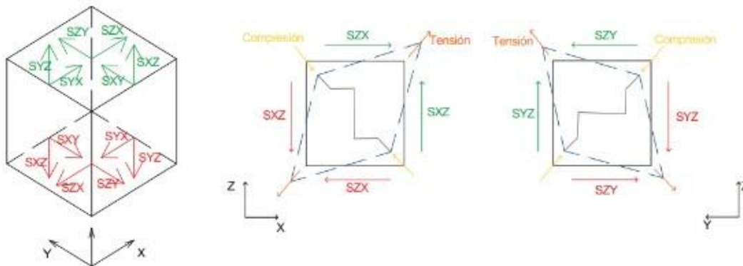
Figura 4.16. Esfuerzos cortantes en los sólidos (Quiroz, 2017)
