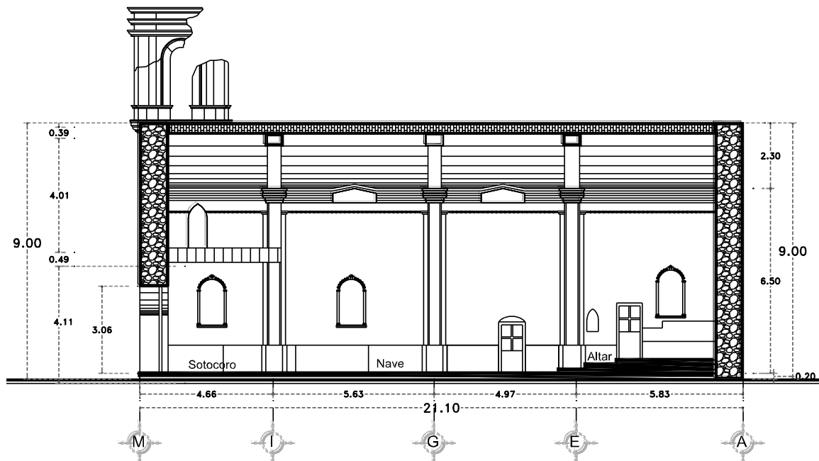
Figura 3.14. Corte longitudinal V-V' de la iglesia de Pilcaya
