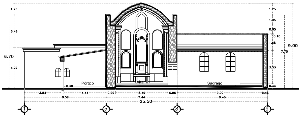
Figura 3.15. Corte transversal W-W' de la iglesia de Pilcaya
