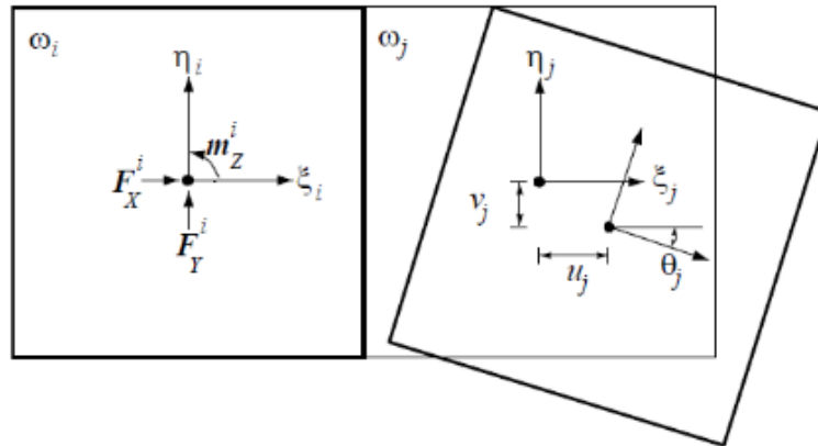
Figura 2.8. Fuerzas y desplazamientos de los elementos rígidos (Orduña, Roeder y Peña, 2007)
