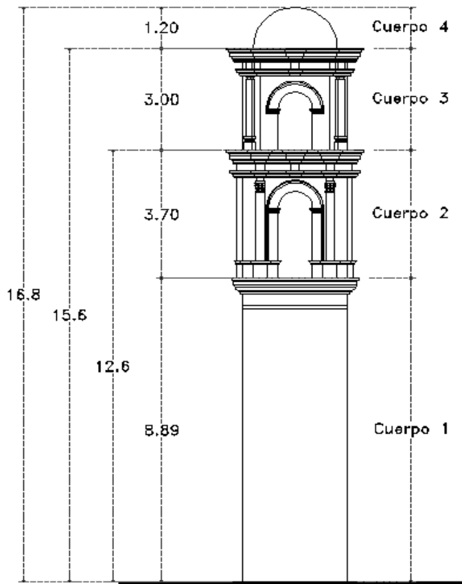
Figura 4.22. Torre con referencias para la revisión de sus distorsiones
