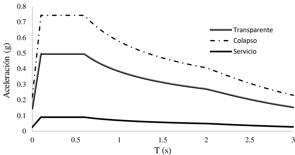
Figura 4.13. Espectros horizontales: transparente, de colapso y servicio
