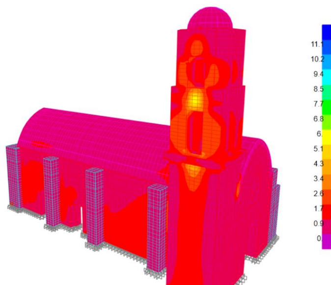
Figura 4.18. Esfuerzos cortantes S_{23} en cerramientos en las caras Poniente y Oriente de la torre (en \text{kg/cm}^2 )
