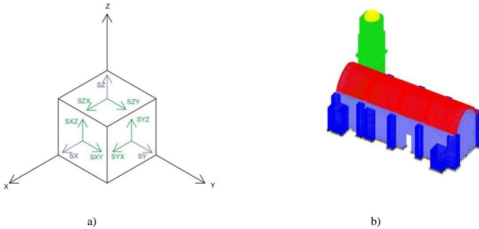
Figura 4.15. Ejes ortogonales en el modelo: a) Esfuerzos axiales en un sólido (Quiroz, 2017), b) Modelo numérico de la iglesia
