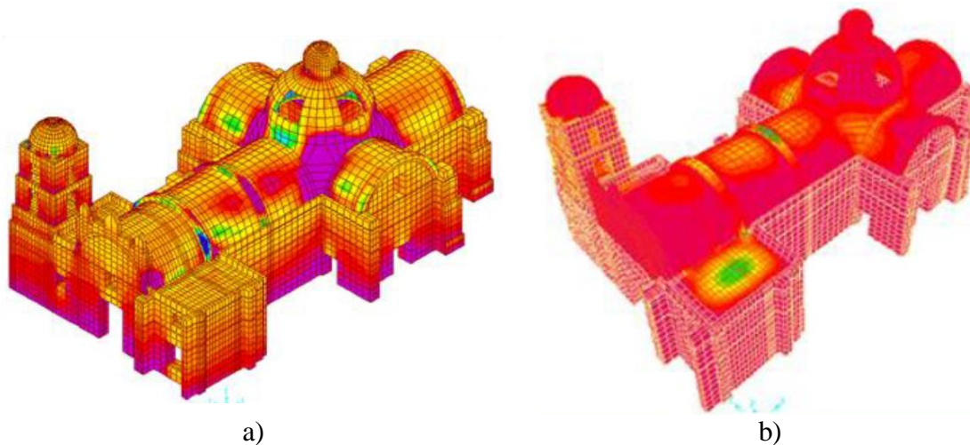
Figura 2.11. Esfuerzos en el modelo numérico: a) axiales por peso propio, b) cortantes transversales con sismo 100% en dirección longitudinal y 30% en dirección transversal (Robles, 2013)
