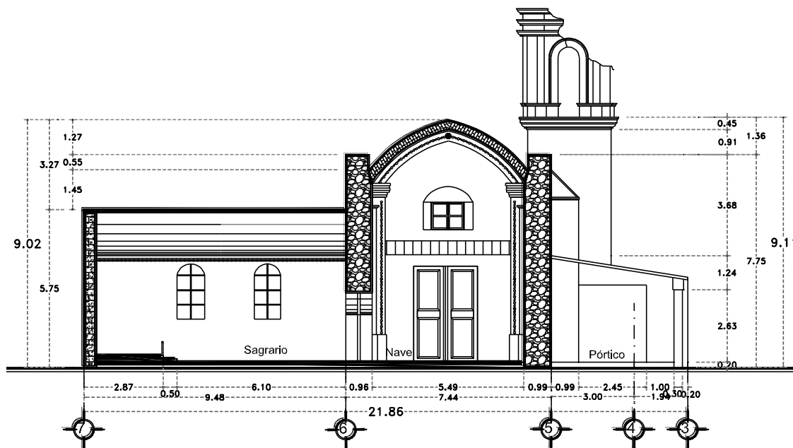
Figura 3.17. Corte transversal Z-Z' de la iglesia de Pilcaya
