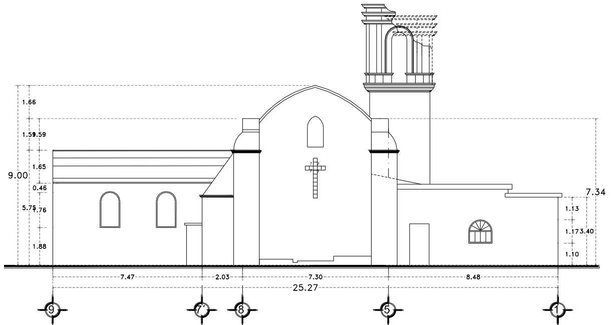
Figura 3.11. Fachada Norte de la iglesia de Pilcaya, Puebla
