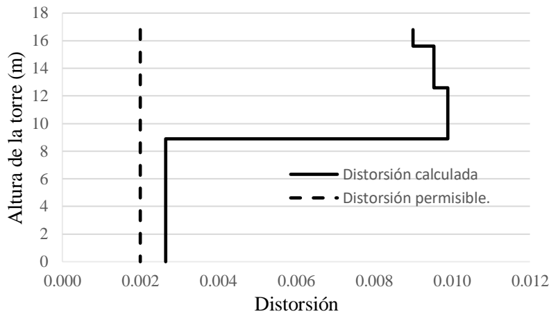
Figura 4.26. Comparación de las distorsiones calculadas y las permitidas para estado límite de colapso en dirección longitudinal
