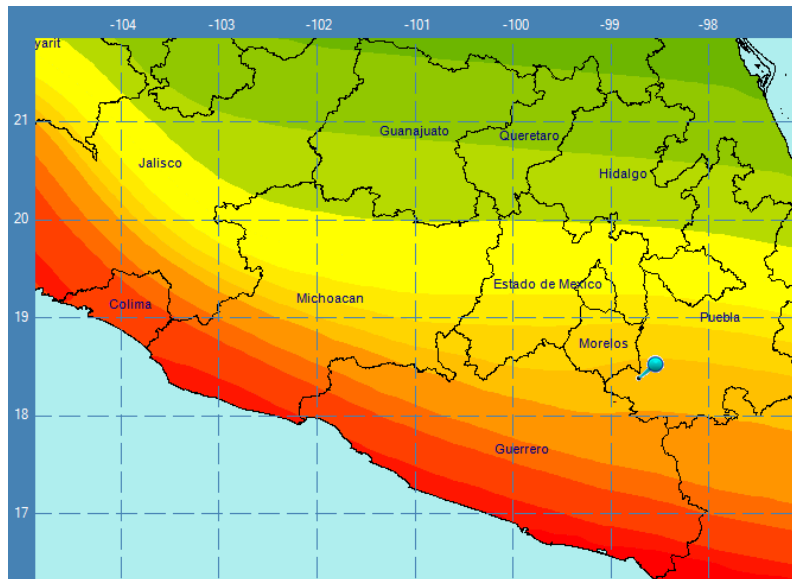
Figura 1.4. Epicentro del sismo del 19 de septiembre de 2017 (Imagen extraída del programa PRODISIS)
