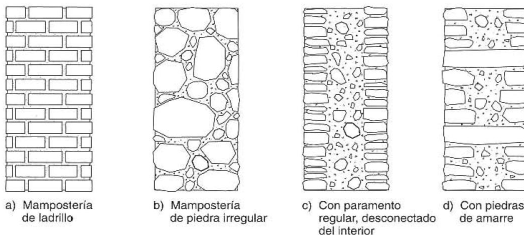
Figura 2.3. Algunas modalidades de mampostería (Meli, 1998)
