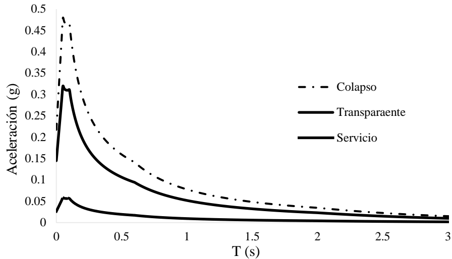
Figura 4.14. Espectros verticales: transparente, de colapso y servicio.
