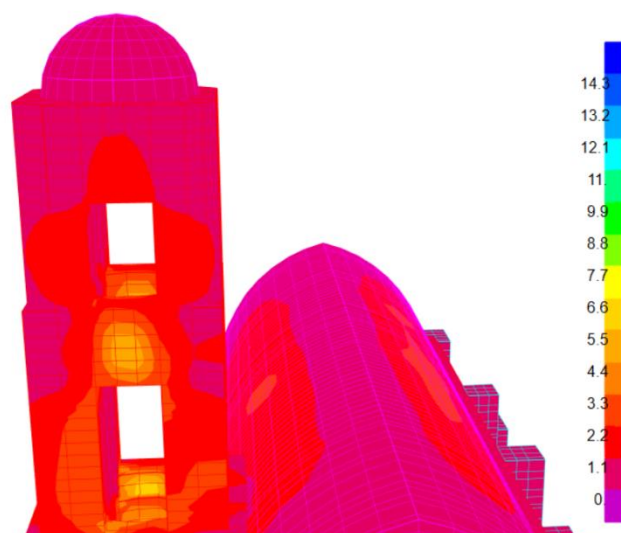
Figura 4.19. Esfuerzos cortantes en los cerramientos de las caras frontal y trasera de la Torre (en \text{kg/cm}^2 )
