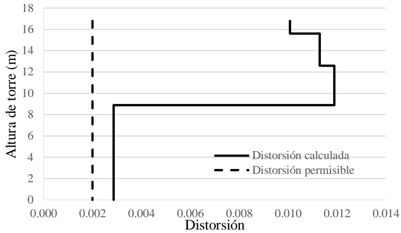
Figura 4.25. Comparación de las distorsiones calculadas y las permitidas para estado límite de colapso en dirección transversal
